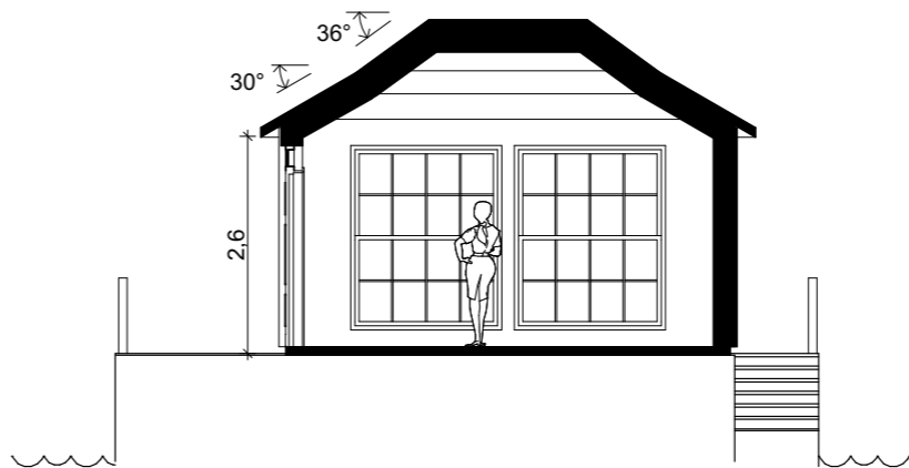
SEKTION A-A
