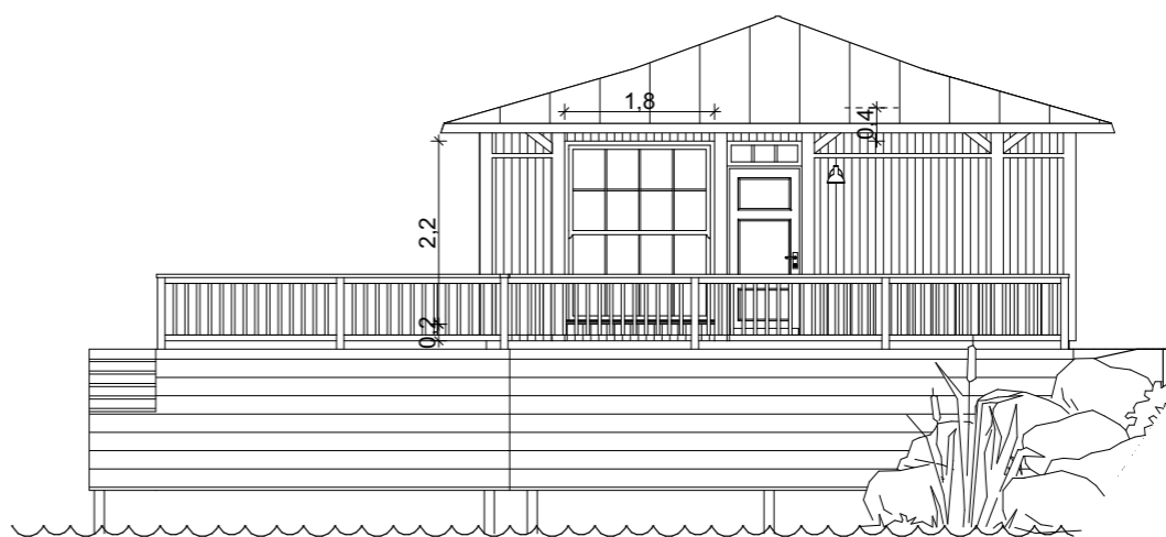
FASAD A4 - MOT SYDVÄST
