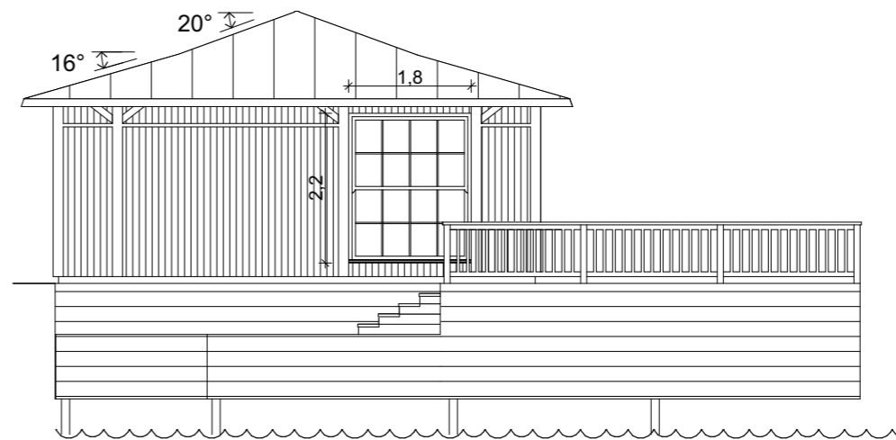
FASAD A2 - MOT NORDOST
