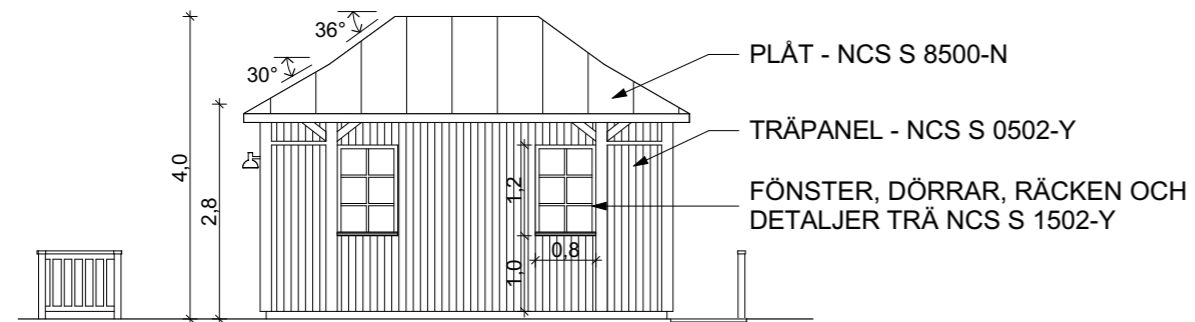
FASAD A1 - MOT SYDOST
