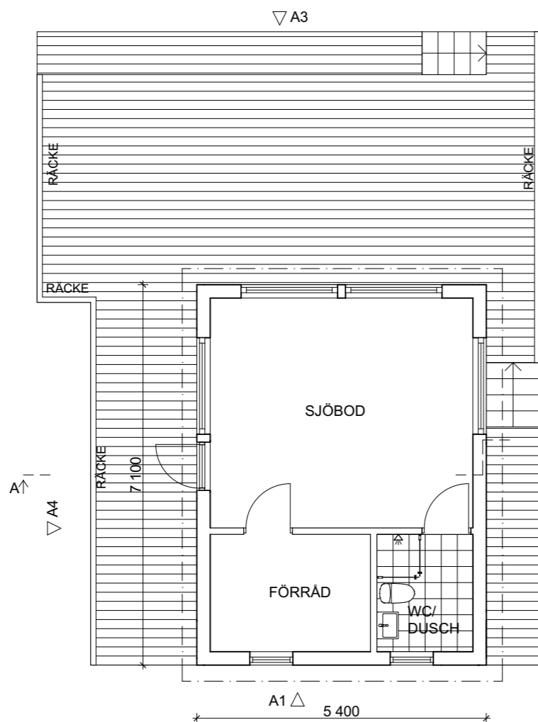
ENTRÉPLAN
