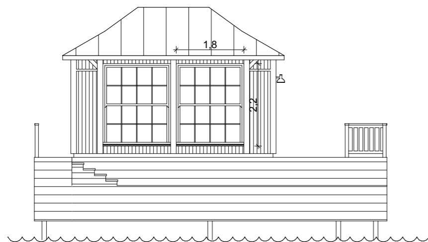
FASAD A3 - MOT NORDVÄST
