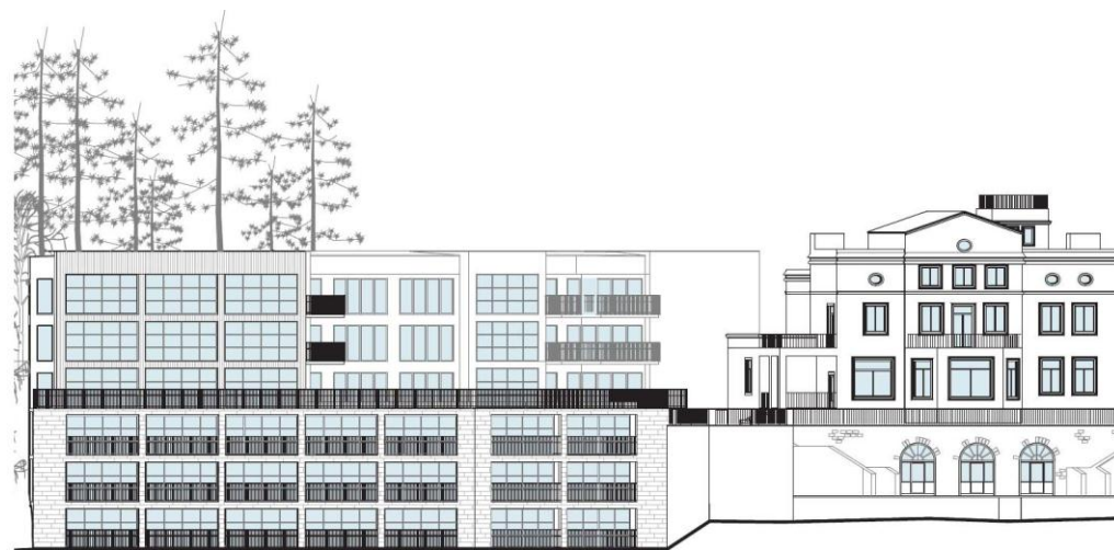
Huvudbyggnadens och vårdboendets fasad mot söder (Baggensfjärden).
