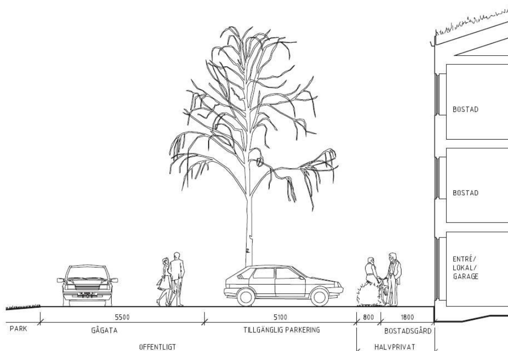
Principsektion genom gångfartsgata-tvårvälld parkering och förgårdsmark till bostadshus.
