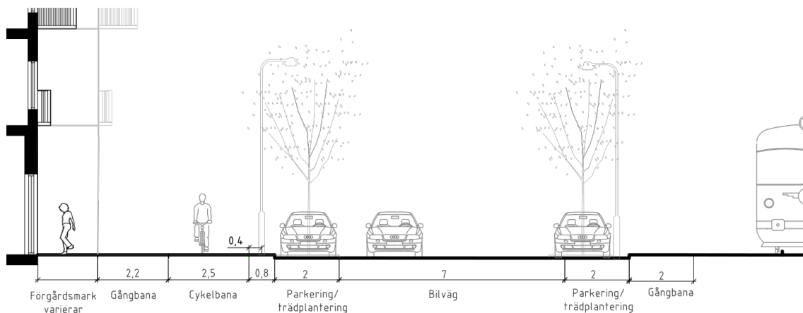
Fisksättravägens föreslagna sektion. Måtten som anges är i meter. (Bild: Mandaworks)
