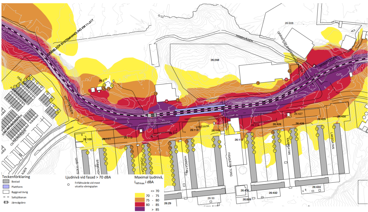
Nytt stationsläge, trafikflöde 2030. Maximal ljudnivå från spårtrafik 1,5 meter över mark och vid fasad. Se illustrationen i sin helhet i ritning A04 Bullerutredning – Järnvägsplan, Fisksätra station Nacka, Akustikkonsulten, 2020-01-27.
