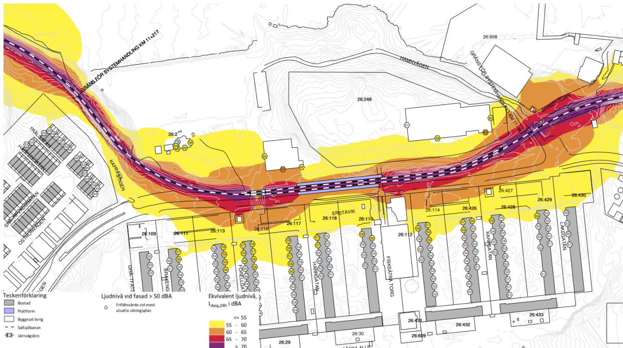
Nytt stationsläge, trafikflöde 2030. Ekvivalent ljudnivå från spårtrafik 1,5 meter över mark och vid fasad. Se illustrationen i sin helhet i ritning A03 Bullerutredning – Järnvägsplan, Fisksätra station Nacka, Akustikkonsulten, 2020-01-27.
