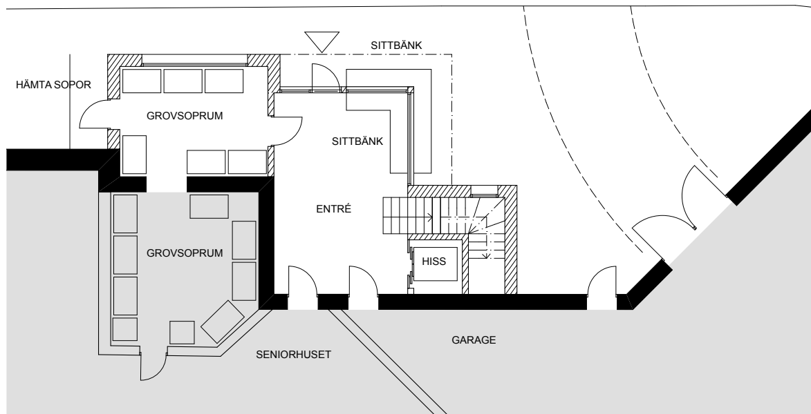
Förslag entréplan.
