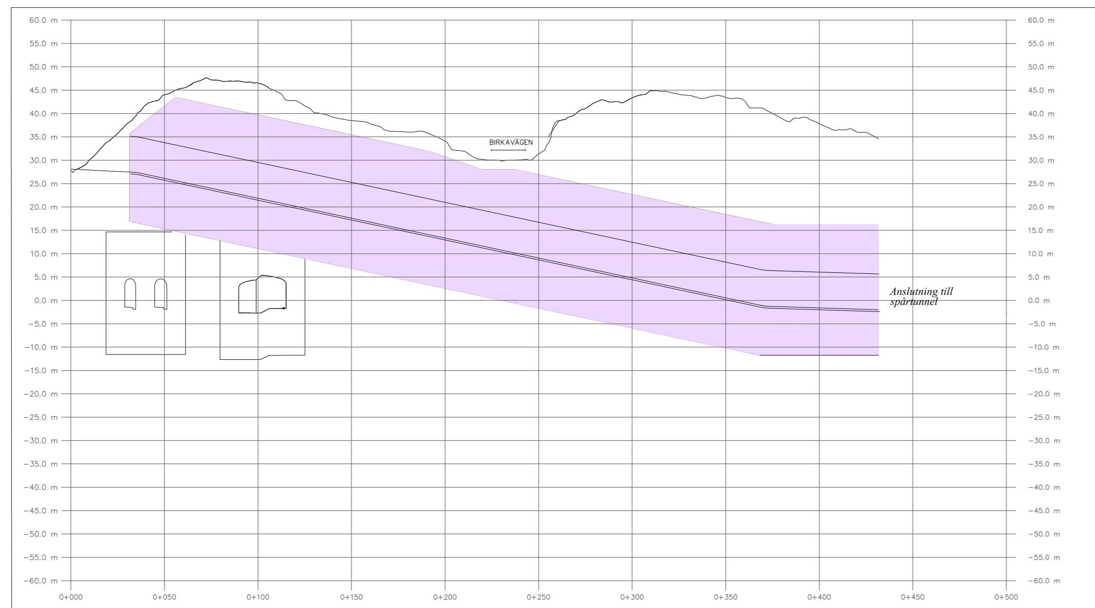
Järfa Profil, arbetstunnel (i driftskedet utrymningsväg och ventilationstunnel)
