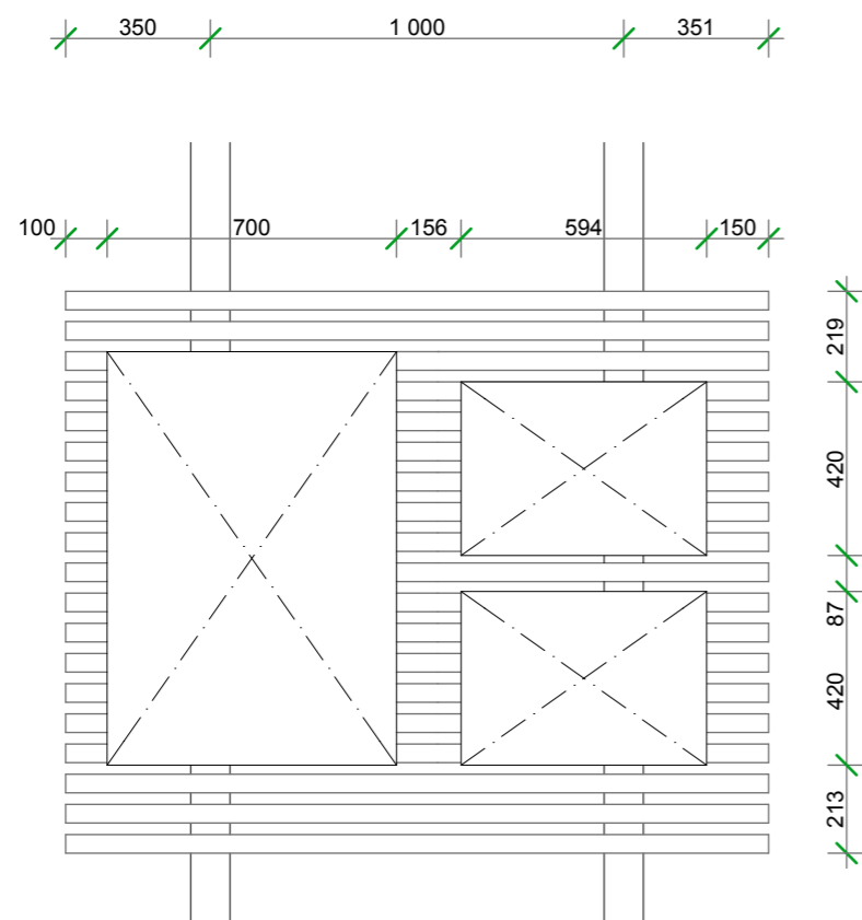
ELEVATIONER
