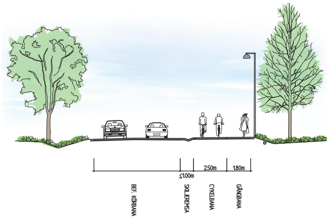
Bild 26. GC-väg med skiljeremsa 1m eller smalare som utförs med hårdgjord yta.
