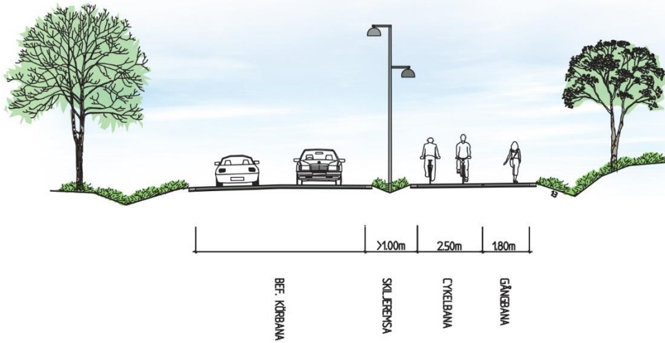
Bild 27. GC-väg med grön skiljeremsa.
