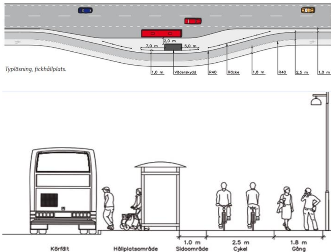
Bild 31. Princip för utformning vid busshållplatser (Källa: regional cykelplan för Stockholms län).
