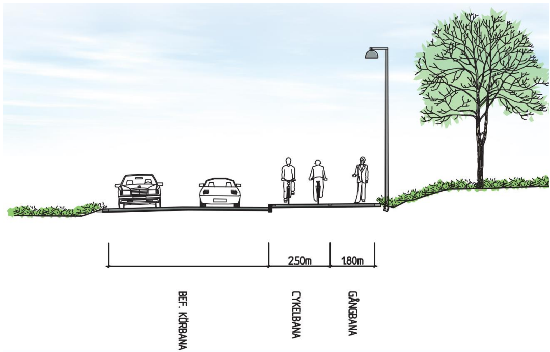
Bild 25. Kantstensförlagd GC-väg utan skiljeremsa.
