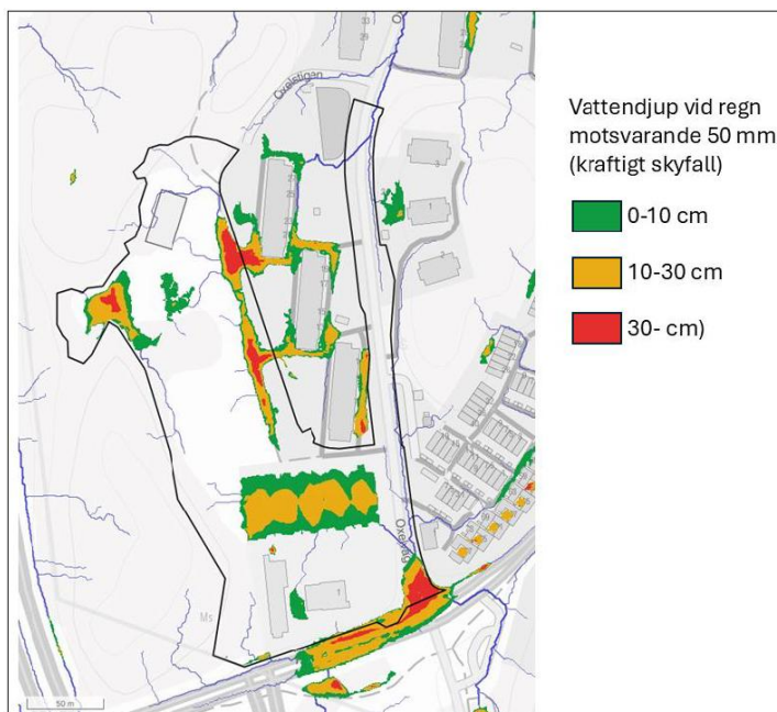
Figur 50: Översvåmningsanalys av befintlig situation ifrån dagvattenutredningen (Marktema 2024). Planområdesgränsen har uppdaterats till antagandet, och den norra delen ingår inte längre i planen.
