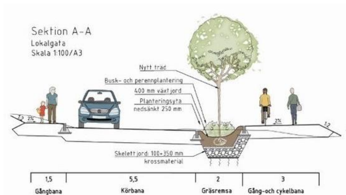
Figur 35: Utformning som visar sektion för den föreslagna lokalgatan. Bilden är inte skalenlig. (Bjerking 2023)
