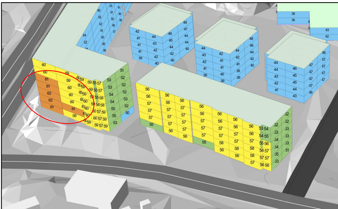
Figur 42: Fasad utmed Oxelvägen med ekvivalent ljudnivå över 60 dBA. Ältavägen ses i mörkgrått till vänster i bild och Oxelvägen syns nederst i bild. (Akustikkonsulten 2024)
