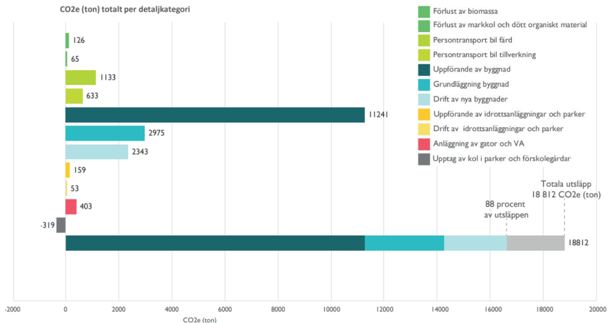
Figur 51: Koldioxidekvivalenter, CO 2 e, uttryckt i ton, per detaljkategori, och totalt. I den samlade stapeln i botten är de blå delarna relaterade till byggnaderna, och den grå delen visar övriga detaljkategorier samlat (Nacka kommun 2024).
