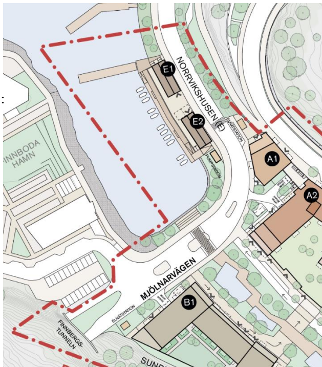
Byggnaderna E1 och E2 motsvarar föreslagna sjöbodarna. Röd linje motsvarar föreslagna plangräns.
