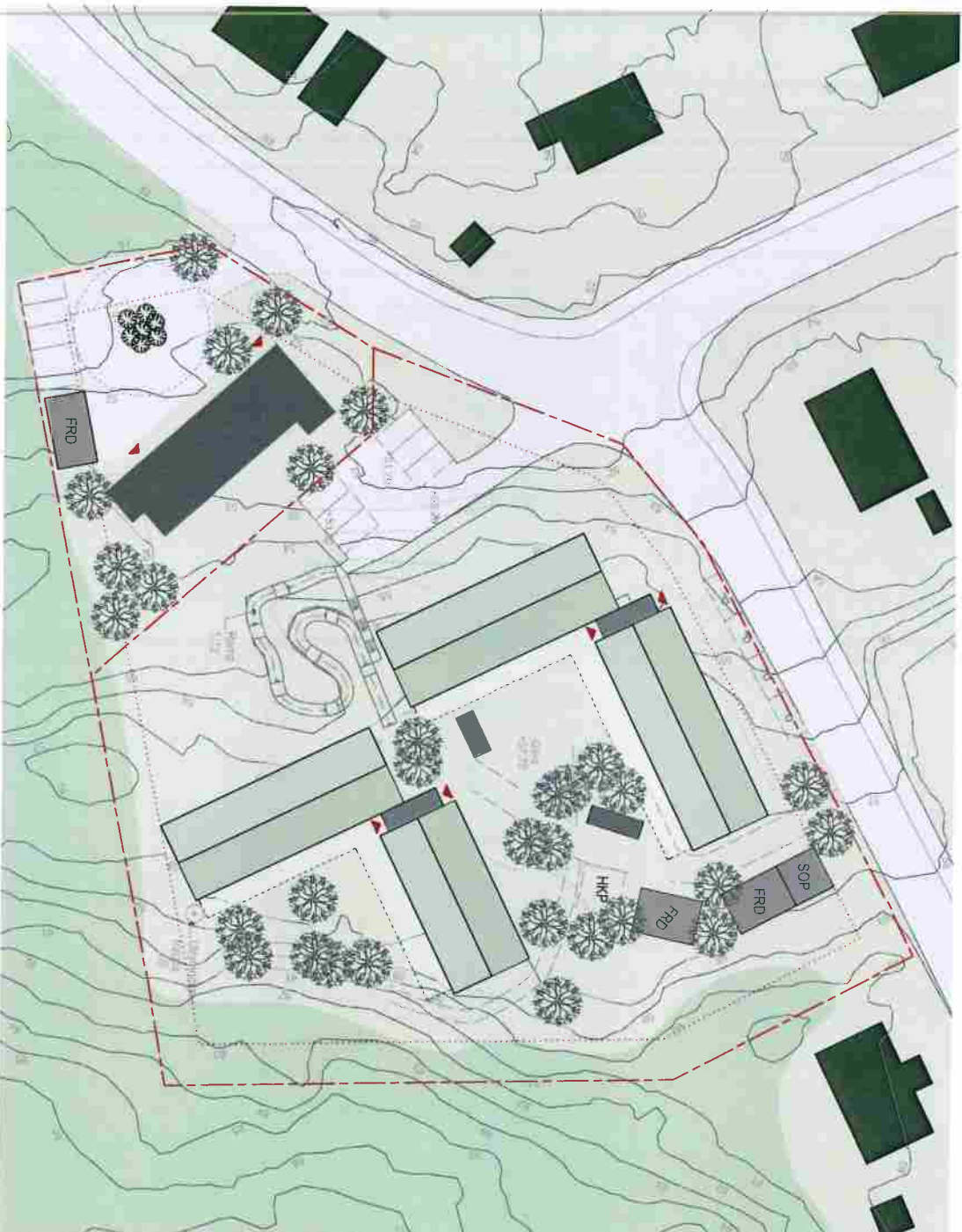
Alternativ med backvändning för transporter till LSS-boende Skala 1:500
