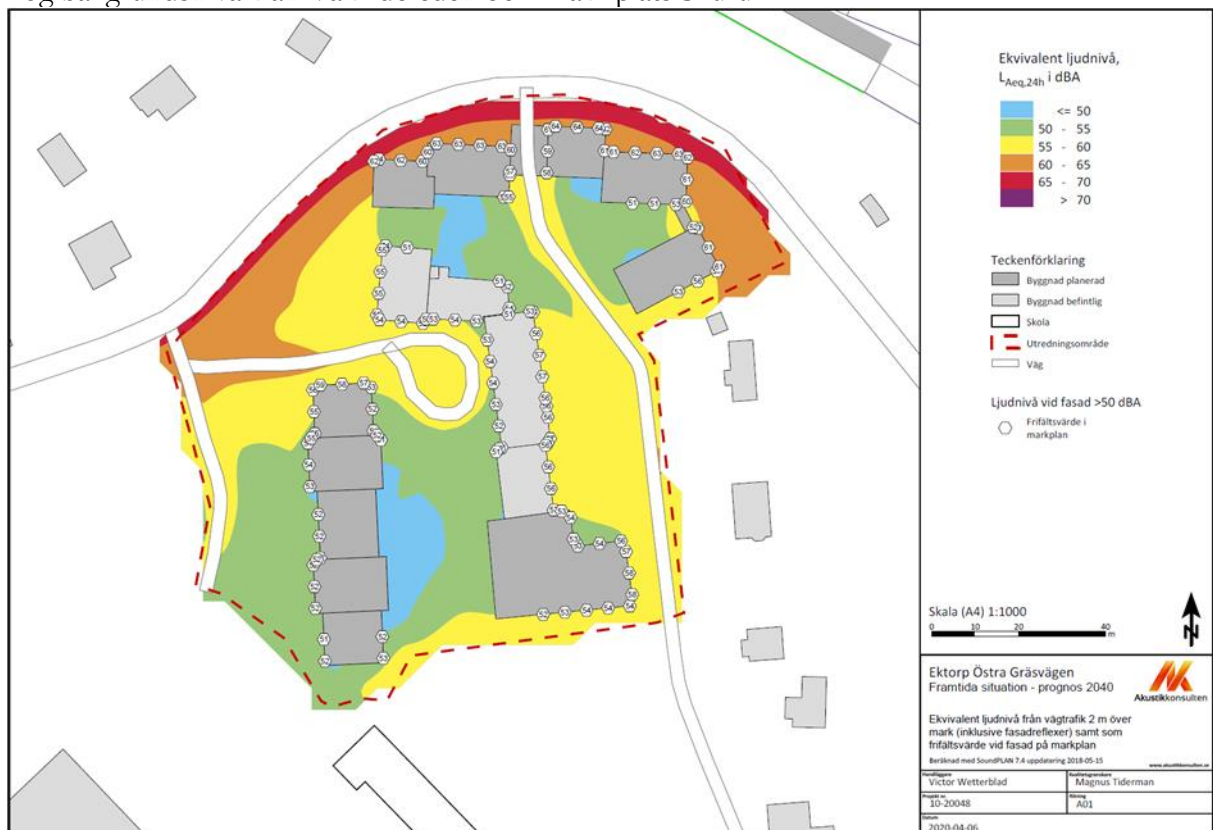
Figur 9. Beräknad ekvivalent ljudnivå från vägtrafik 2 m över mark för hela planområdet.
