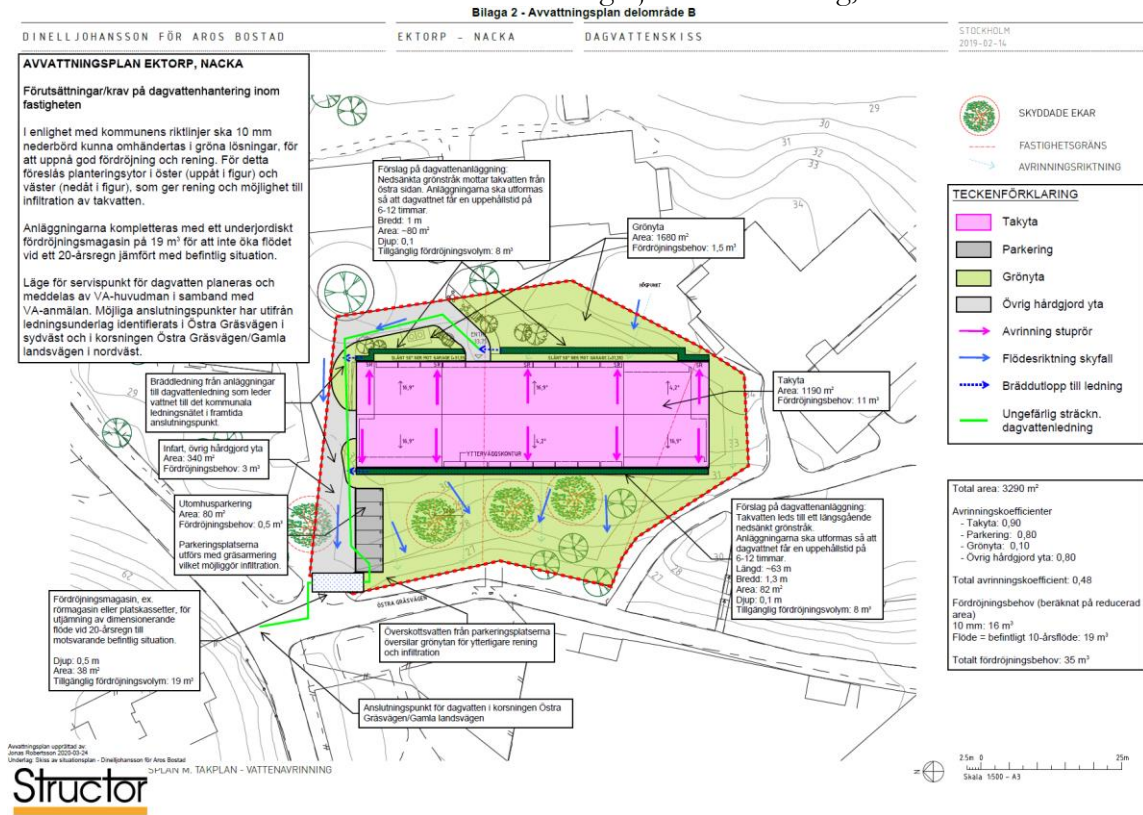
Figur 6. Översiktlig avvattningsplan som visar föreslagna dagvattenhantering inom Delområde B.
