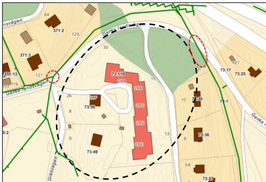
Figur 4. Figuren visa ledningsnät och föreslagna anslutningspunkter.
