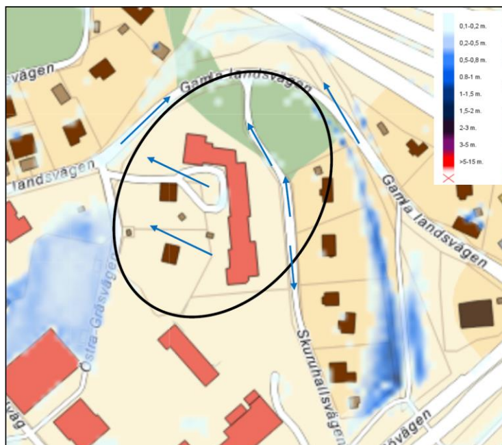
Figur 20. Utdrag från Nacka kommuns skyfallsanalys, 100-årsregn med klimatkfaktor 1.2. Detaljplaneområdets ungefärliga lokalisering är markerad med en svart ellips. Pilar illustrerar vattnets ungefärliga flödesriktningar i terrängen vid ett skyfall. En mindre yta i sydöst avrinner åt söder, i övrigt sker avrinningen vid skyfall mot norr.
