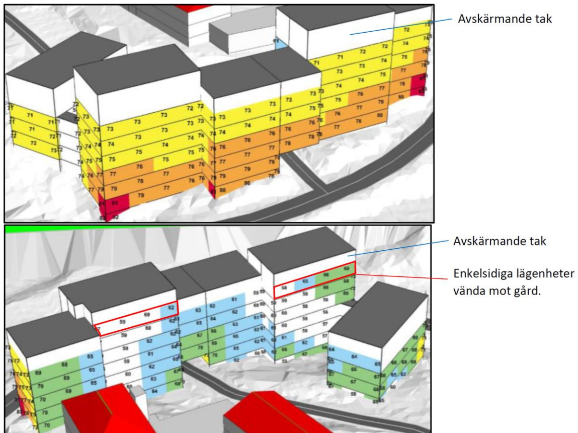
Figur 11. Beräknad maximal ljudnivå vid fasad anseende vägtrafik nattetid.
