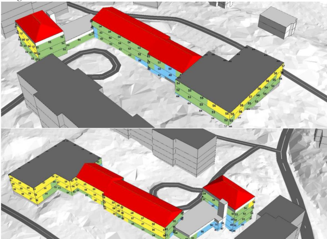
Figur 13. Beräknad ekvivalent ljudnivå vid fasad anseende vägtrafik.
