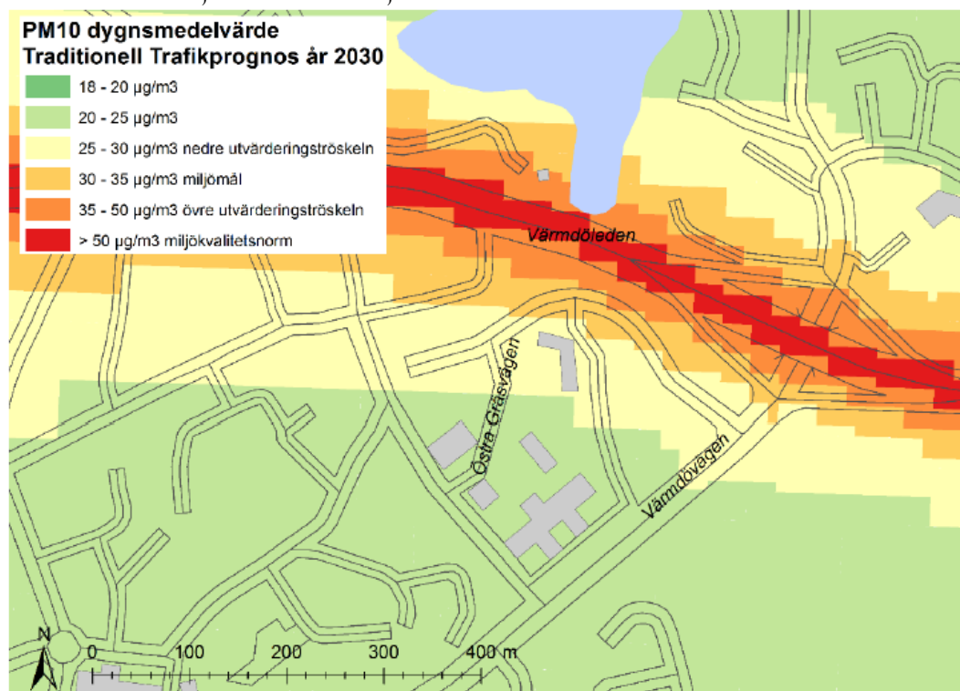
Figur 18. Beräknad dygnsmedelhalt år 2030 av partiklar, PM10 ( \mu\text{g}/\text{m}^3 ), under det 36:e värsta dygnet. Trafikprognos traditionell. Normvärdet som ska klaras är 50 \mu\text{g}/\text{m}^3 och miljömålet 30 \mu\text{g}/\text{m}^3 .
