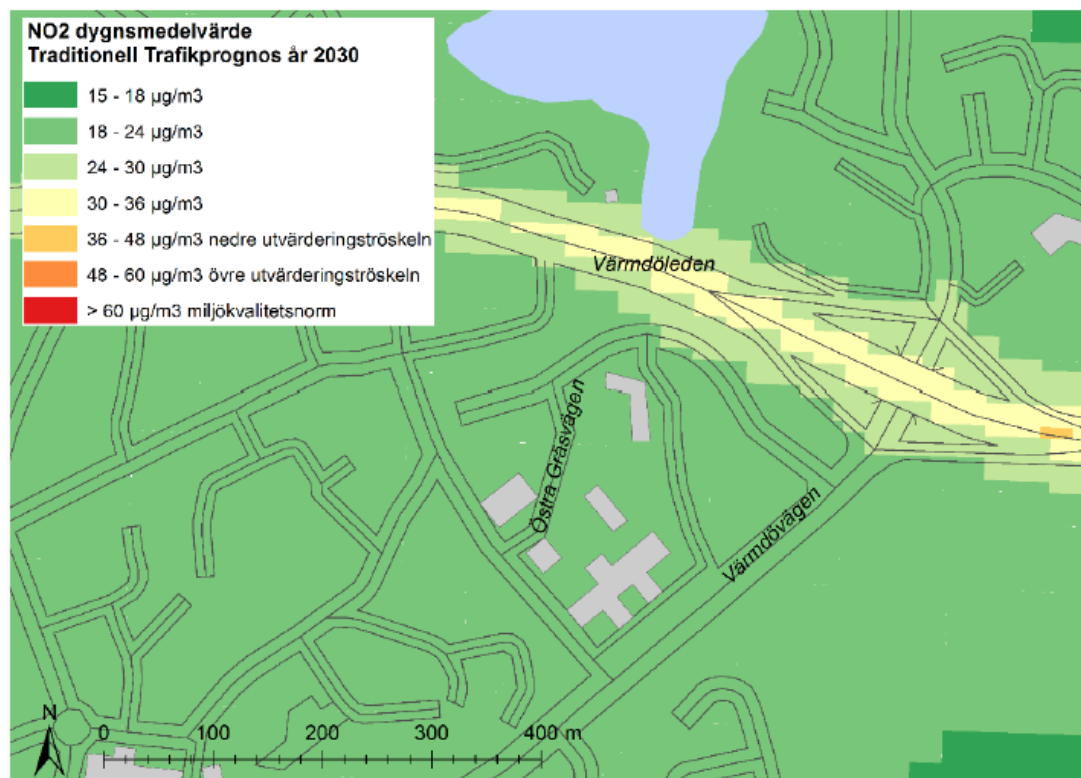
Figur 19. Beräknad dygnsmedelhalt år 2030 av kväveoxid, NO 2 ( \mu\text{g}/\text{m}^3 ), under det 8:e värsta dygnet. Trafikprognos traditionell. Normvärdet som ska klaras är 60 \mu\text{g}/\text{m}^3 . Miljömål saknas.
