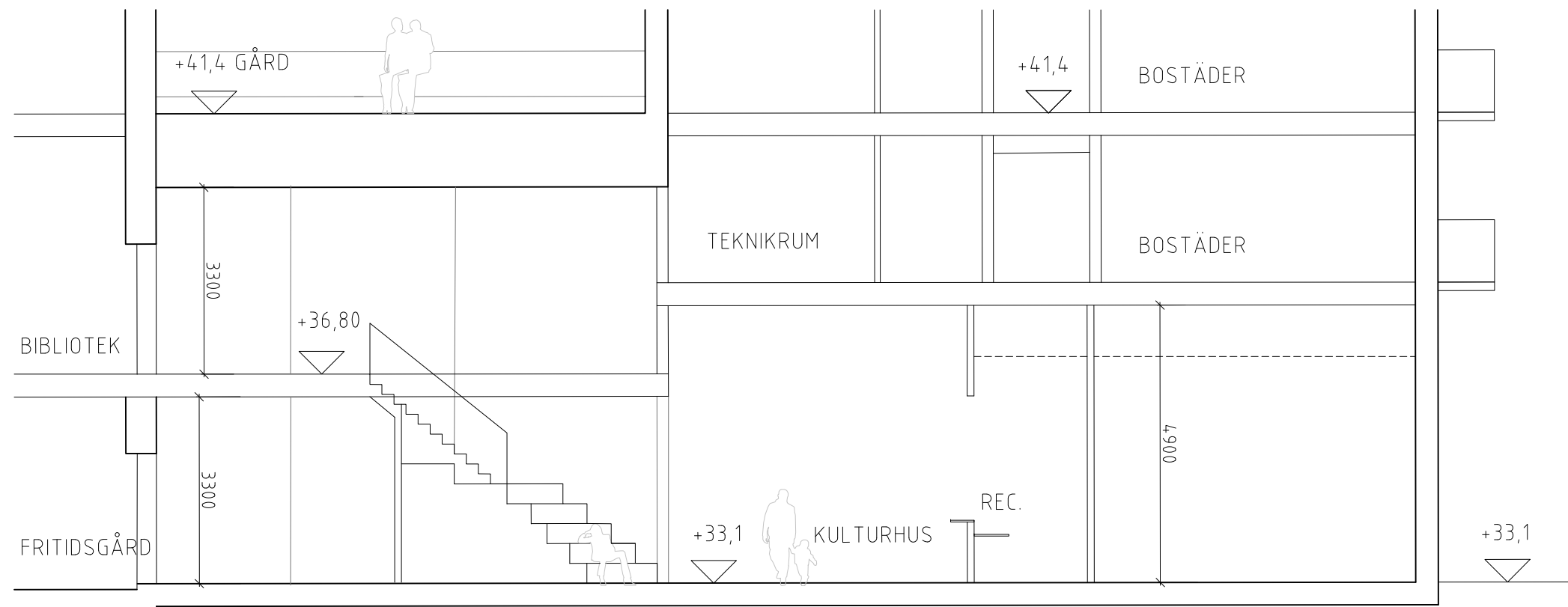
SNITT - TAGEN UR SEKTION D - ALT 2
