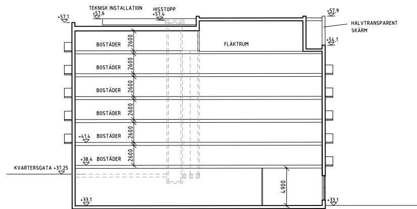
SEKTION A ALT 2
