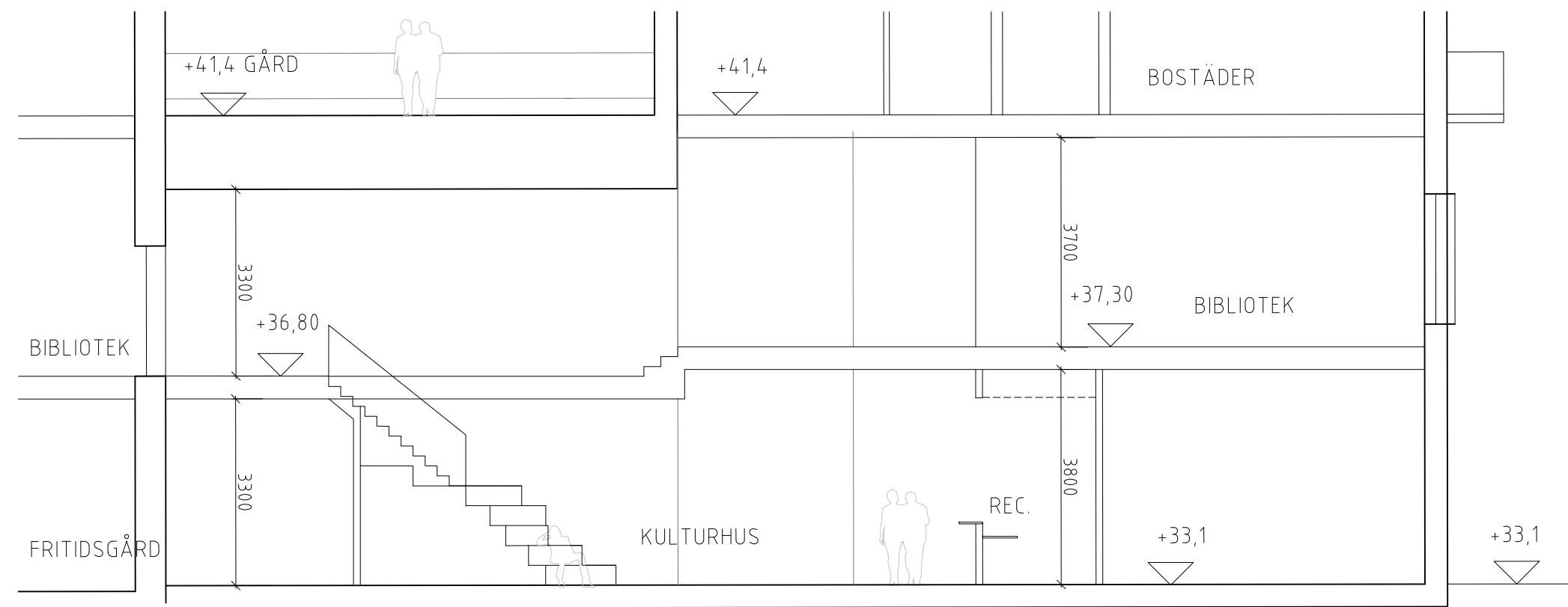
SNITT - TAGEN UR SEKTION D - ALT 3
