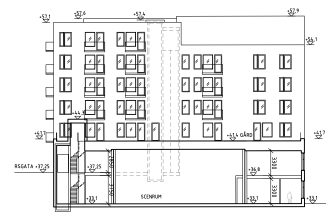
SEKTION B ALT 2 OCH ALT 3
