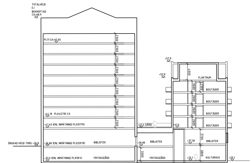
SEKTION D, PRINCIP ALT 3 ALT 3
