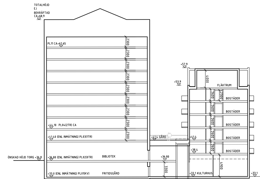
SEKTION D, PRINCIP ALT 2 ALT 2
