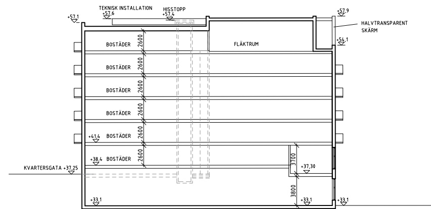
SEKTION A ALT 3
