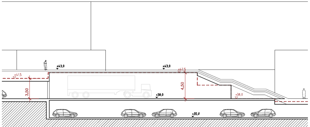
Principsektion B-B, trappa mellan Kanholmsvägen och Röda torget.
