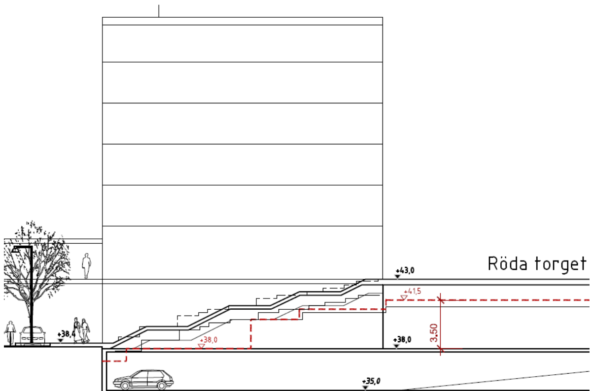
Principsektion A-A, trappa mellan Edövägen och Röda torget.
