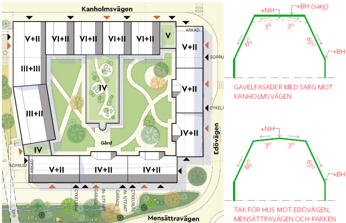
Till vänster: Illustrationsplan exempelutförning, Brunnberg & Forsbed - kvarter Hantverksbuset, norr åt höger (utförning av allmän platsmark ej i enlighet med planförslaget). Till höger: principer taksfall kvarter Hantverksbuset
