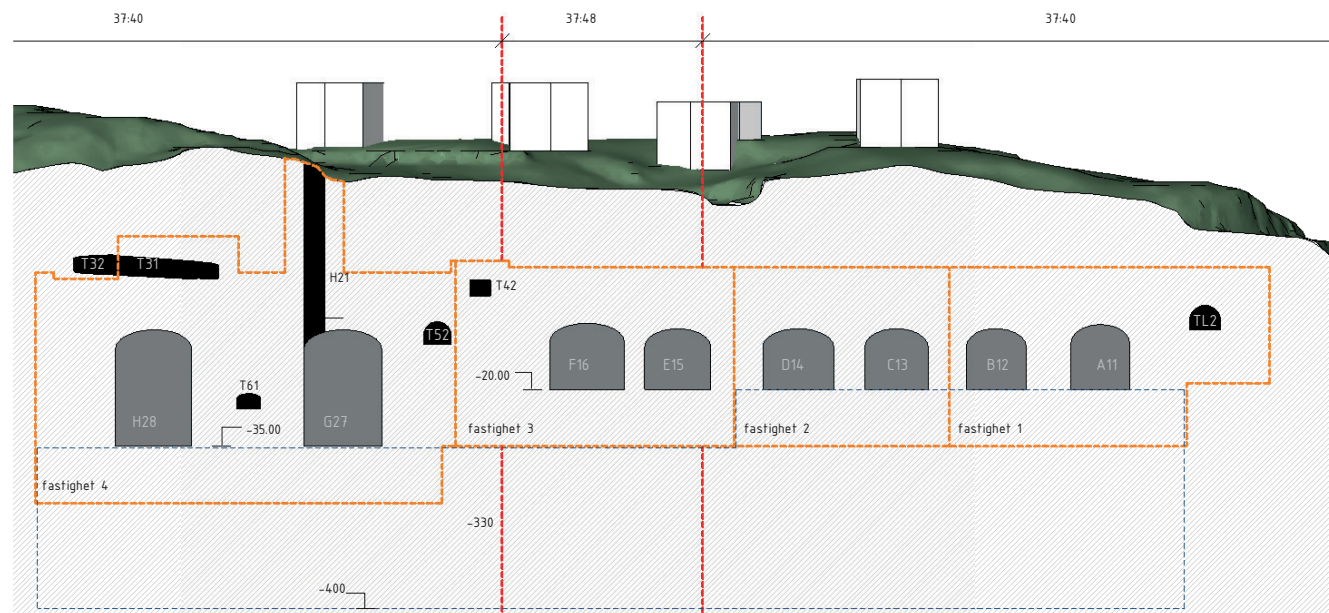
2 Sektion BB 1 : 1000
