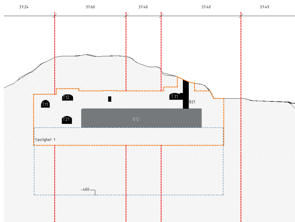
1 Sektion DD 1 : 1000
