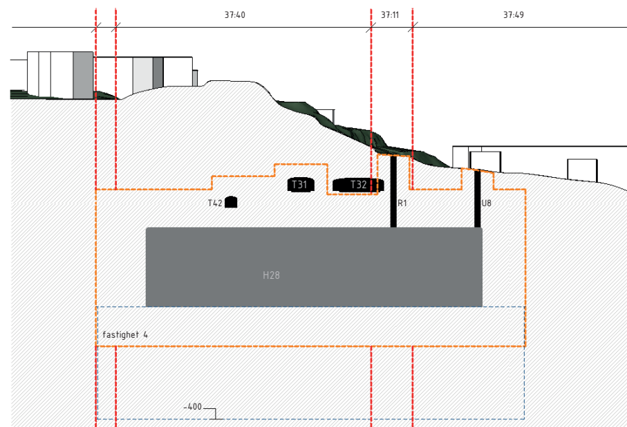
4 Sektion GG 1 : 1000
