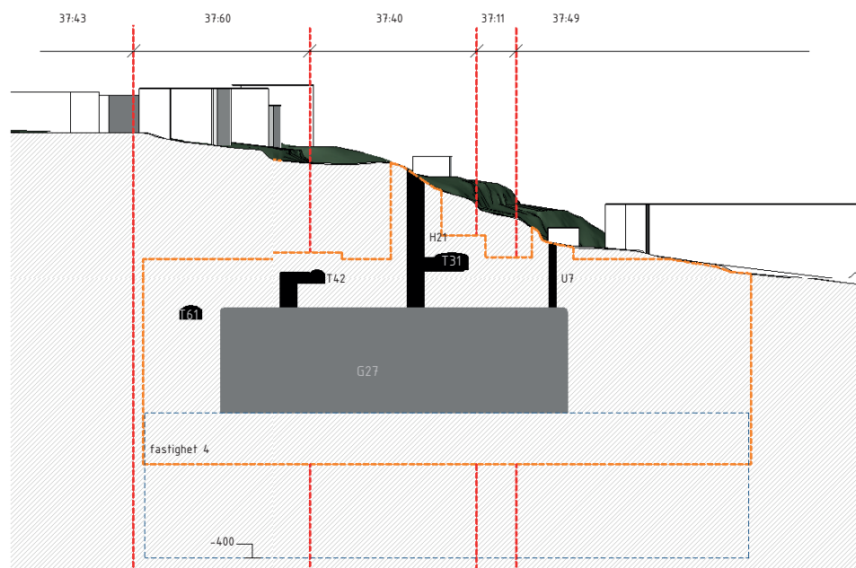
2 Sektion EE 1 : 1000
