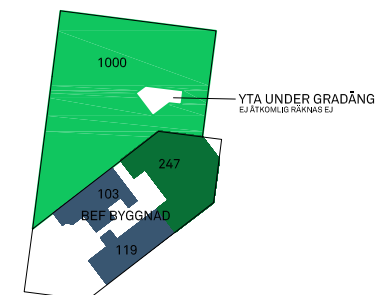
PLAN -1 (09) NY BTA LOKAL 1000kvm BEF BTA LOKAL 247kvm BEF BTA TEKNIK 222kvm
