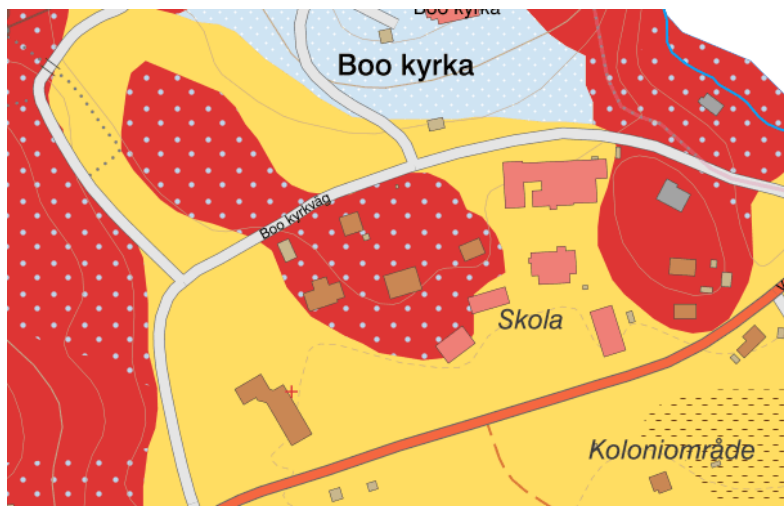
Figur 9: Övergripande jordartskartering. Rött utgörs av berg, gult utgör postglacial lera och ljusblå prickar utgör tunt moränlager. Bildkälla: SGUs jordartskartering.
