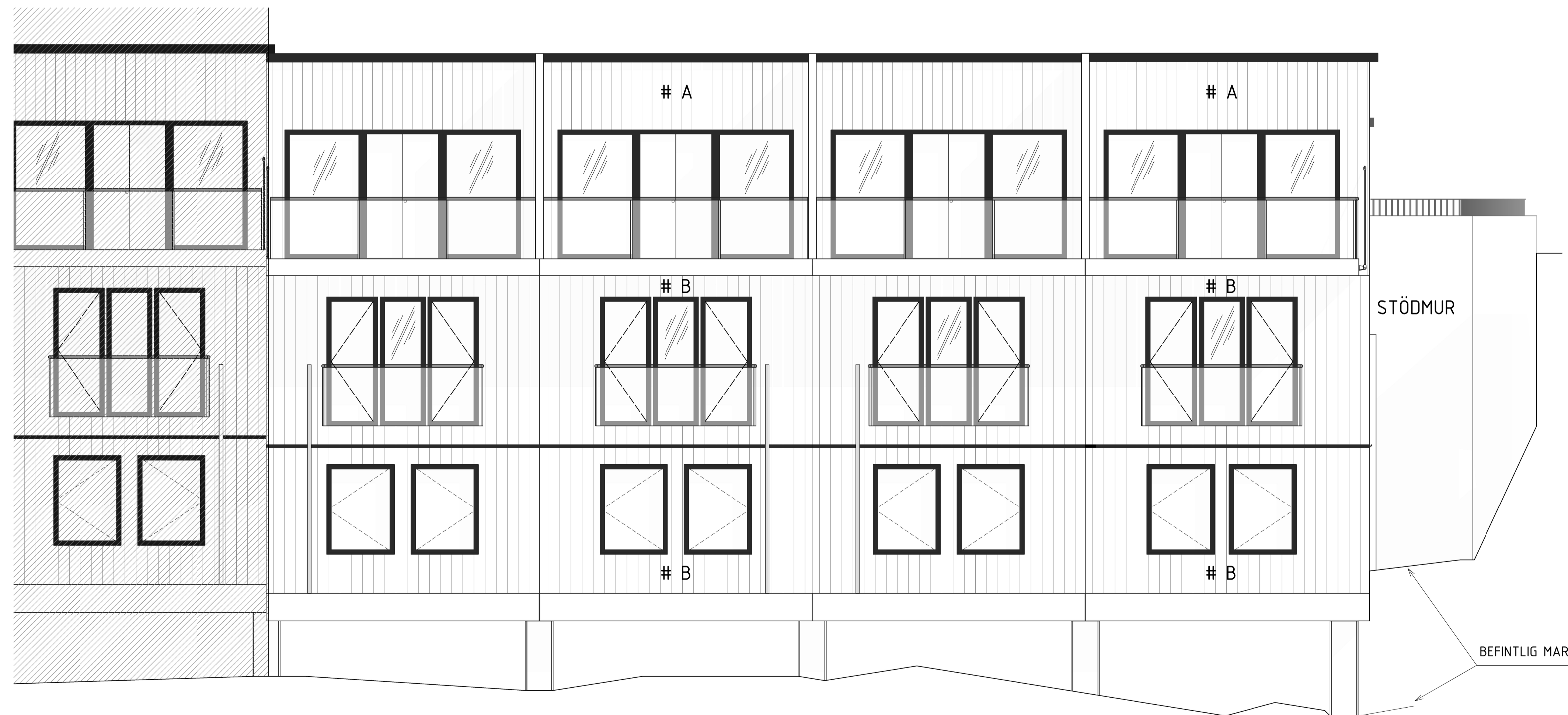
FASAD FRAMSIDA, ENTRÉFASAD ENHET 1-4
