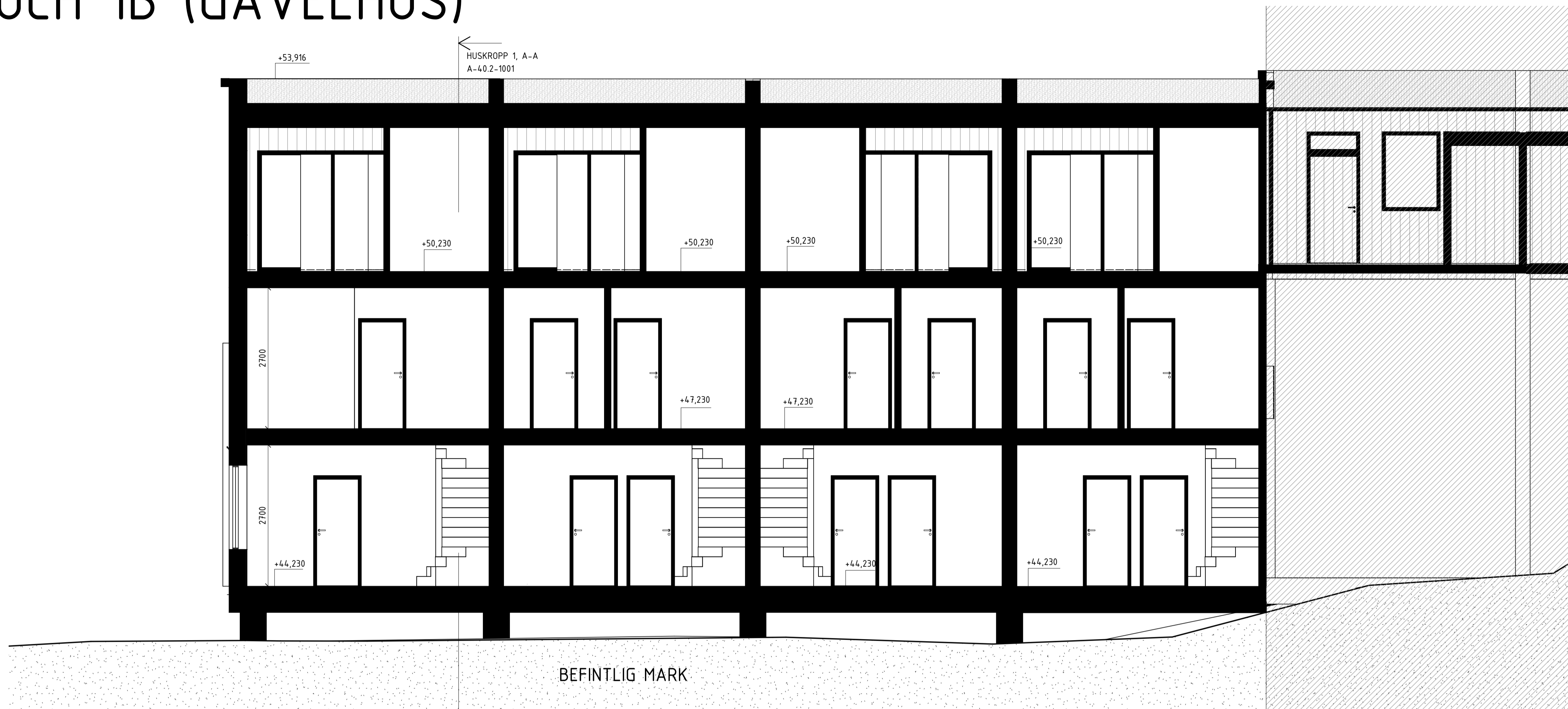
SEKTION C-C ENHET 1-4
