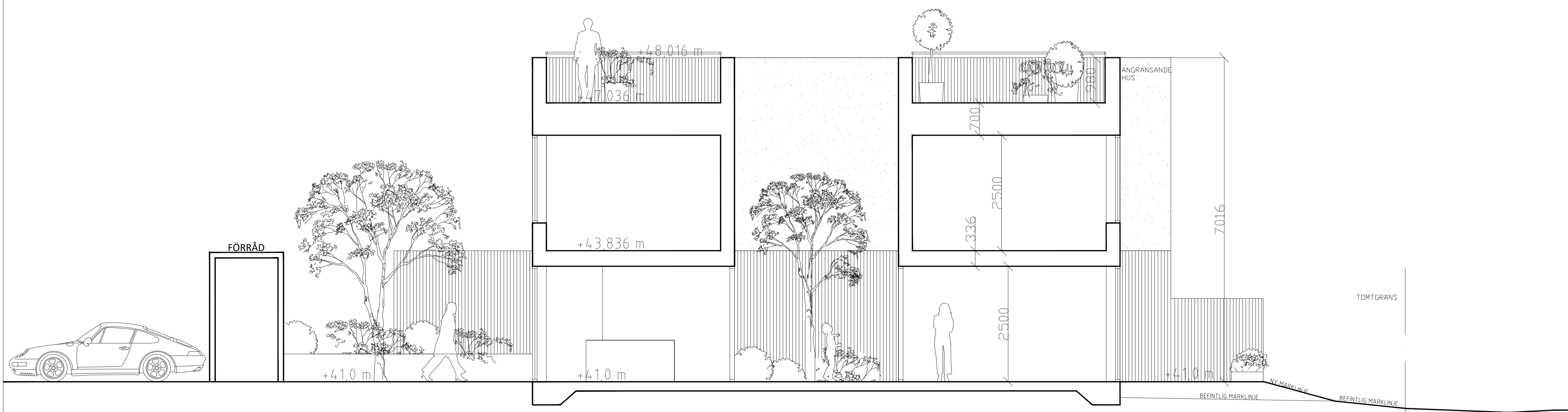
SEKTION BB
