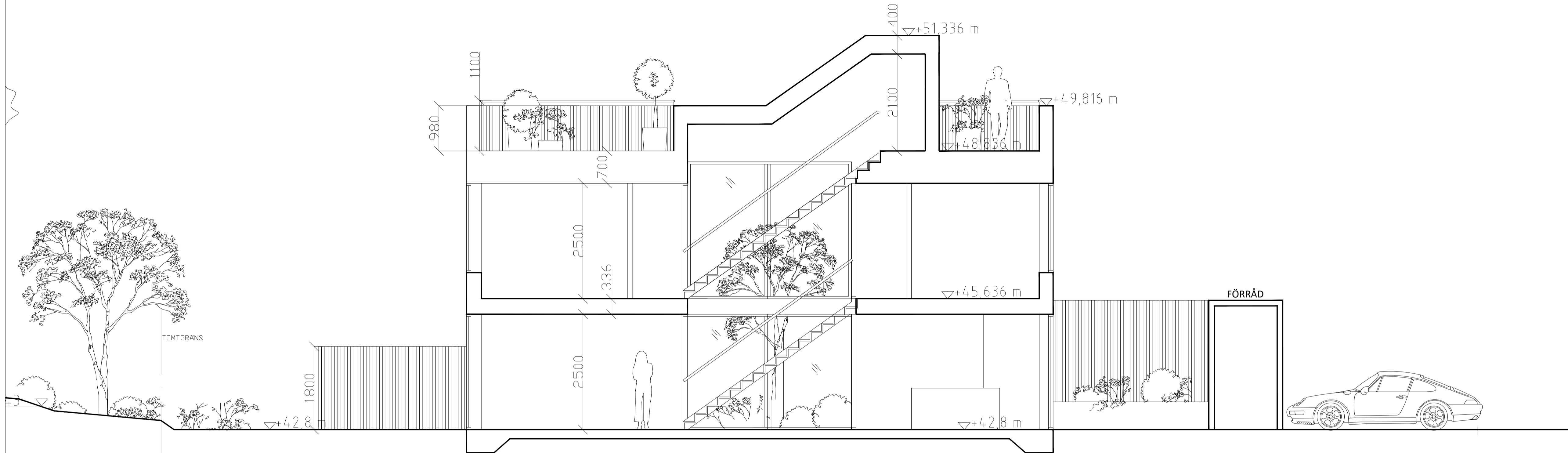
SEKTION AA
