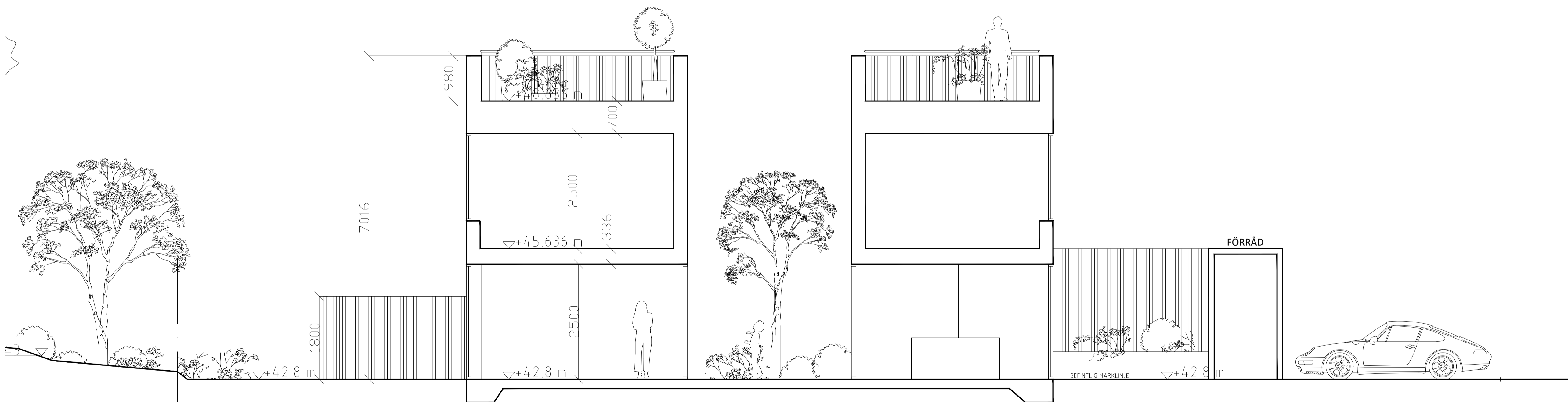
SEKTION AA
