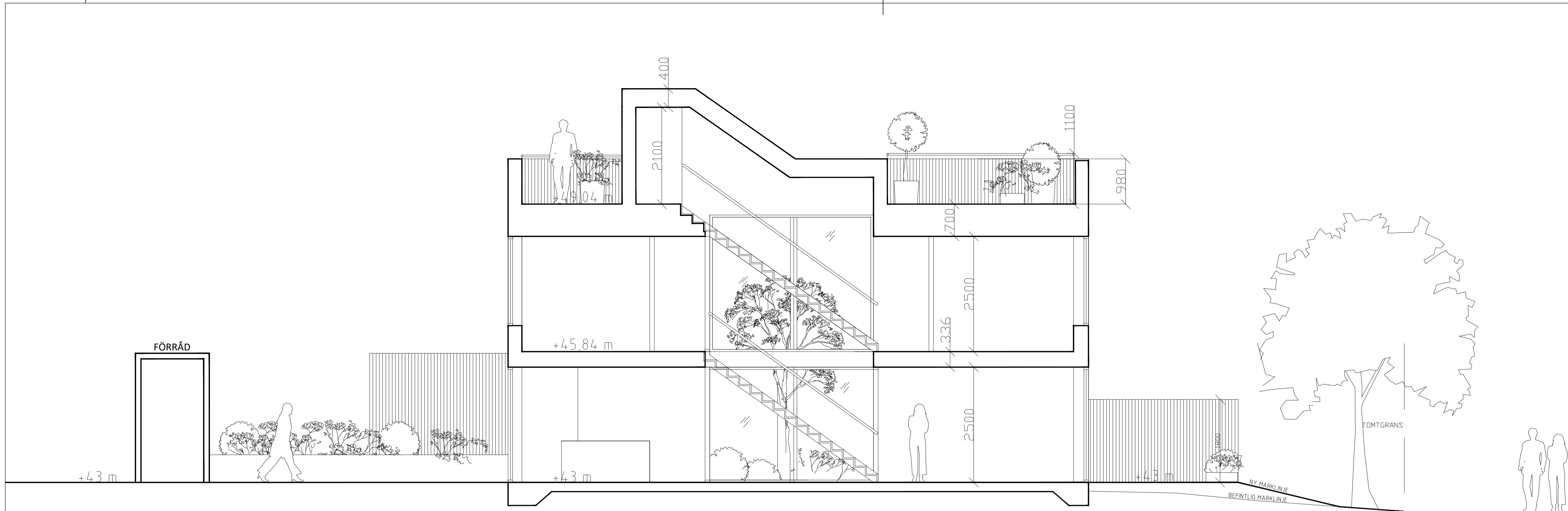
SEKTION AA
