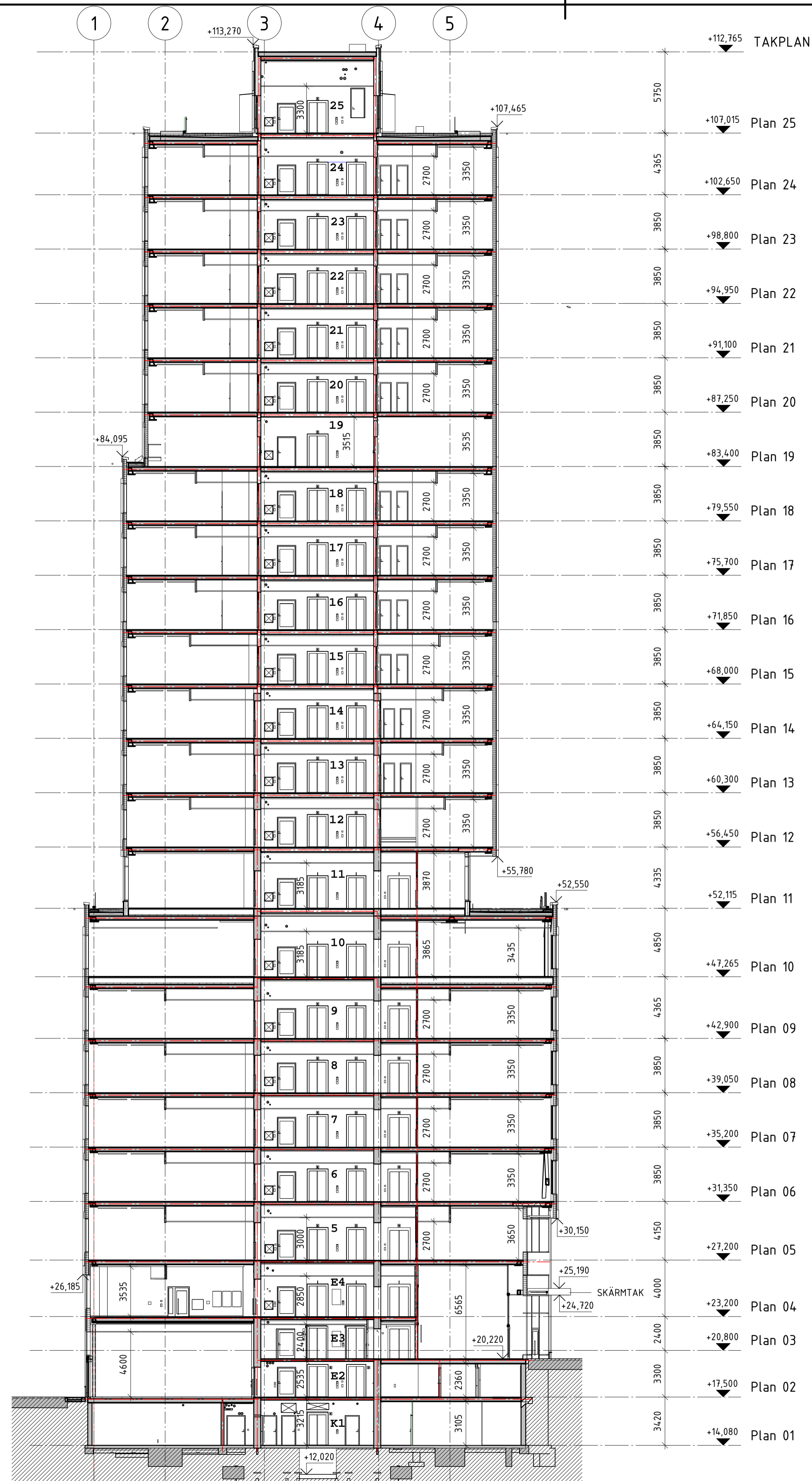
SKALA 1:200 0 1 2 5 10 15 20 METER
