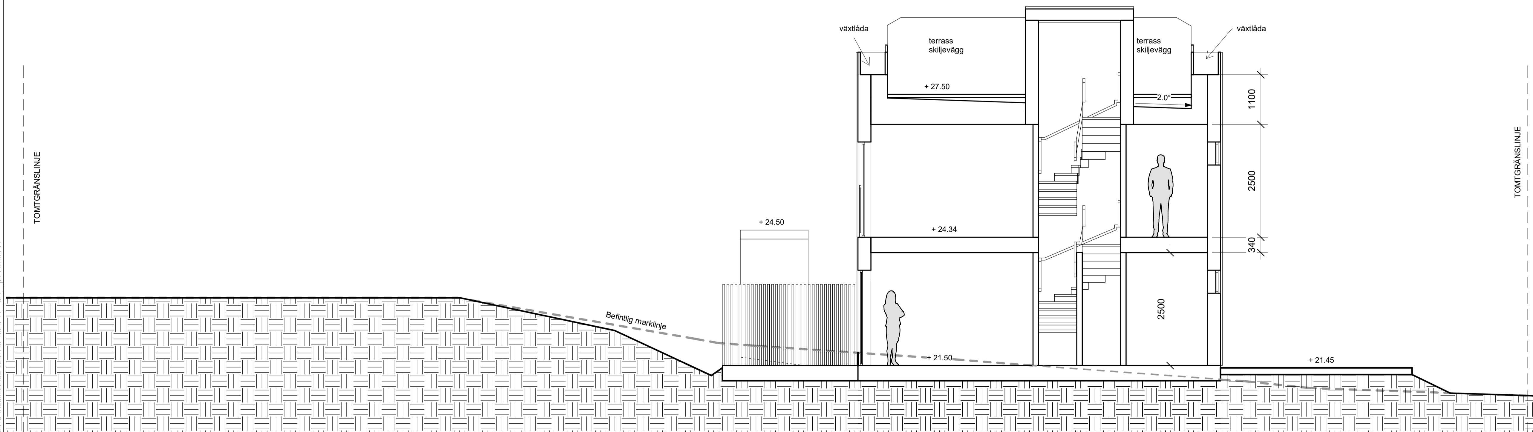
SEKTION B-B
