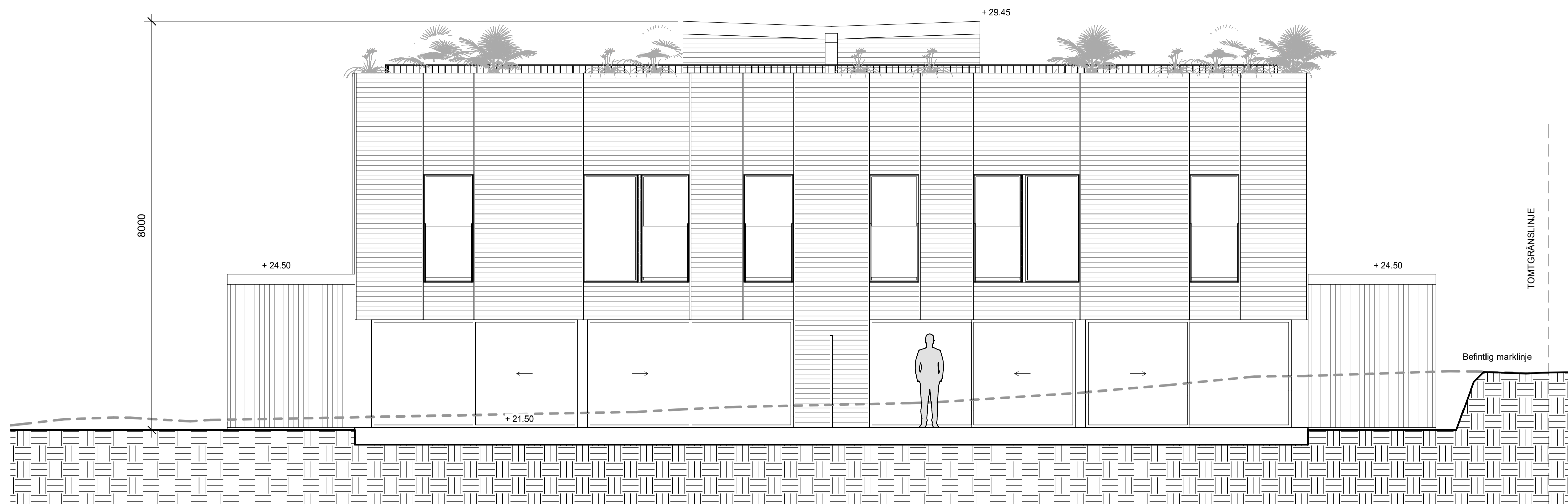
FASAD NORDOST
