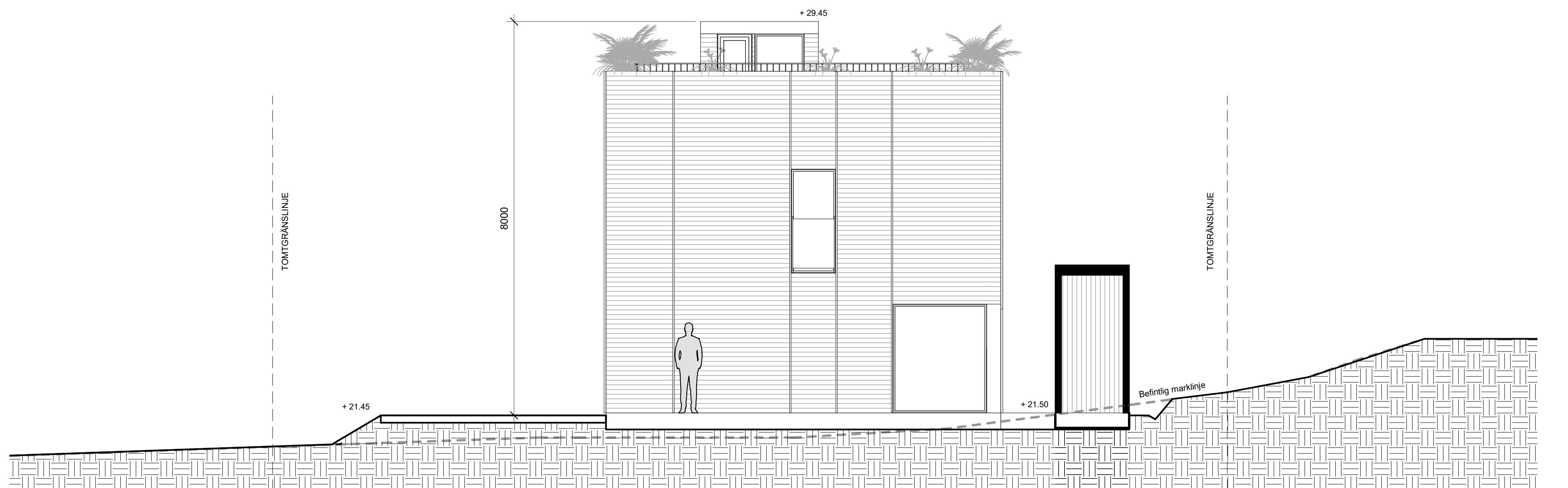
FASAD SYDOST
