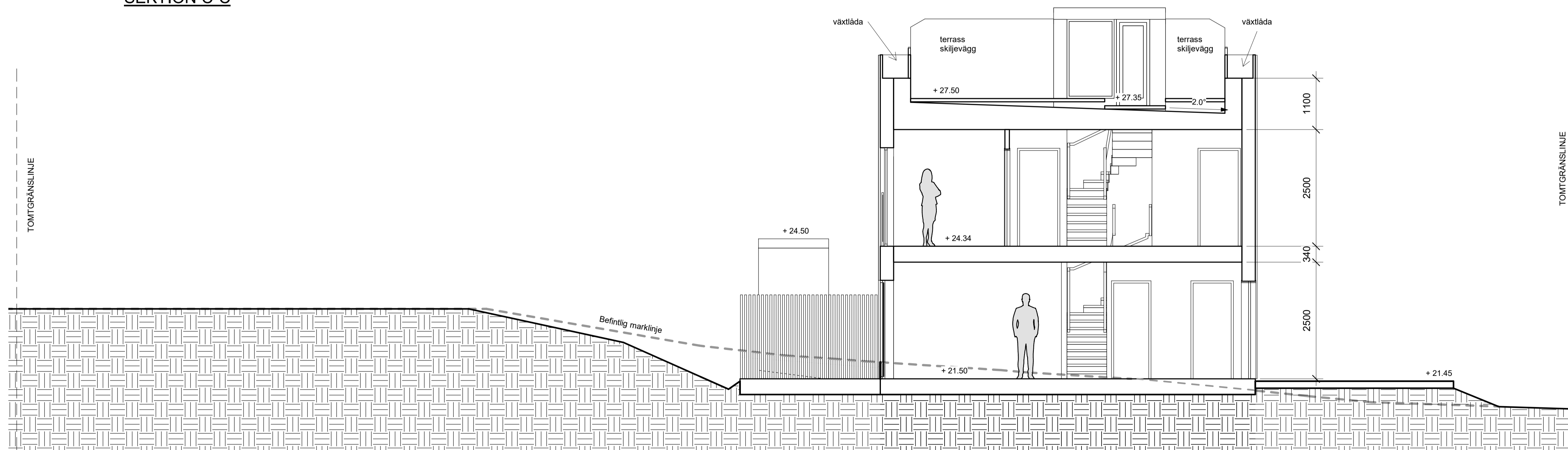
SEKTION C-C
