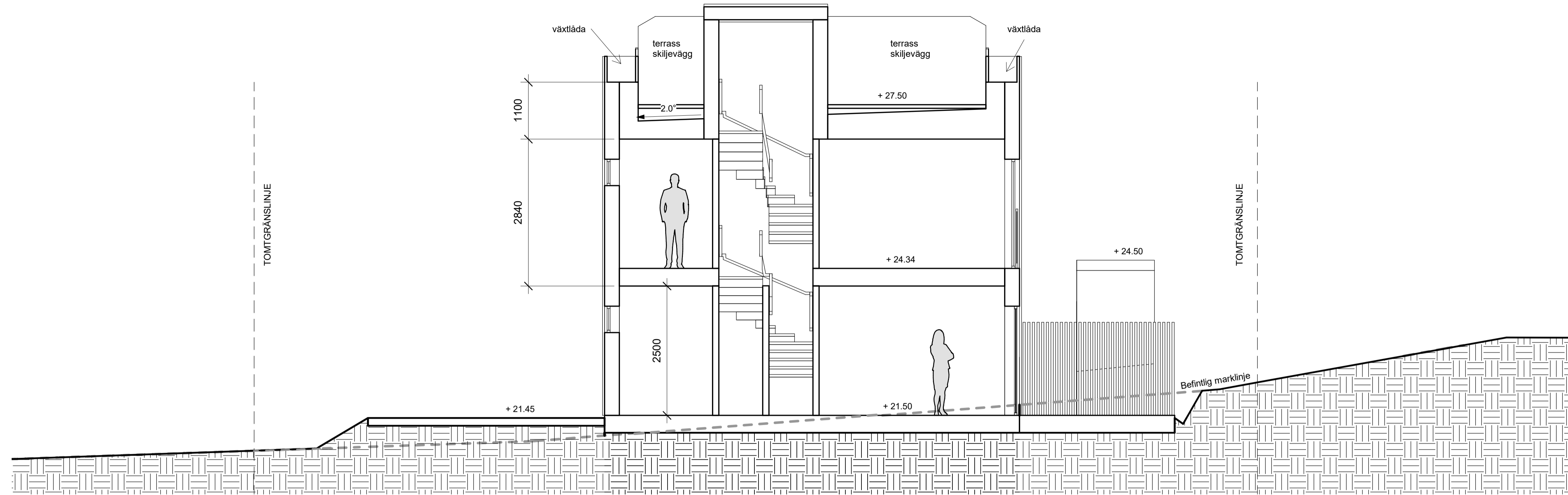
SEKTION A-A
