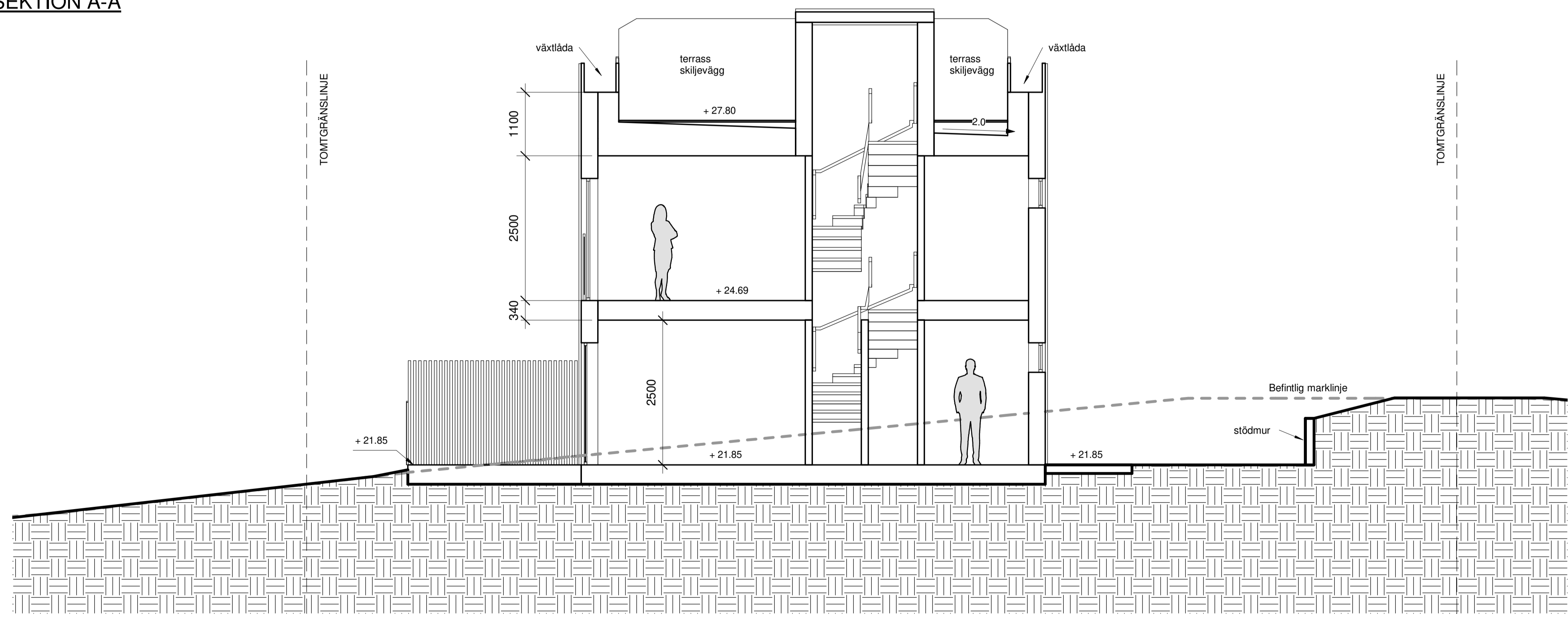
SEKTION A-A
