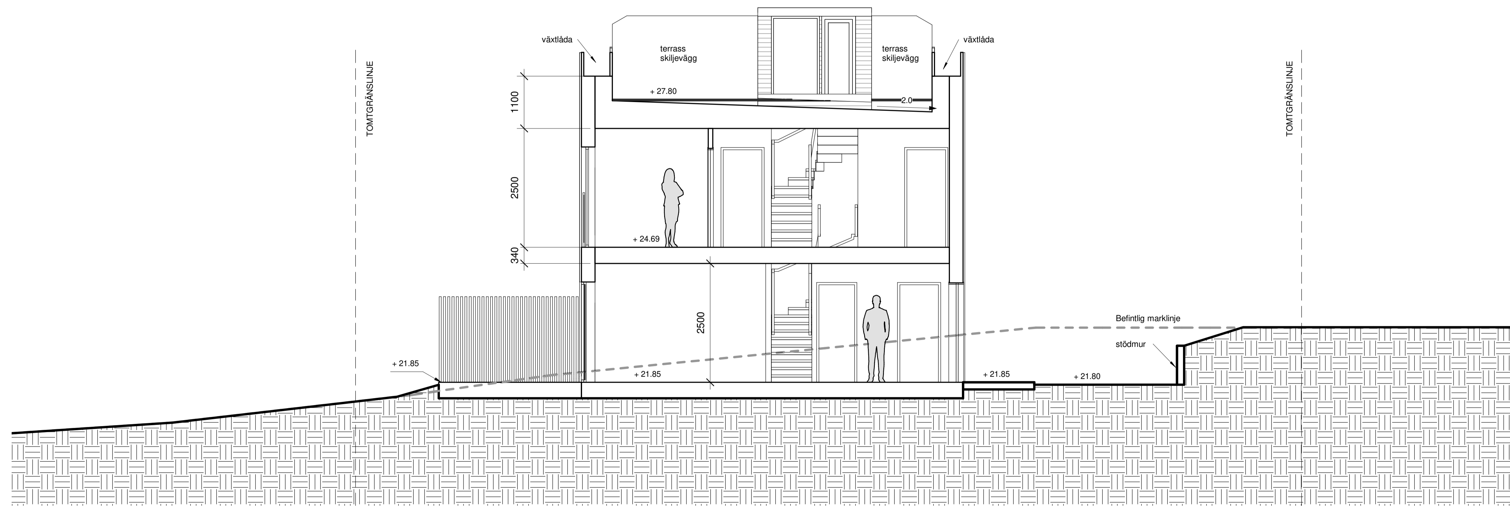
SEKTION D-D
