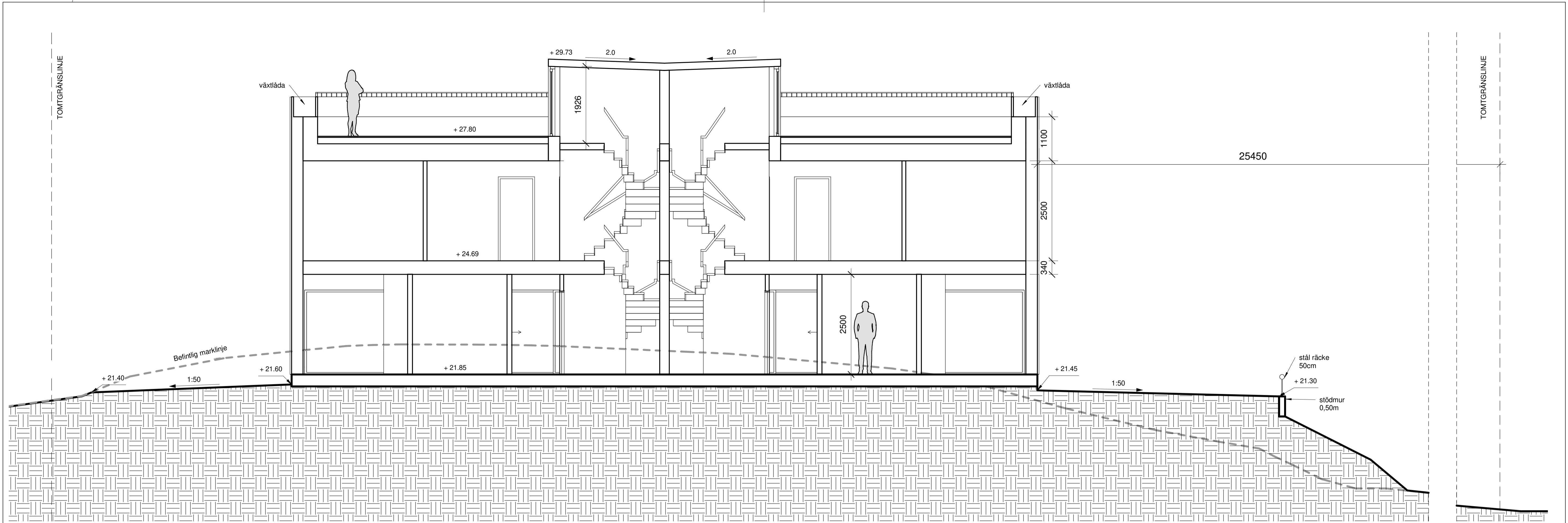
SEKTION C-C
