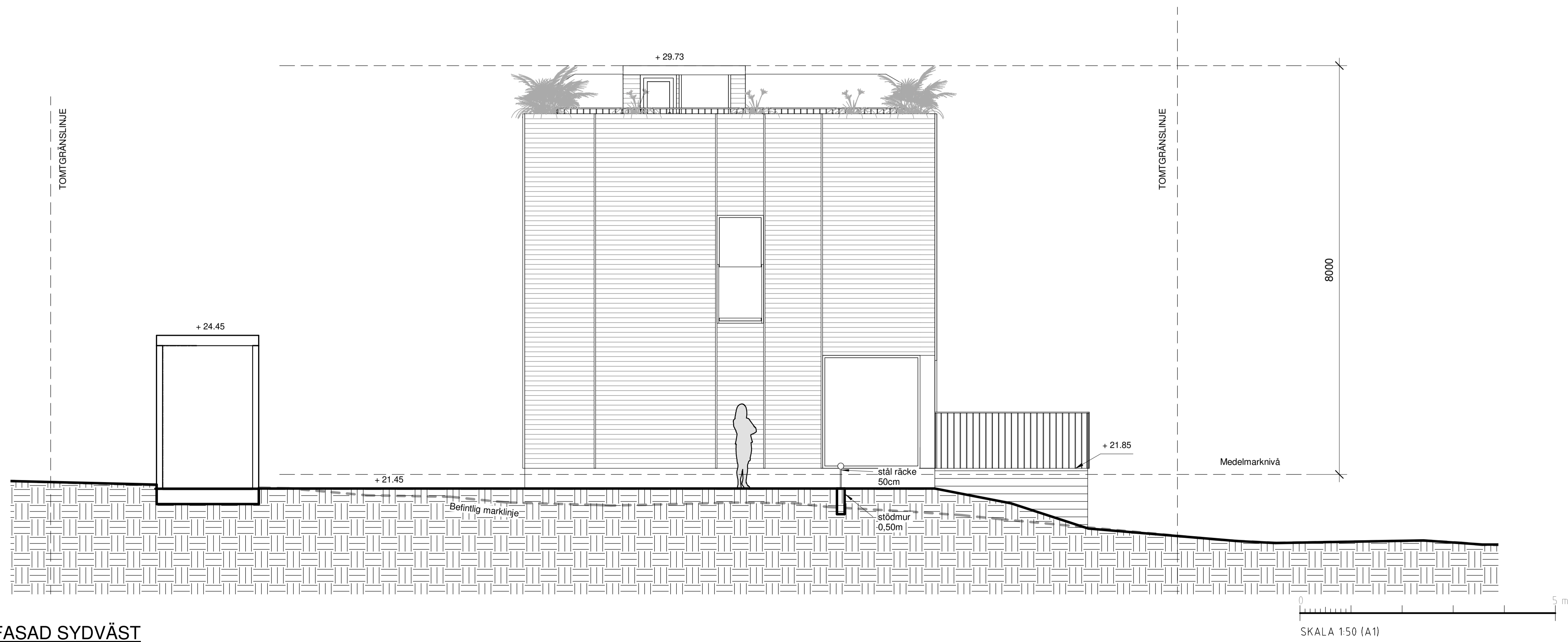
FASAD NORDOST
