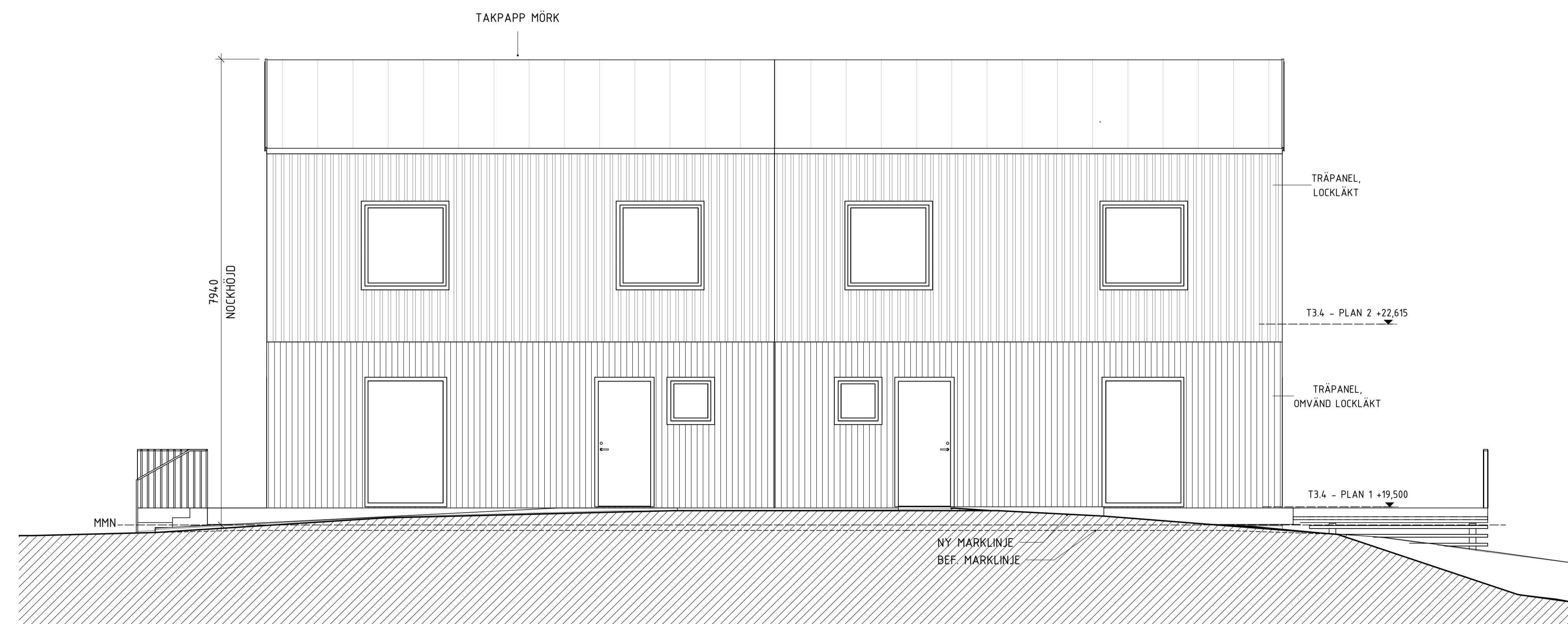
FASAD MOT NORDVÄST
