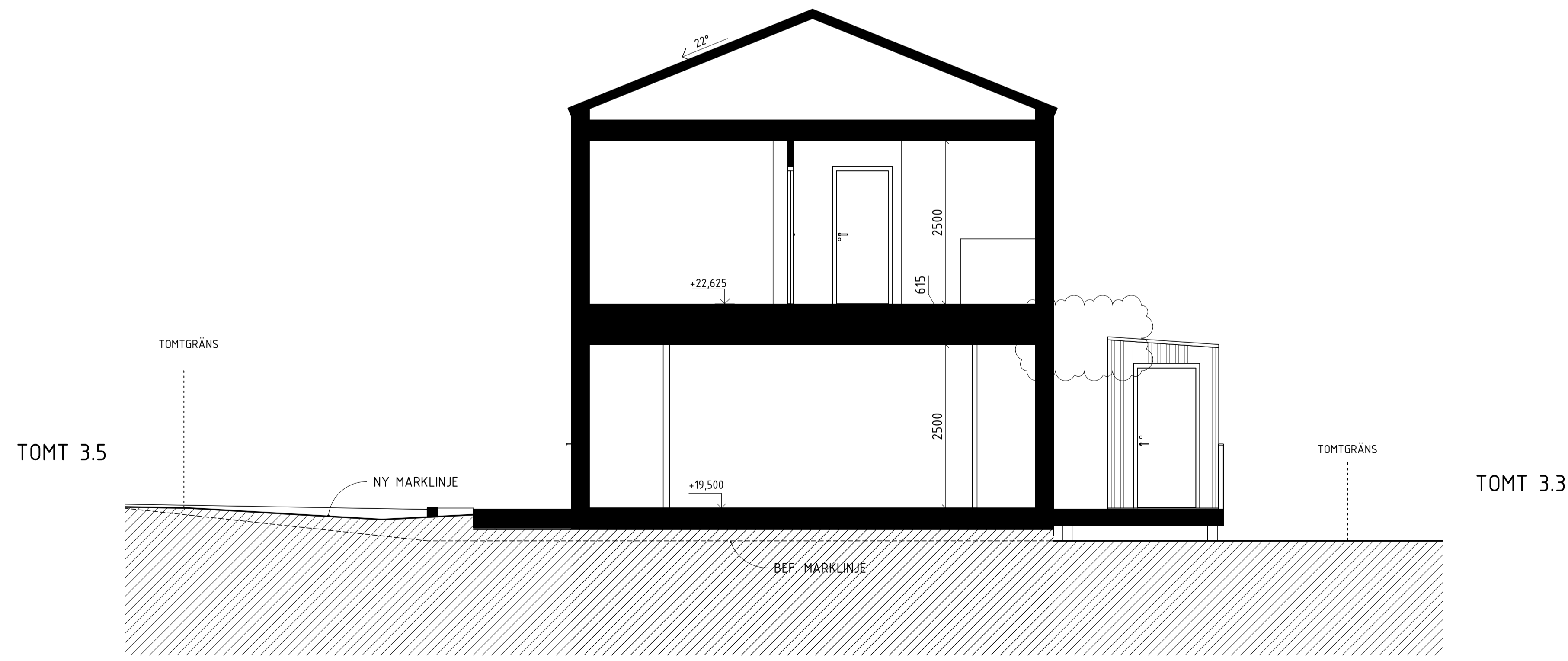
SEKTION A-A
