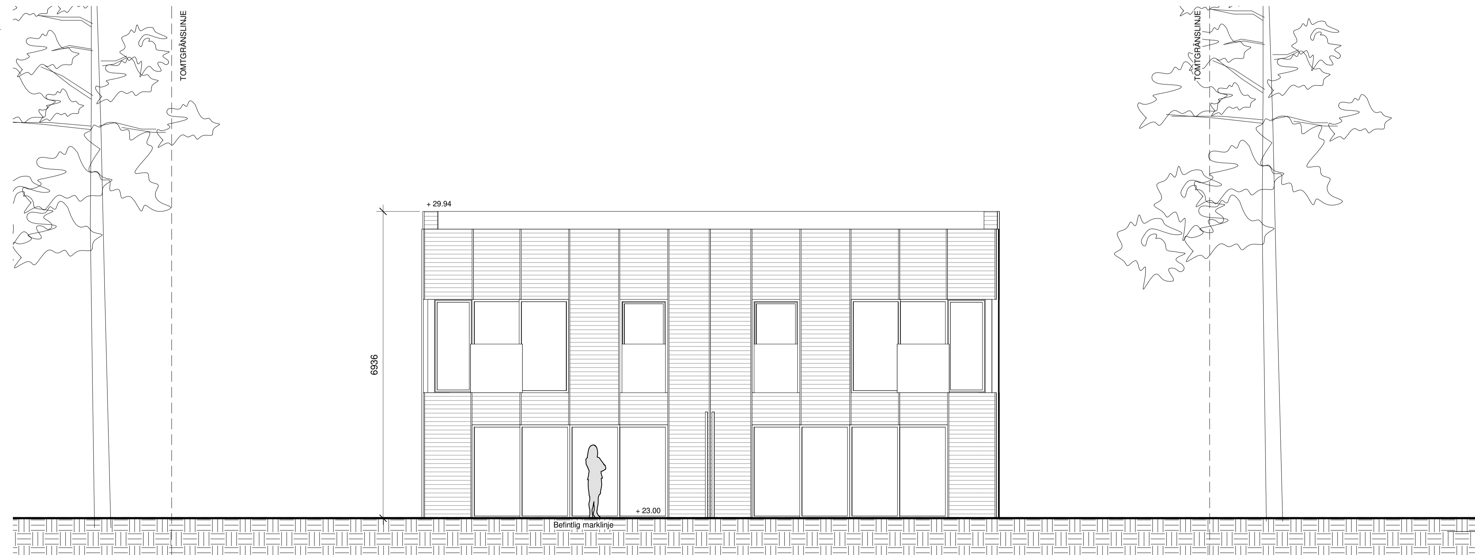
FASAD SYDVÄST
