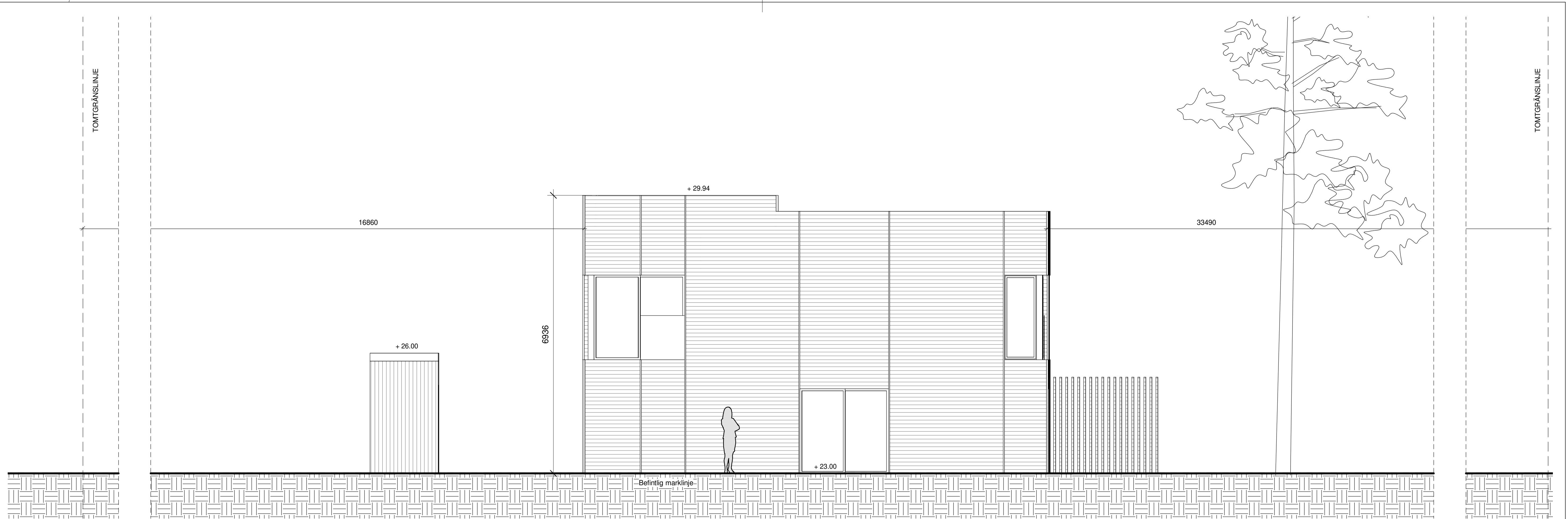
FASAD NORDVÄST
