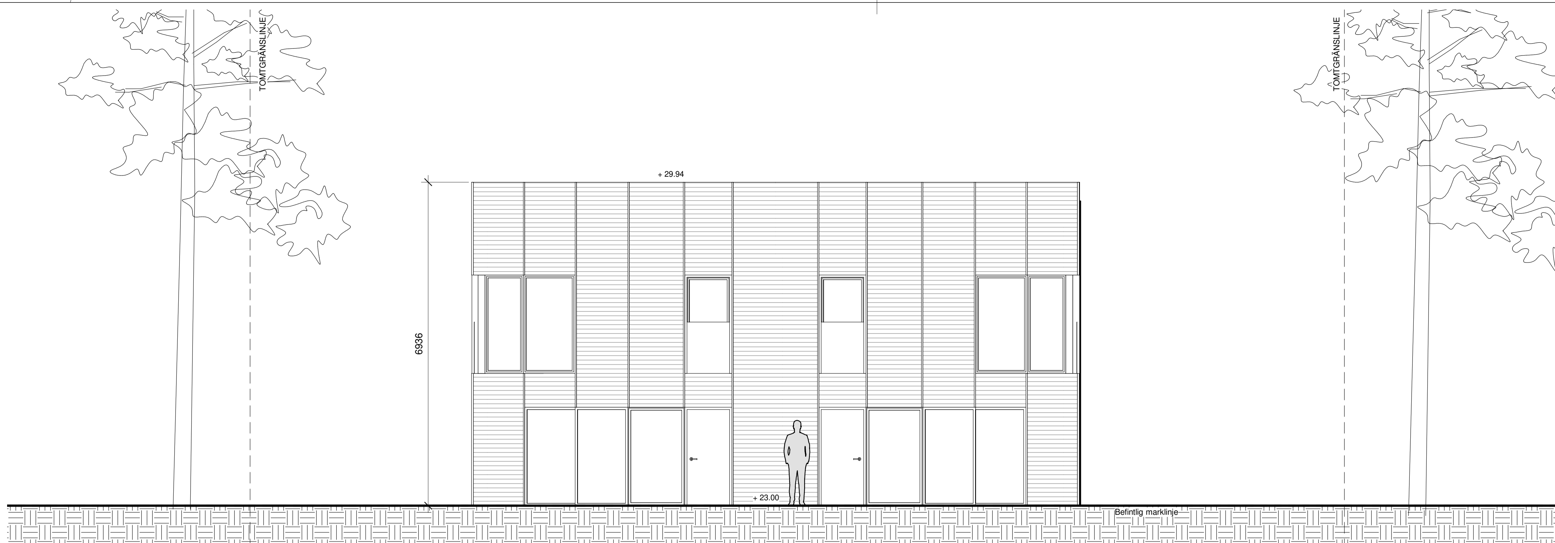
FASAD NORDOST
