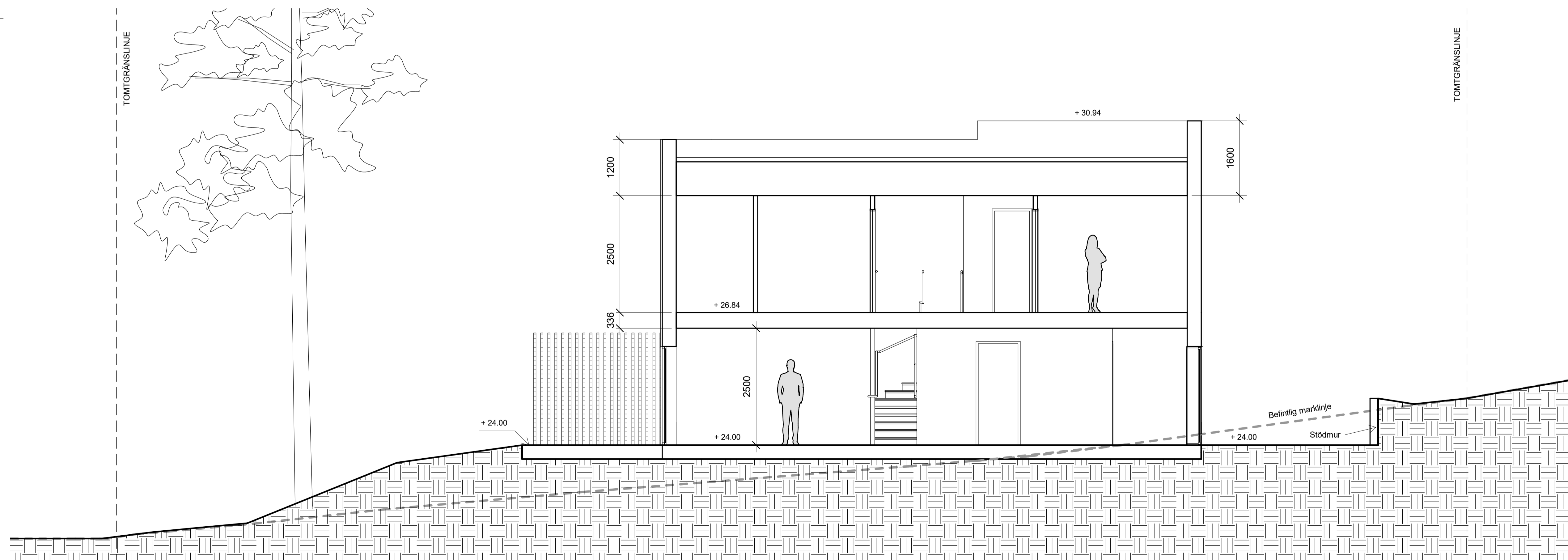
SEKTION B-B
