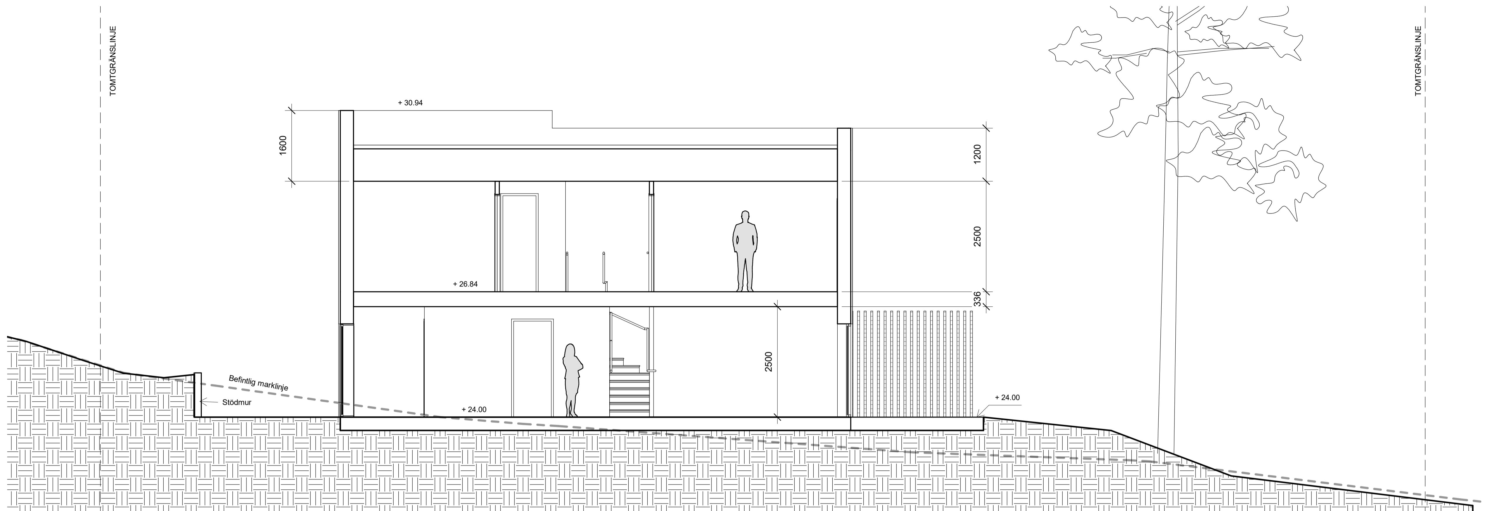
SEKTION B-B
