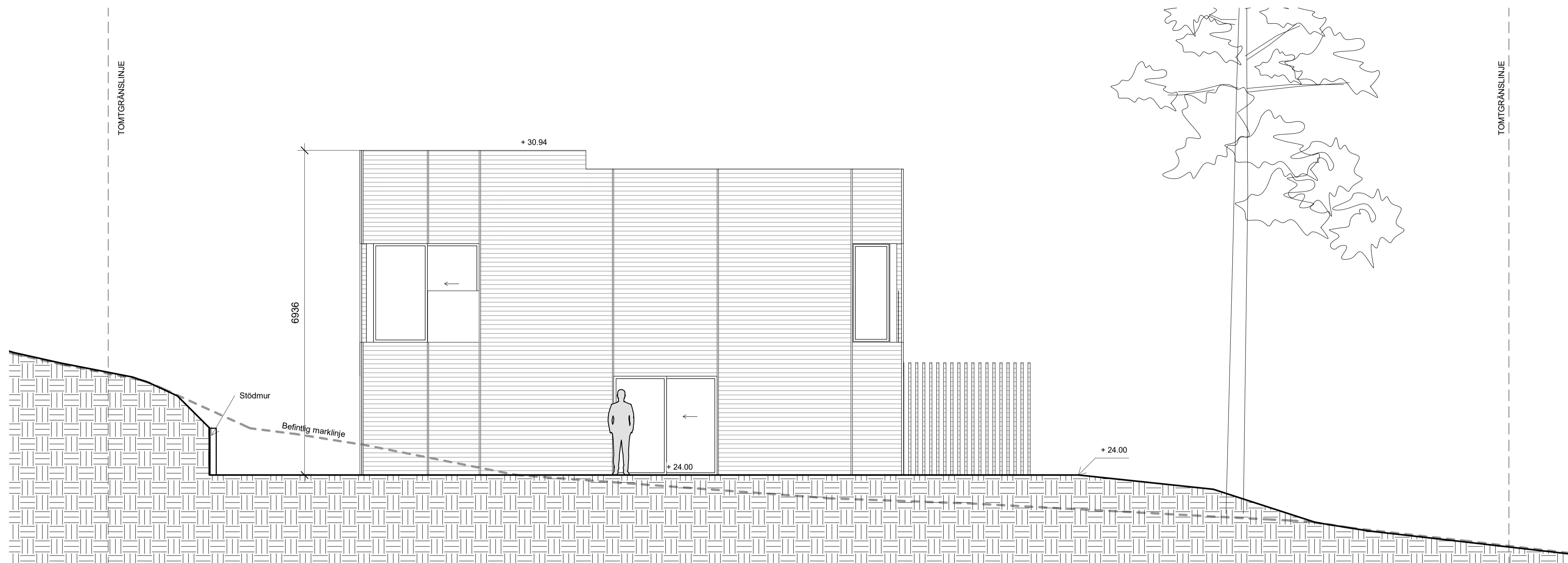
FASAD NORR
