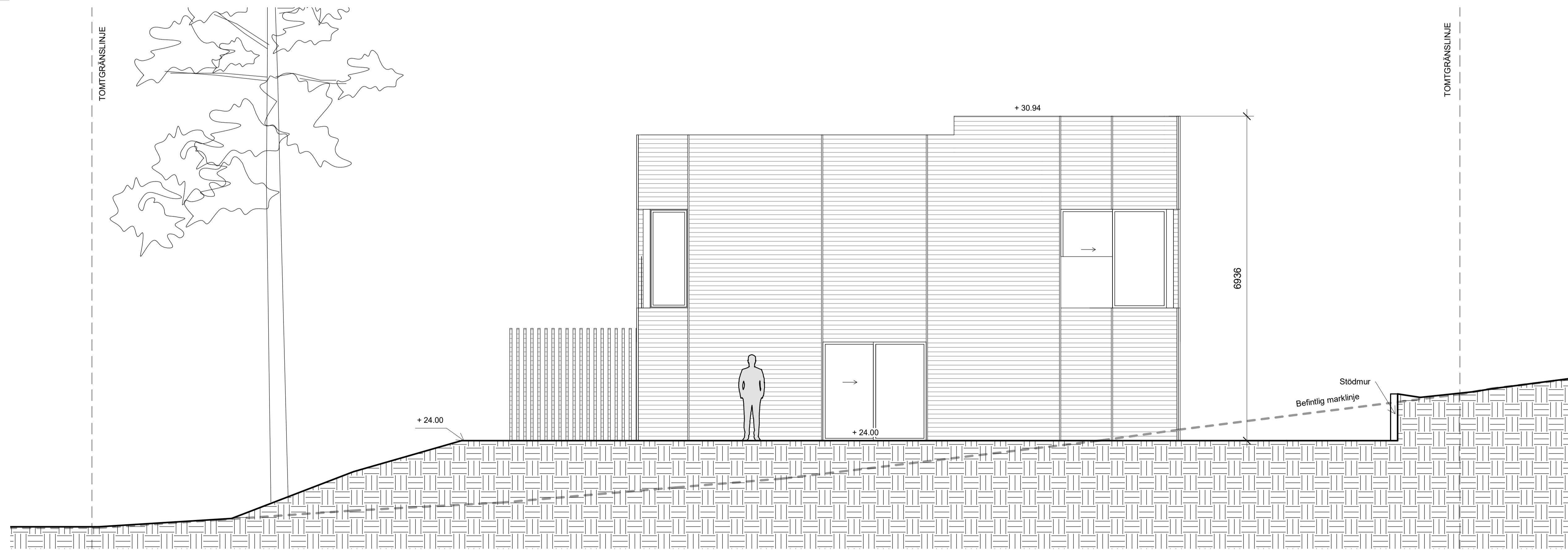
FASAD SÖDER
