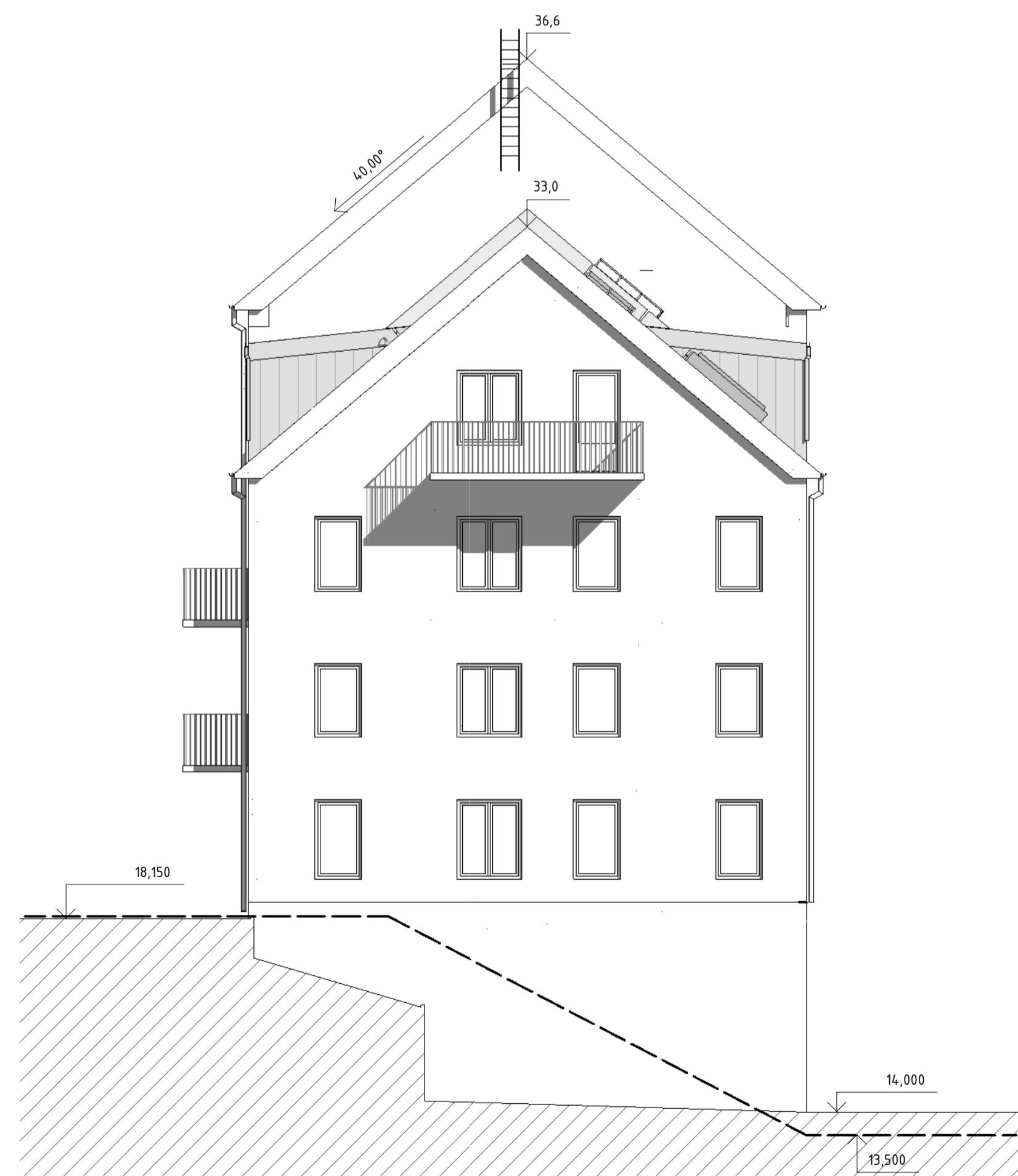
Elevation mot söder
