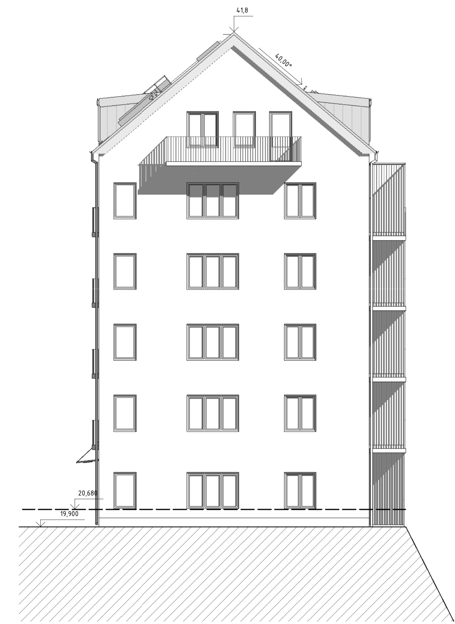
Elevation mot väst
