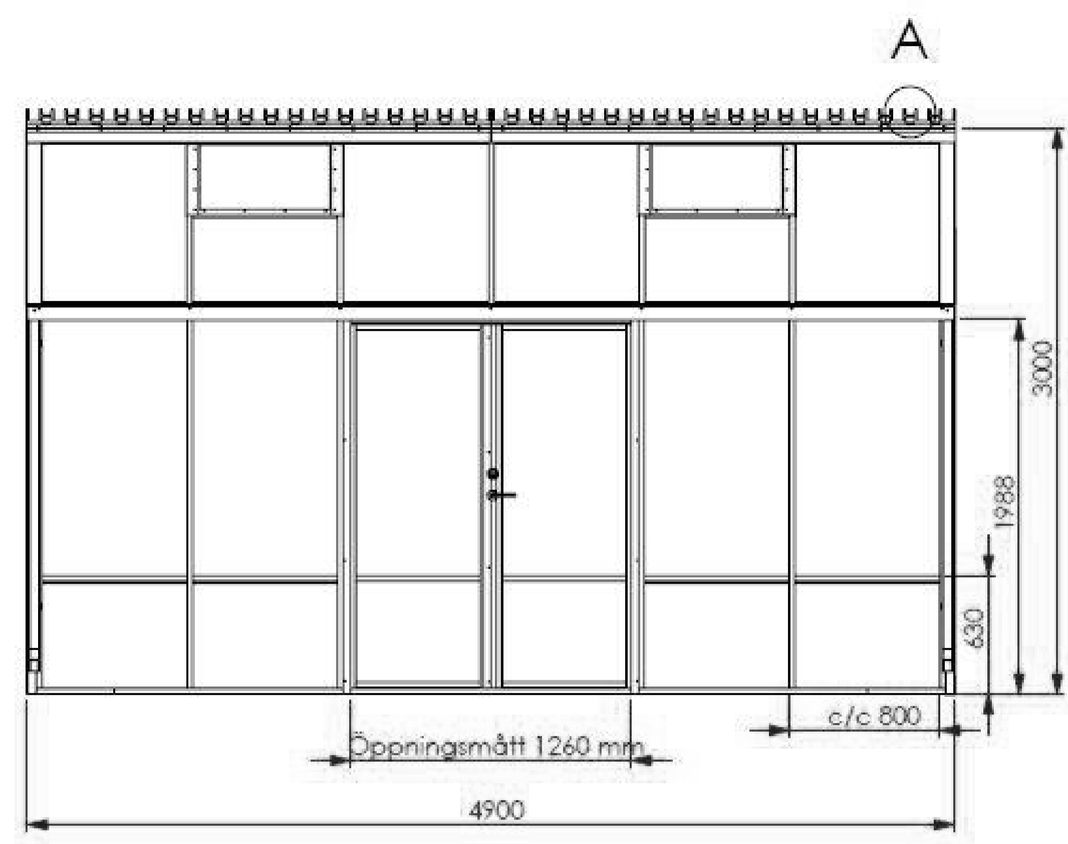
Fasad mot syd & norr Vid fasad mot norr utgår dörr och ersätts av väggsektion. Elevation 1:20/A1
