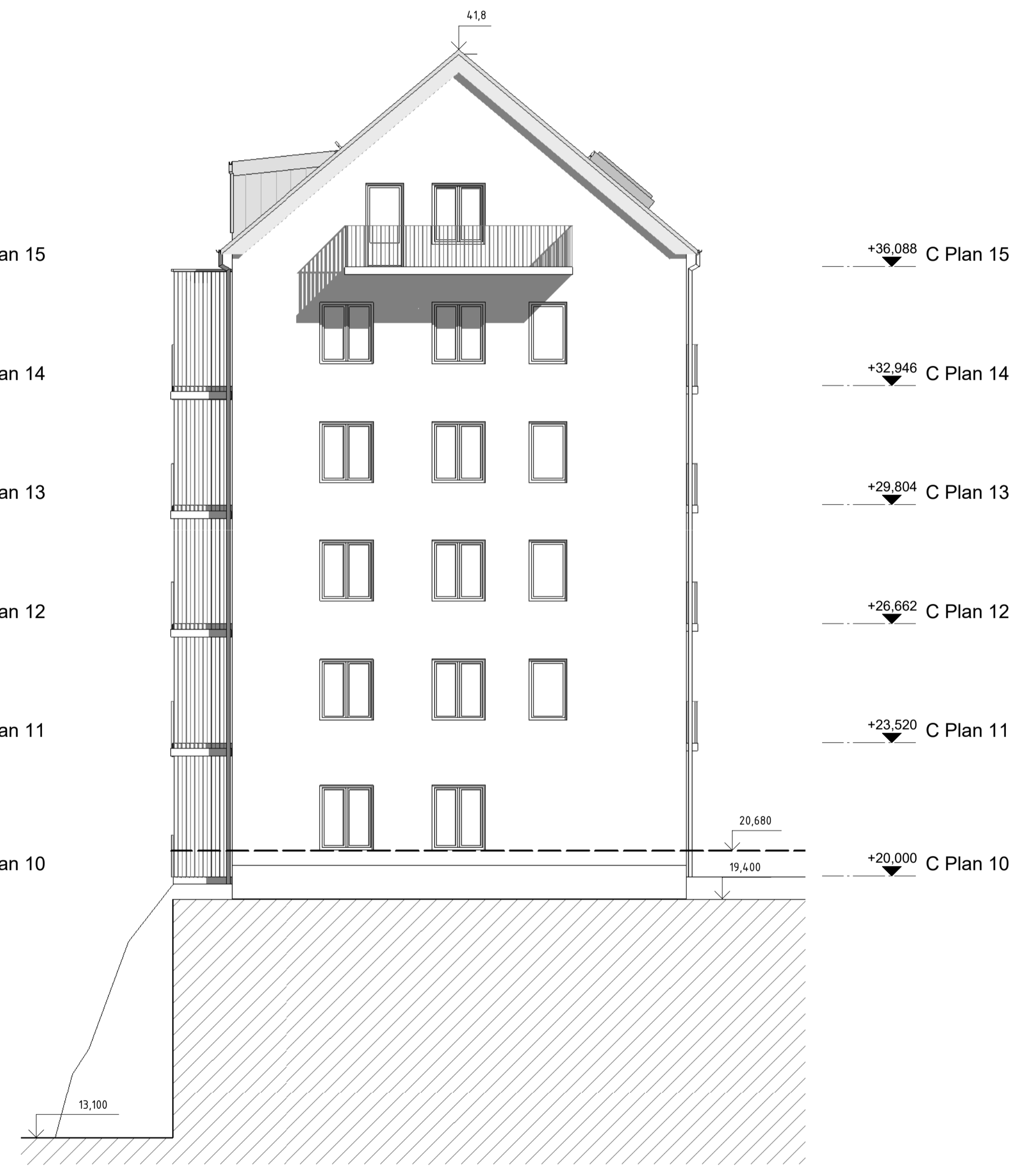
Elevation mot öst
