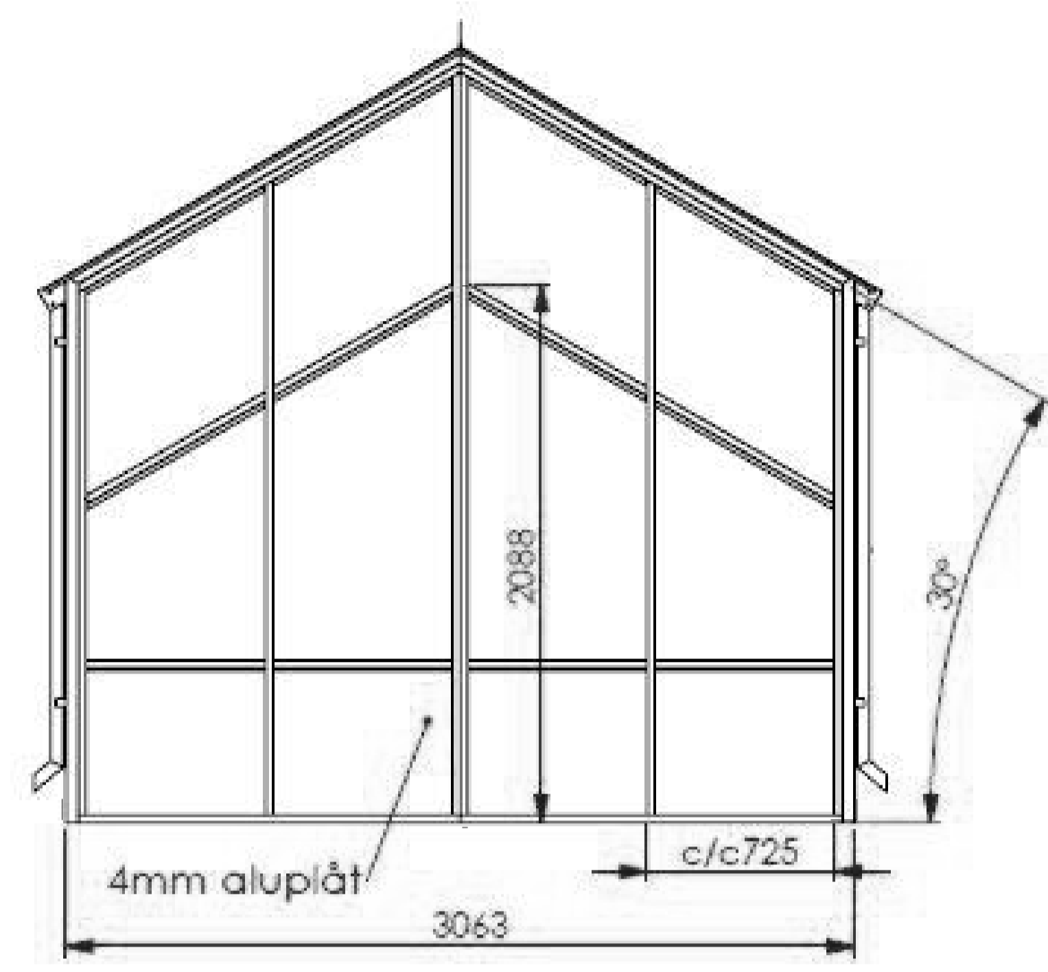
Fasad mot öst & väst Elevation 1:20/A1
