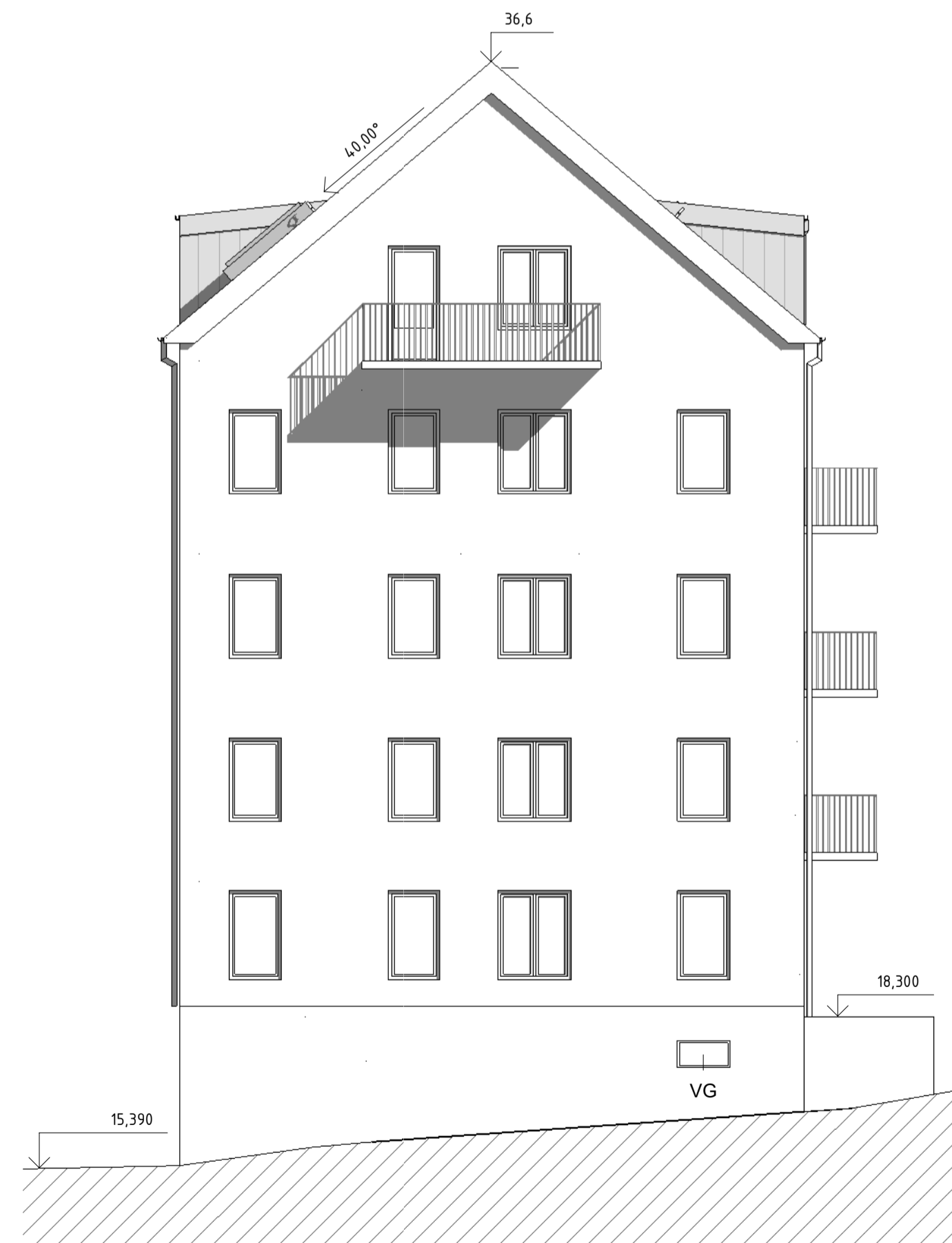
Elevation mot norr
