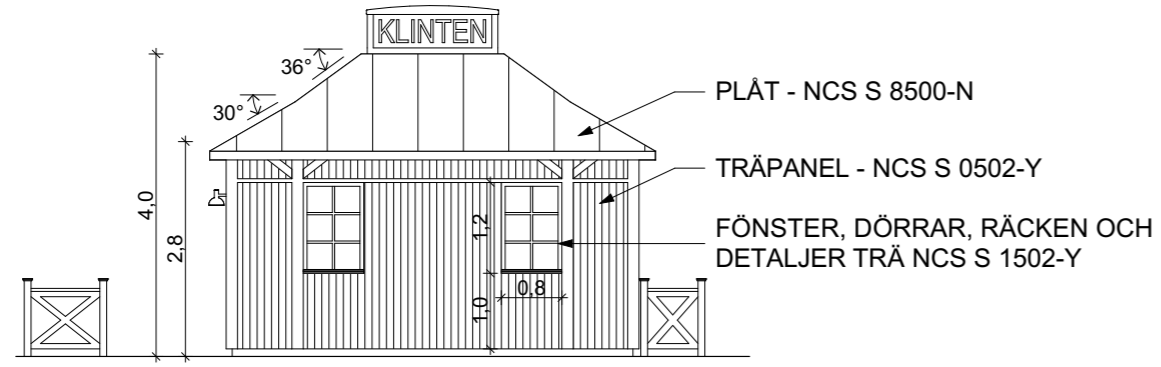
FASAD A1 - MOT SYDOST
