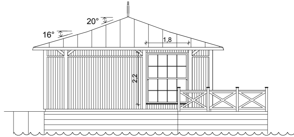
FASAD A2 - MOT NORDOST
