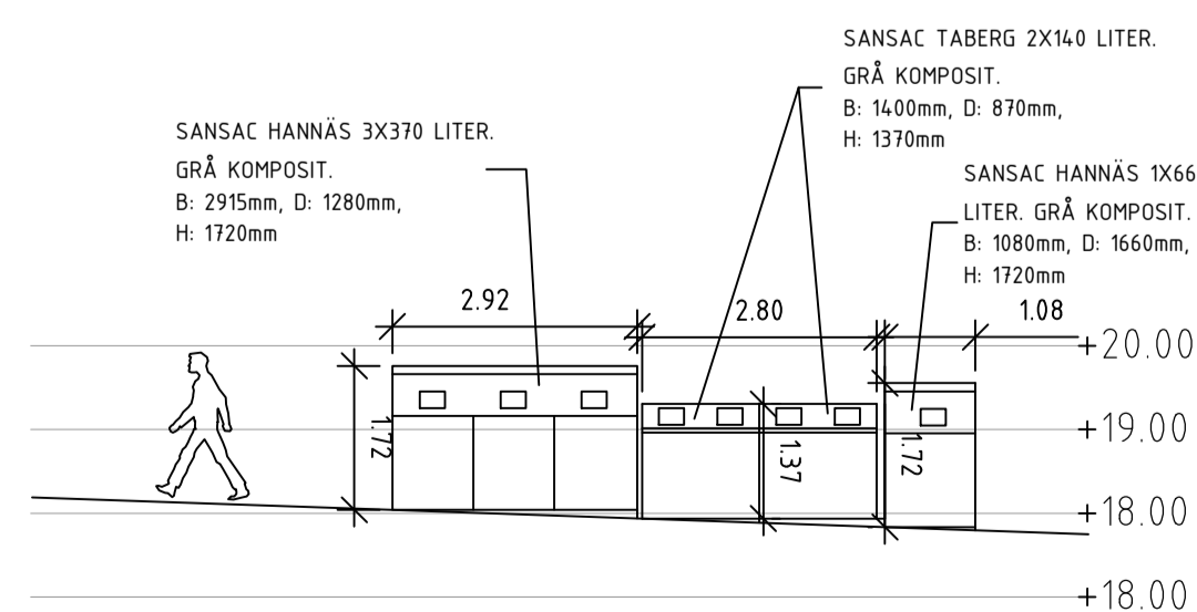
SKALA 1:100 ELEVATION AVFALLSSKÅP
