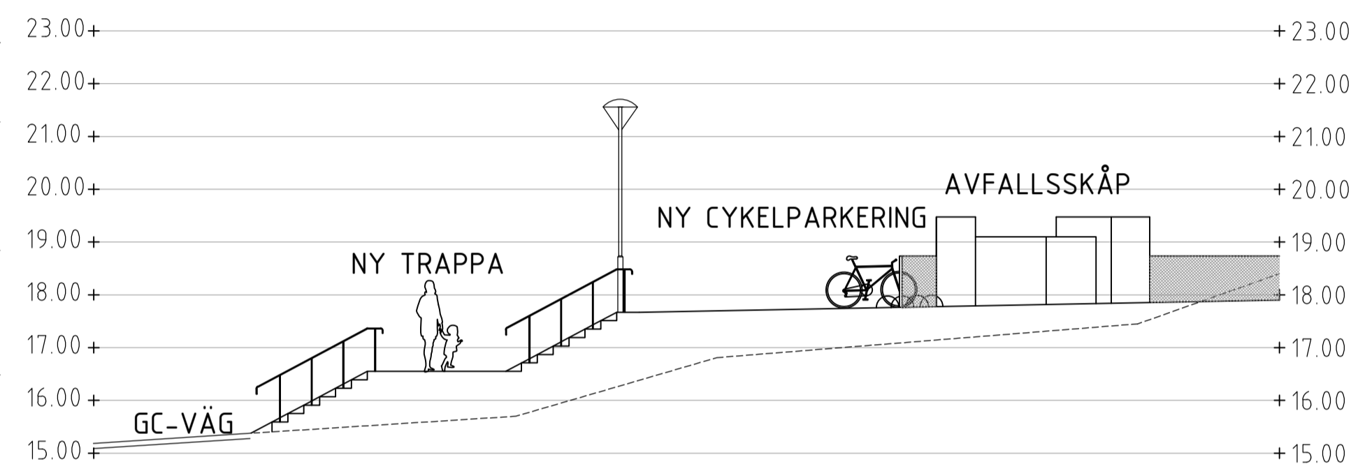
SKALA 1:100 ELEVATION 2'-2 MOT VÄST
