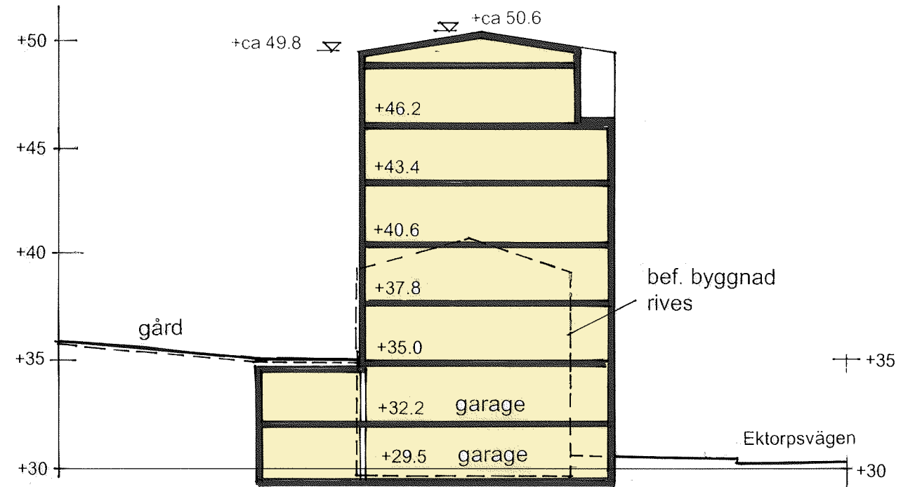
Sektion A-A 1:250
