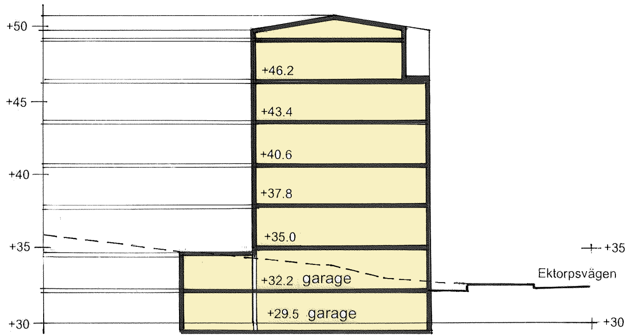
Sektion B-B
