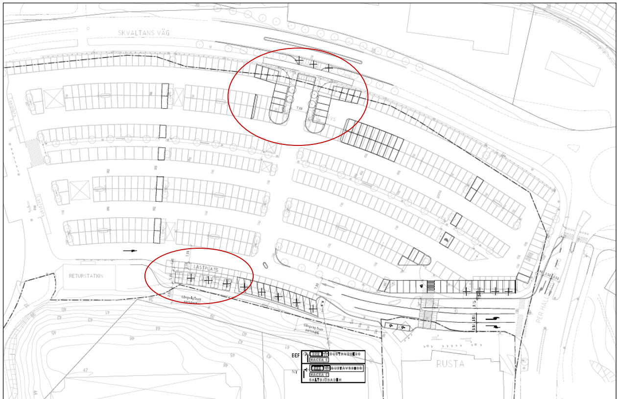
Figur 1. Illustration över föreslagen utformning. Planändringar markerade. (Från: Ombyggnadsförslag parkeringsplats, ritning P02.10002. 2014-07-01 av Grontmij.)
