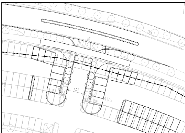
Figur 2. Utfart mot Skvaltans väg. (kryss indikerar träd som behöver tas ner). (Bilder från: Ombyggnadsförslag parkeringsplats, ritning P02.10002. 2014-07-01 av Grontmij.)
