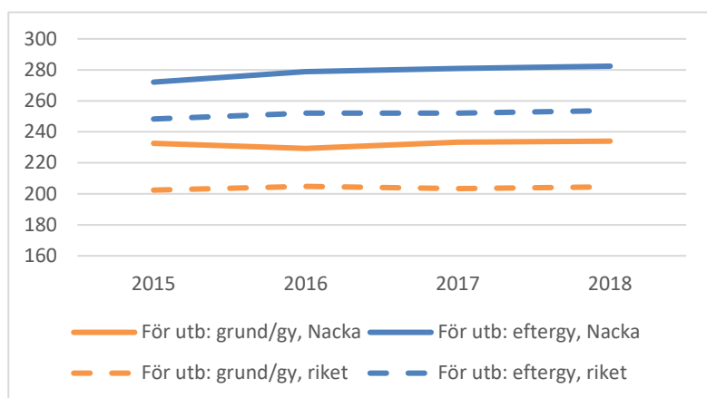
Figur 8 Genomsnittligt meritvärde åk 9 våren 2015-2018, efter föräldrarnas högsta utbildningsnivå (Nacka och riket)
