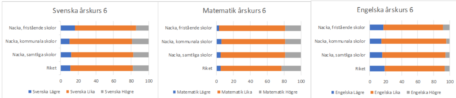
Figur 11: Andel (%) elever med lägre, lika eller högre slutbetyg än provbetyget, årskurs 6, våren 2018
