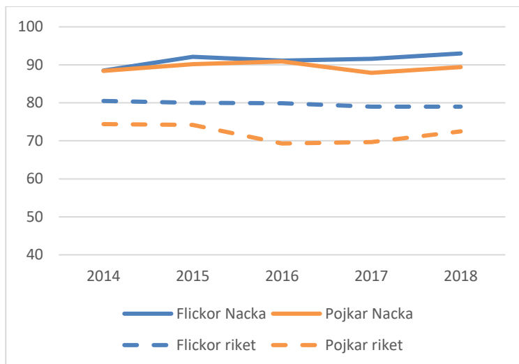
Figur 5 Andelen elever (%) som nått kunskapskraven i alla ämnen i åk 9, efter kön och totalt, i Nacka och riket
