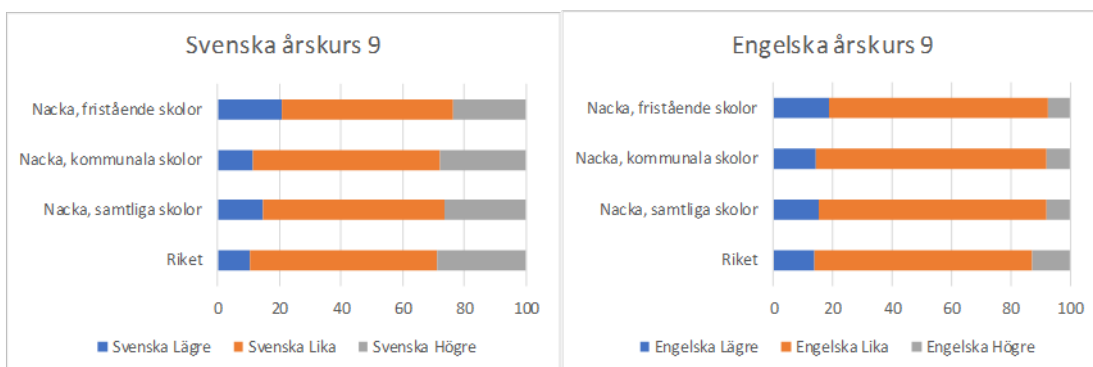
Figur 12: Andel (%) elever med lägre, lika eller högre slutbetyg än provbetyget, årskurs 9, våren 2018 (inga resultat i matematik publiceras i år)
