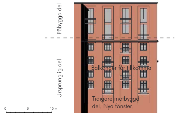
Fasad mot väster, mot gård Hus 3, princip
