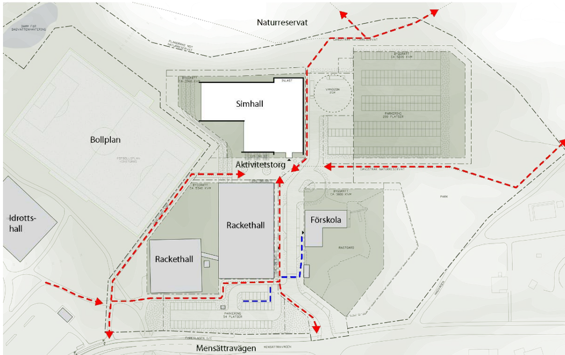
Föreslagna gång- och cykelstråk markerade i rött. Blått streck visar säker väg med upphöjda passager över gata.
