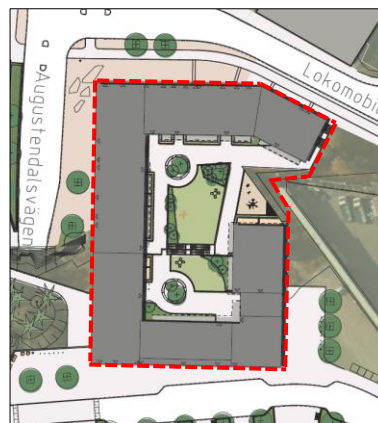
Volymskiss samt situationsplan som illustrerar principen med föreslagen trappande hantering av byggnadsvolymer inom delområde 10. Bild: Kjellander & Sjöberg
