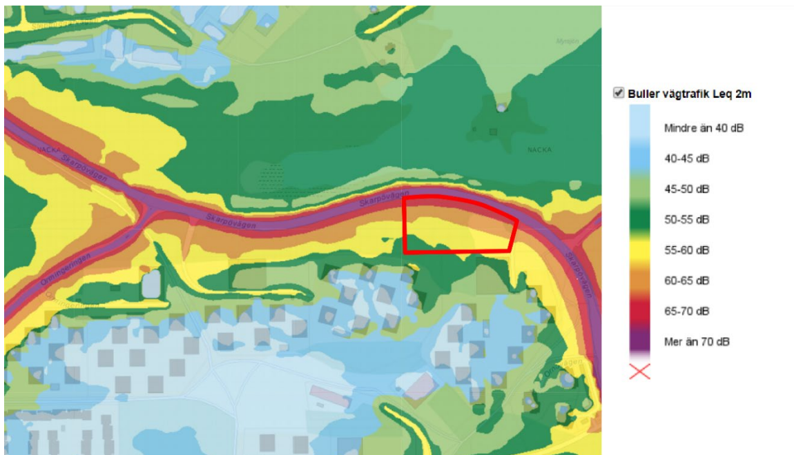
DP Pylonen: buller från vägtrafik, ekvivalent nivå. Plangränsen markerat i rött.
