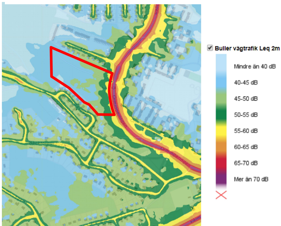
DP Amperen: buller från vägtrafik, ekvivalent nivå. Plangränsen markerat i rött.
