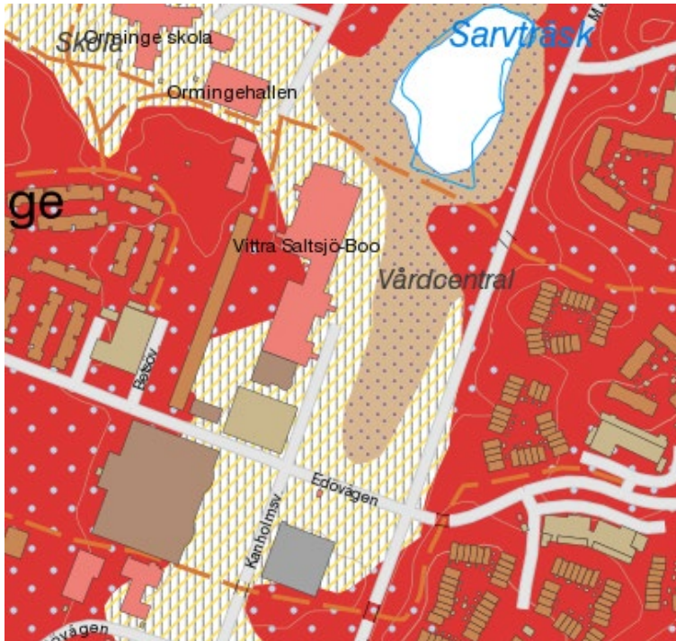
Utdrag från SGU:s jordartskarta. Rödmarkering urberg, brun källror, gulstreckad postglacial lera och fyllning.
