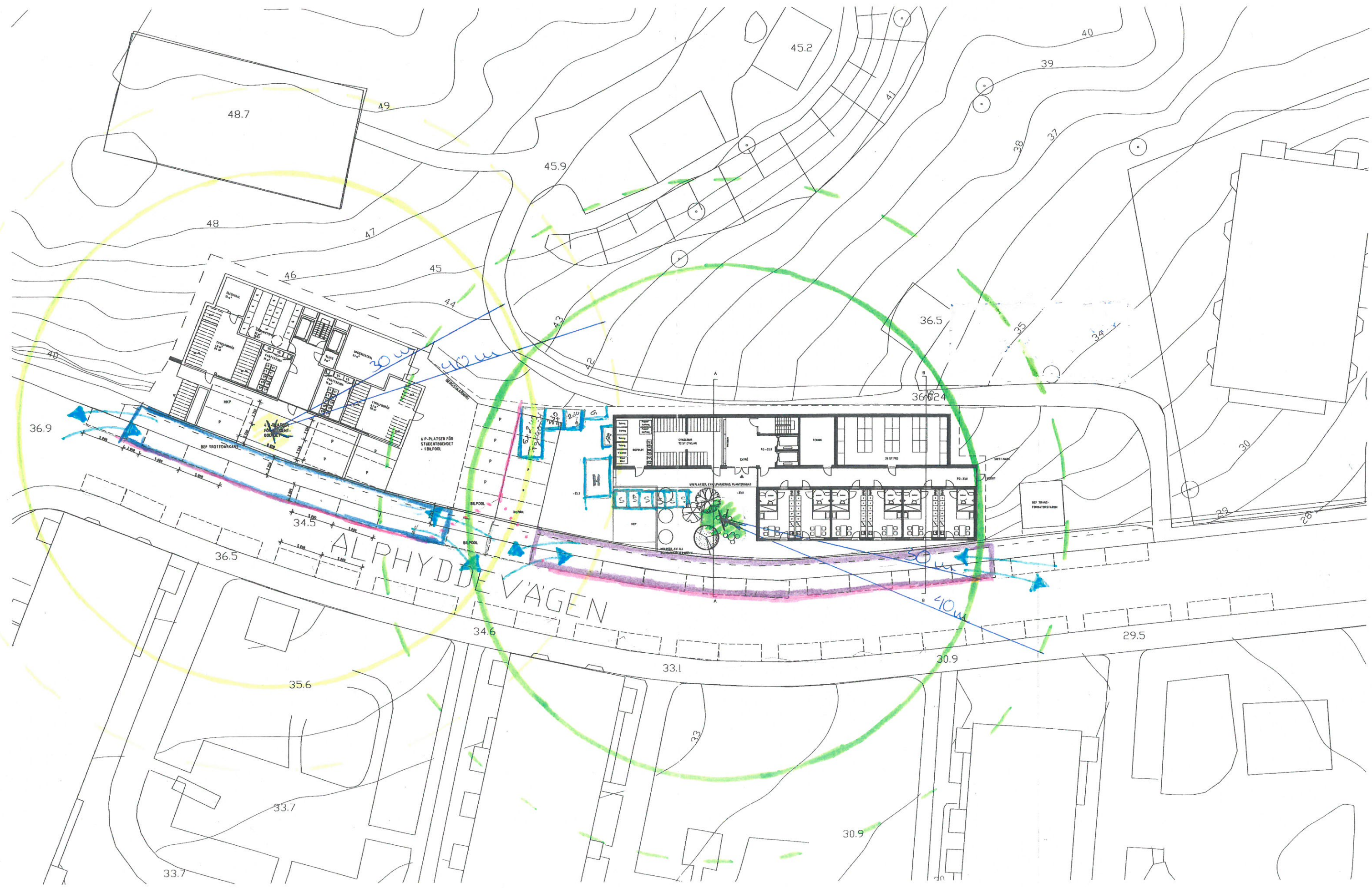
ALPHYDDAN, STUDENTBOSTÄDER. ENTREPLAN. 1:400 (A3). 141021.
