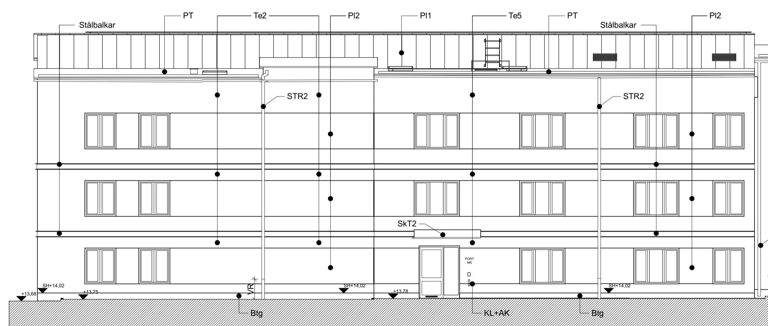
FASAD E - F, G - H MOT NORR
