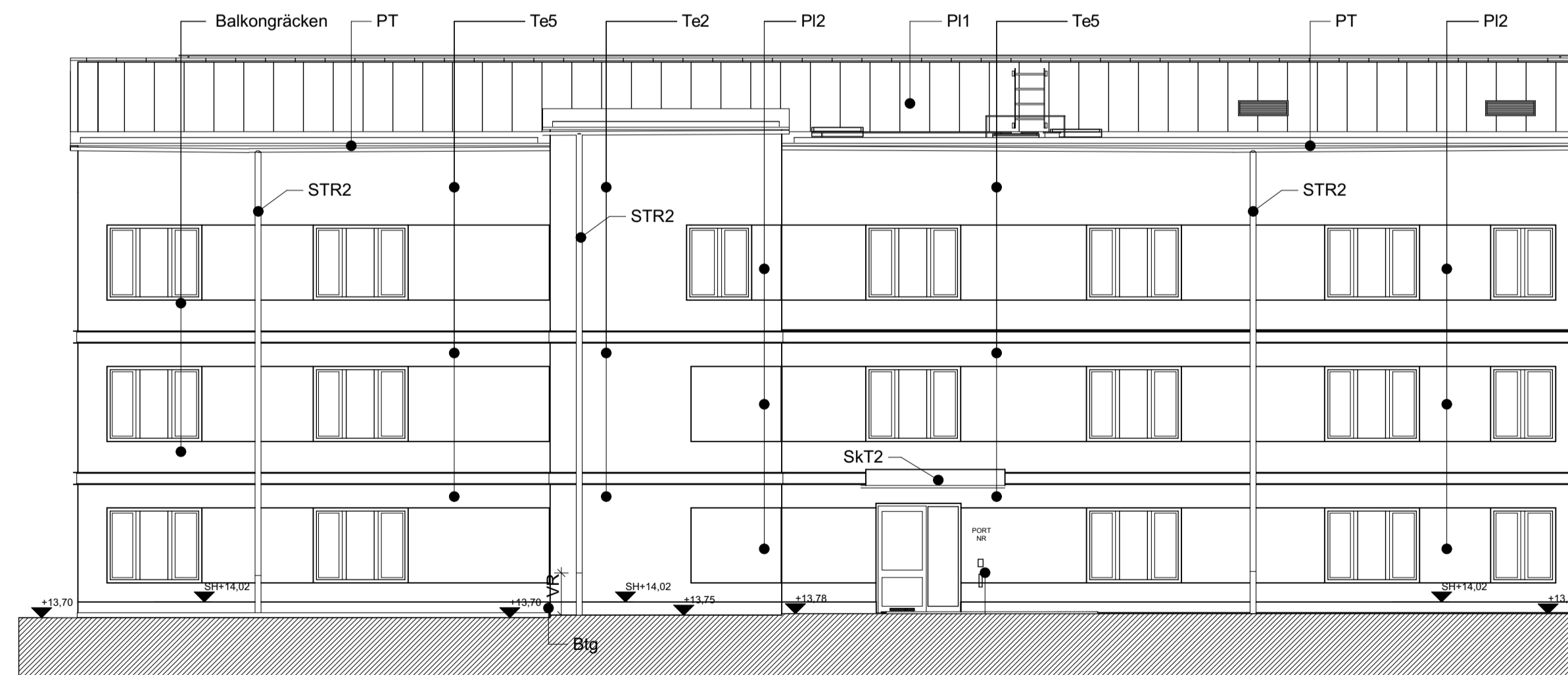
FASAD C - D, E - F, G - H MOT NORR
