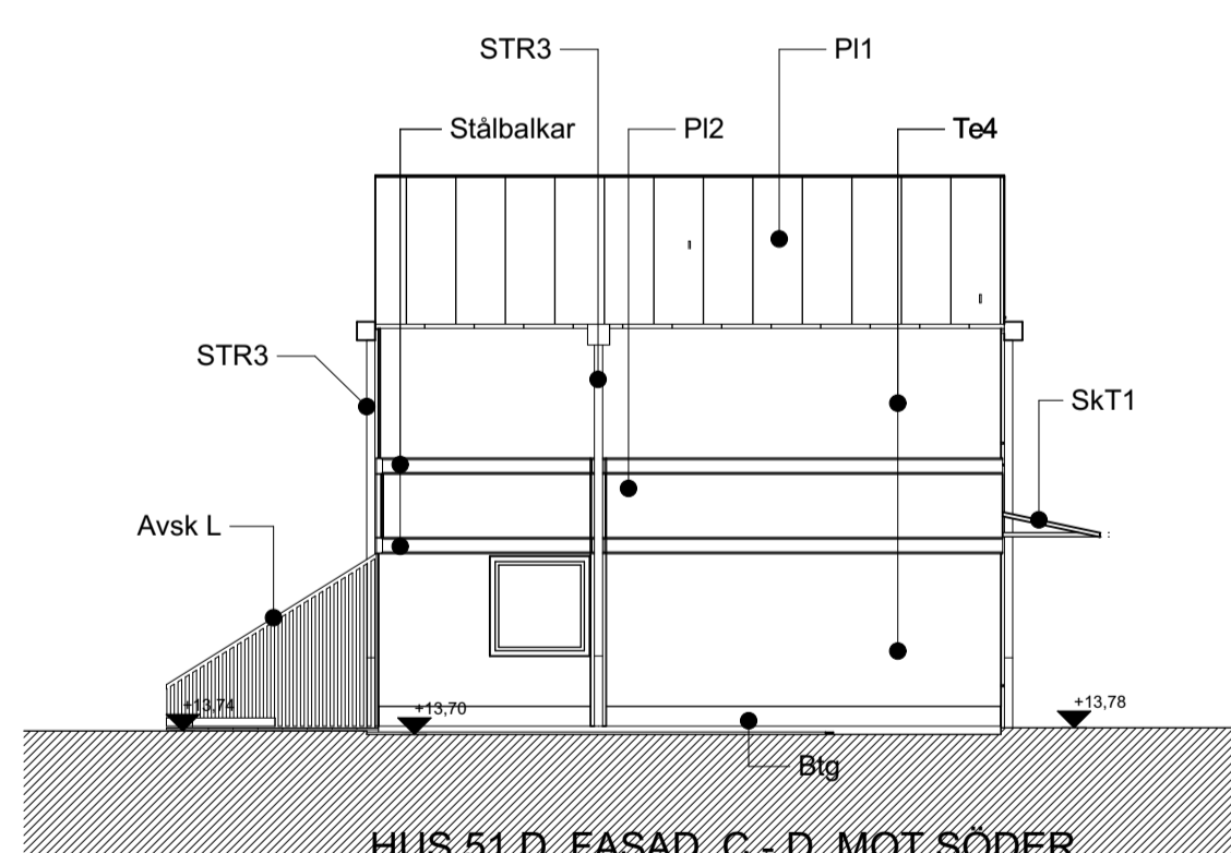
HUS 51 D FASAD C - D MOT SÖDER
