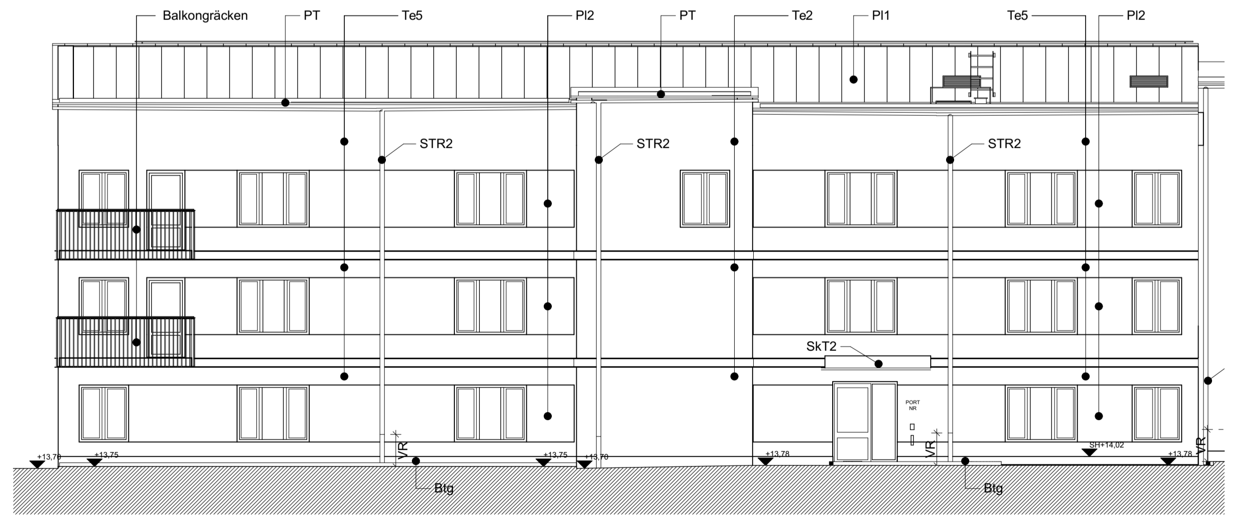
FASAD E - F, G - H MOT NORR
