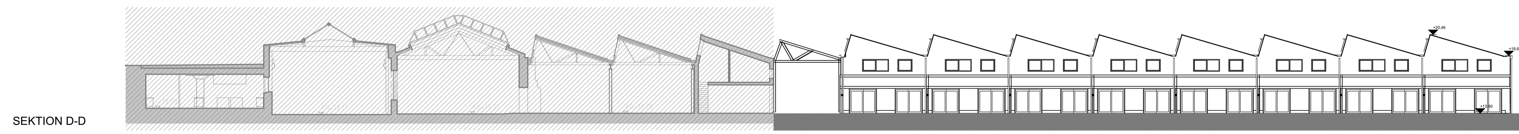
SEKTION D-D HUS 51 E HUS 51 D
