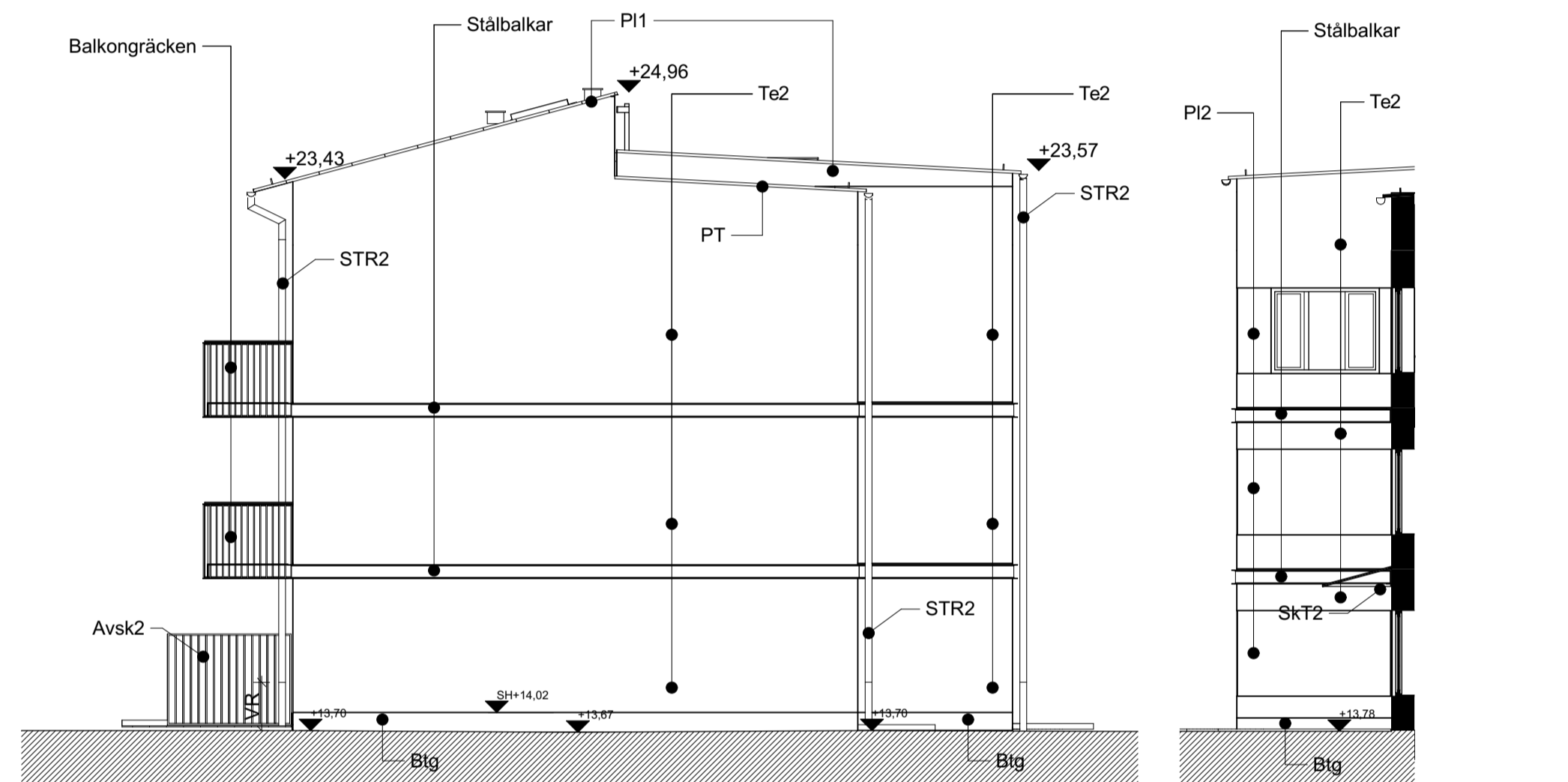
FASAD B - C, D - E MOT ÖSTER
