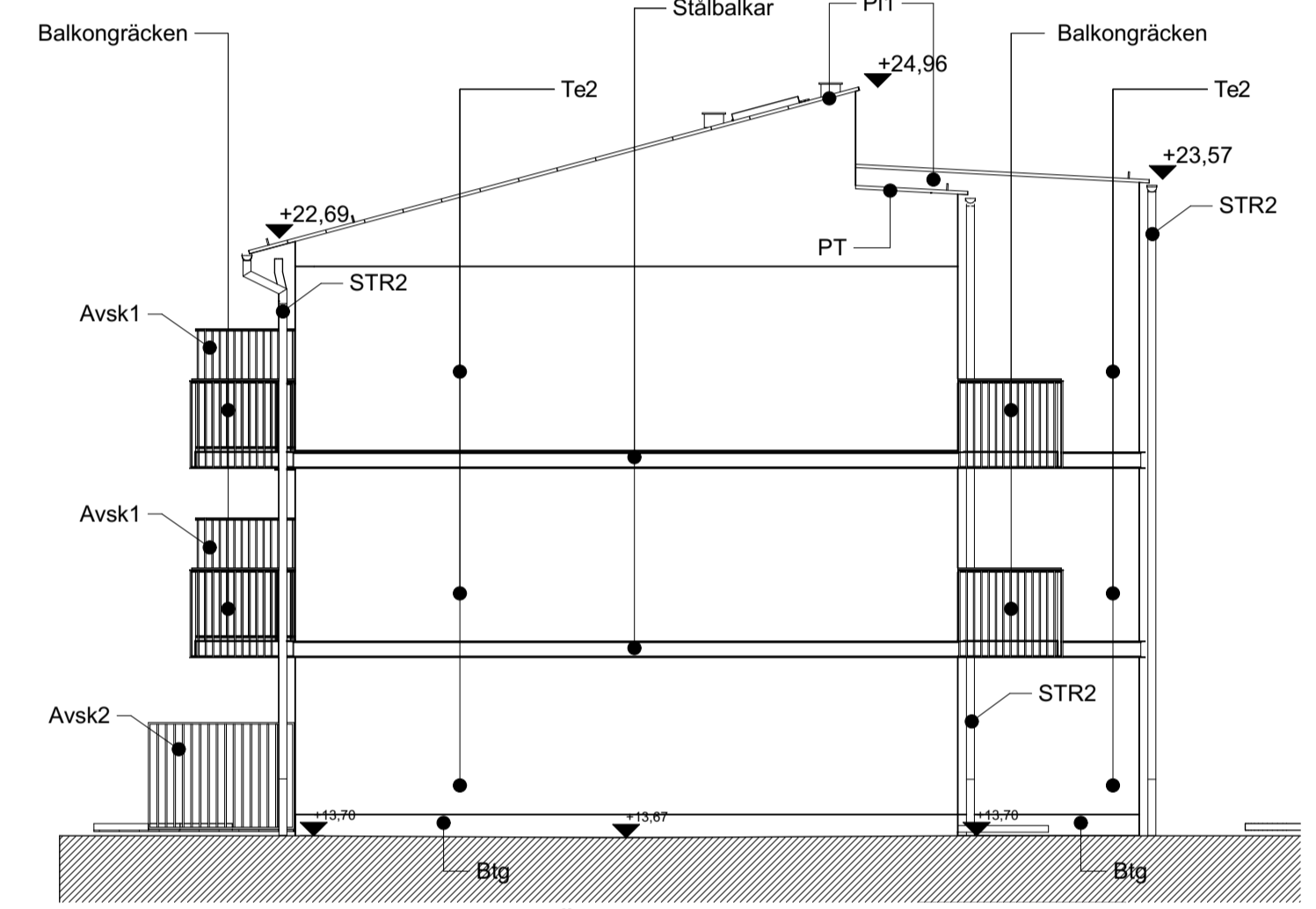
FASAD D - E, F - G MOT ÖSTER
