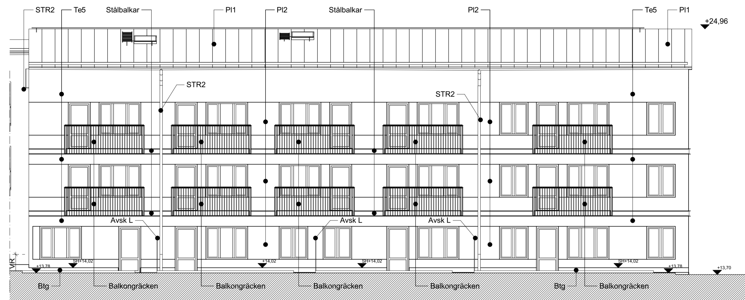
FASAD A - B MOT SÖDER
