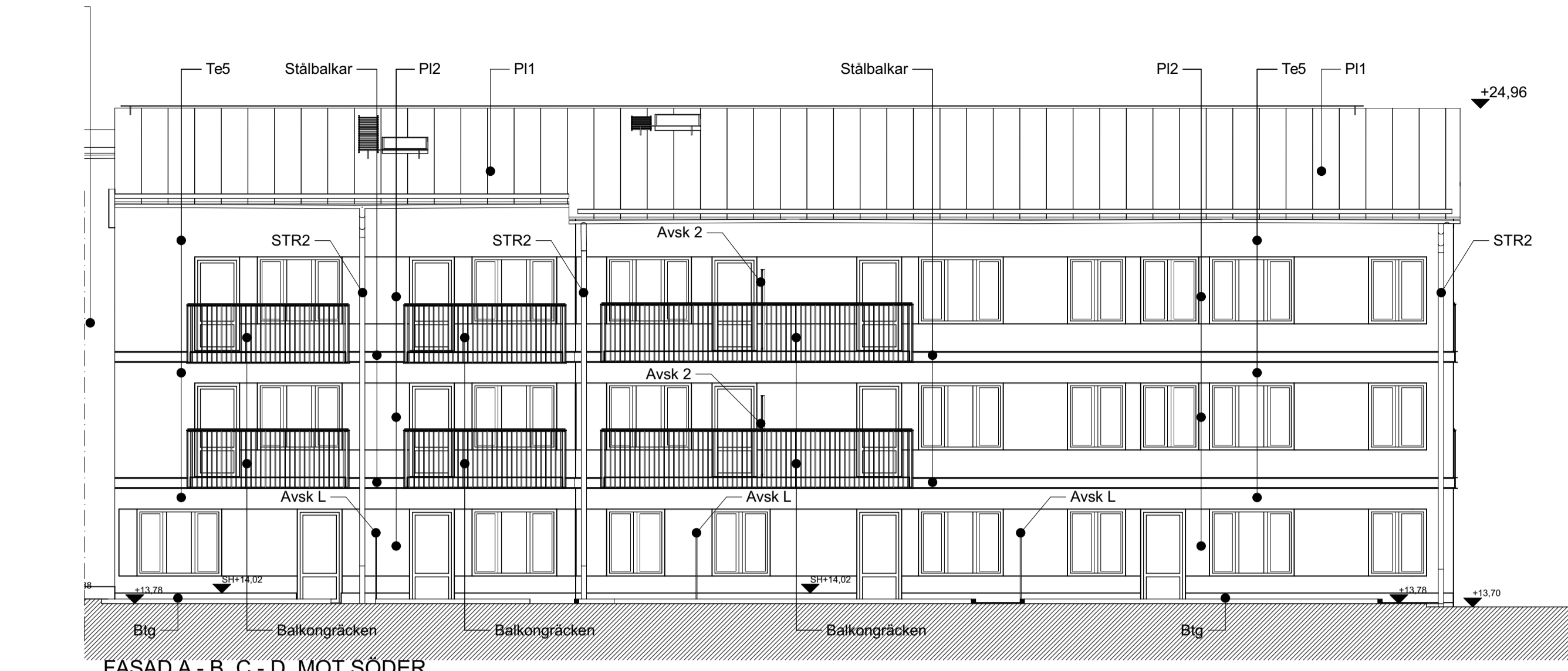
FASAD A - B, C - D MOT SÖDER
