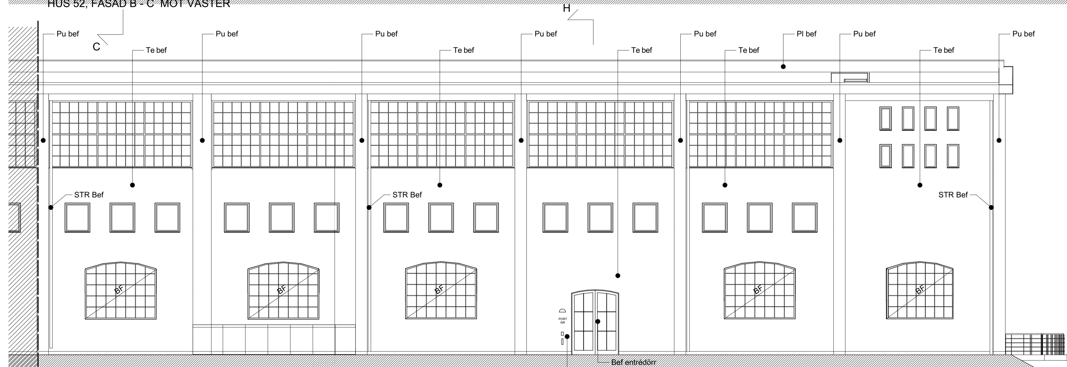
HUS 52, FASAD C - D MOT VÄSTER
