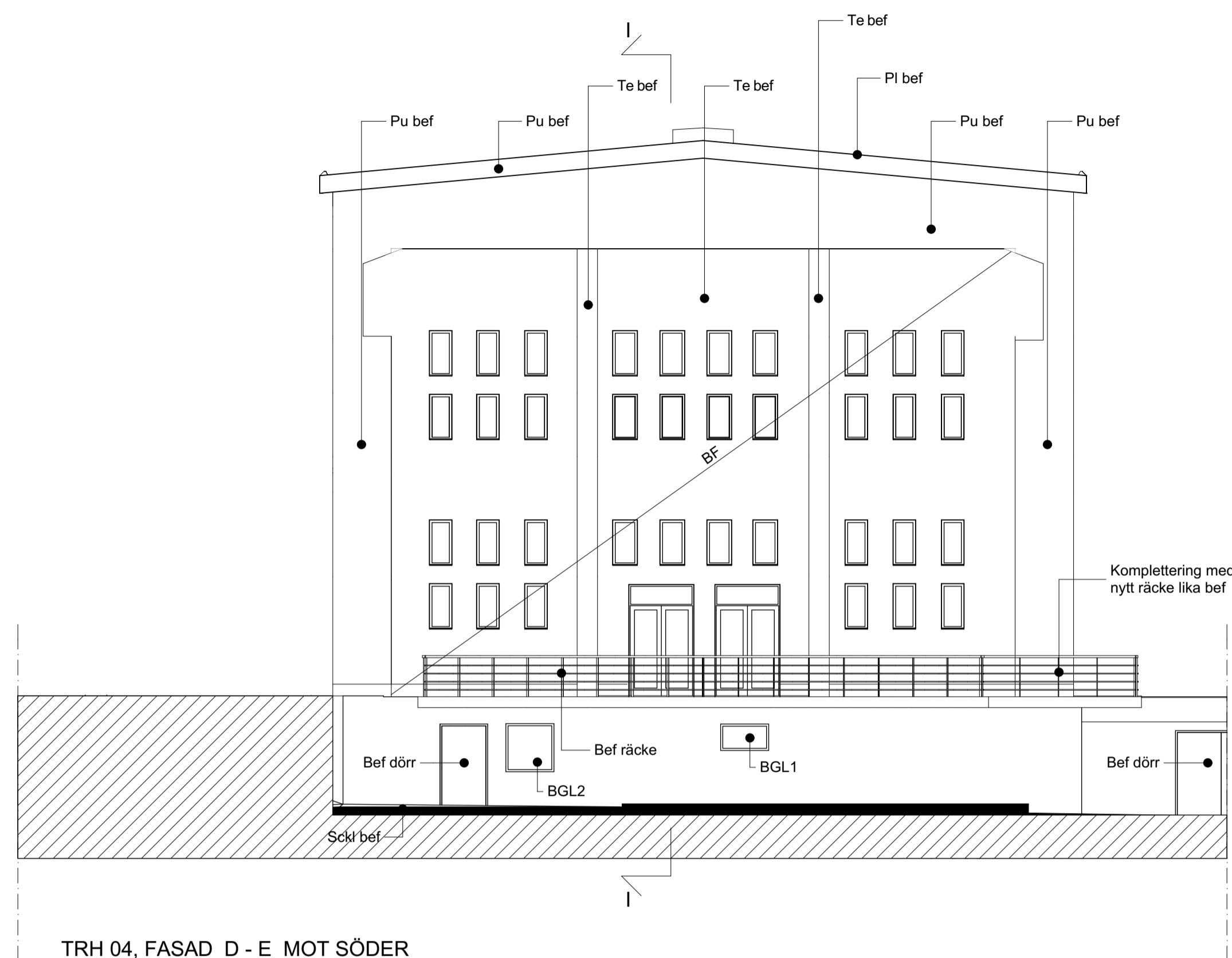
TRH 04, FASAD D - E MOT SÖDER
