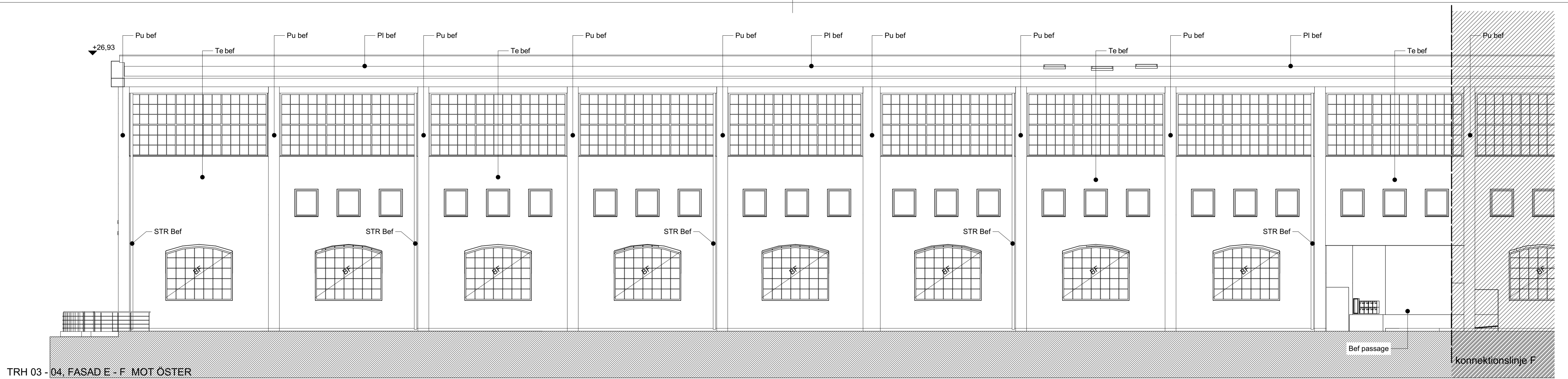
TRH 03 - 04, FASAD E - F MOT ÖSTER
