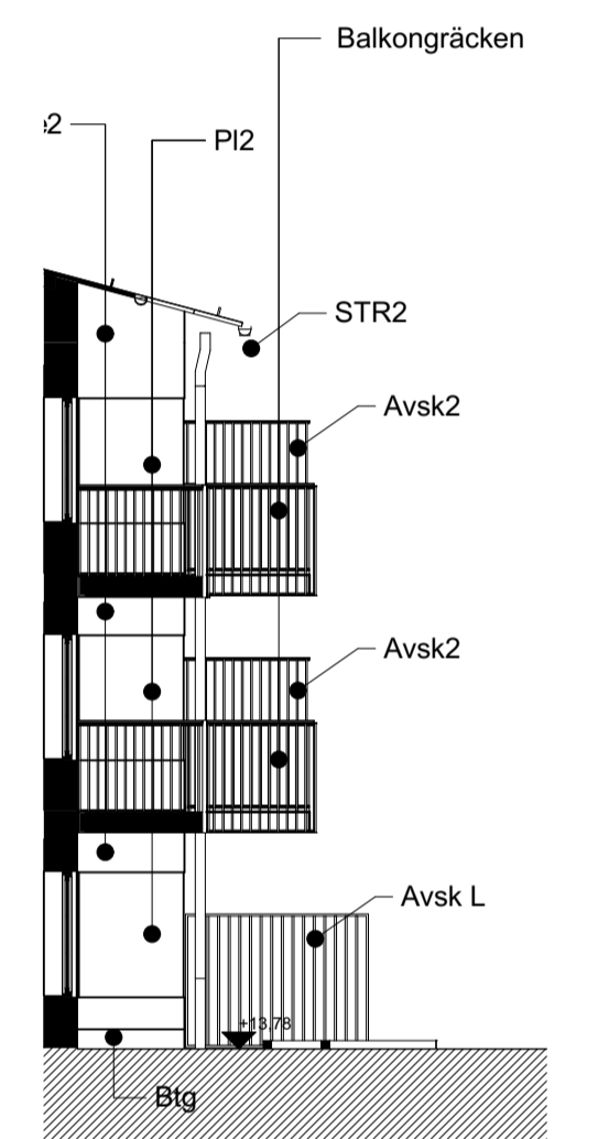
FASAD B - C MOT VÄSTER
