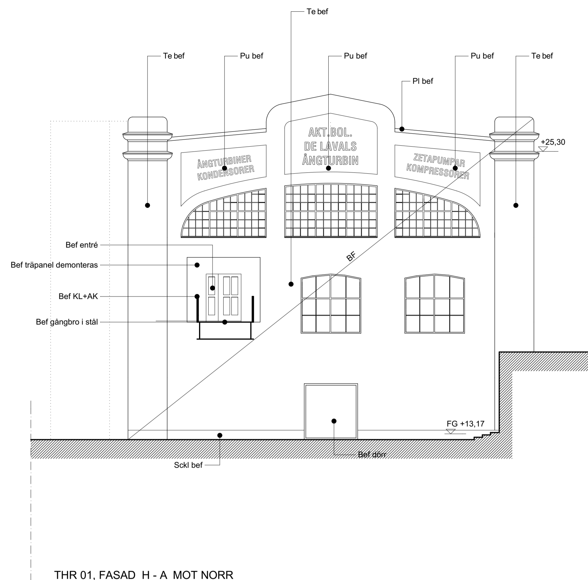
THR 01, FASAD H - A MOT NORR
