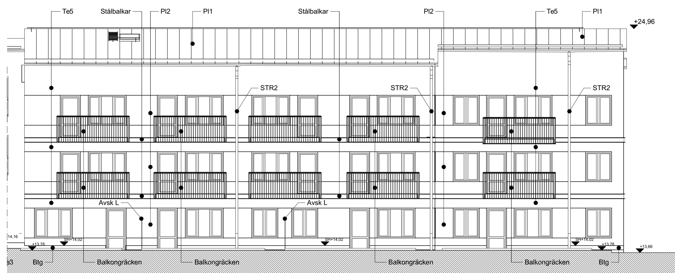
FASAD A - B, C - D MOT SÖDER
