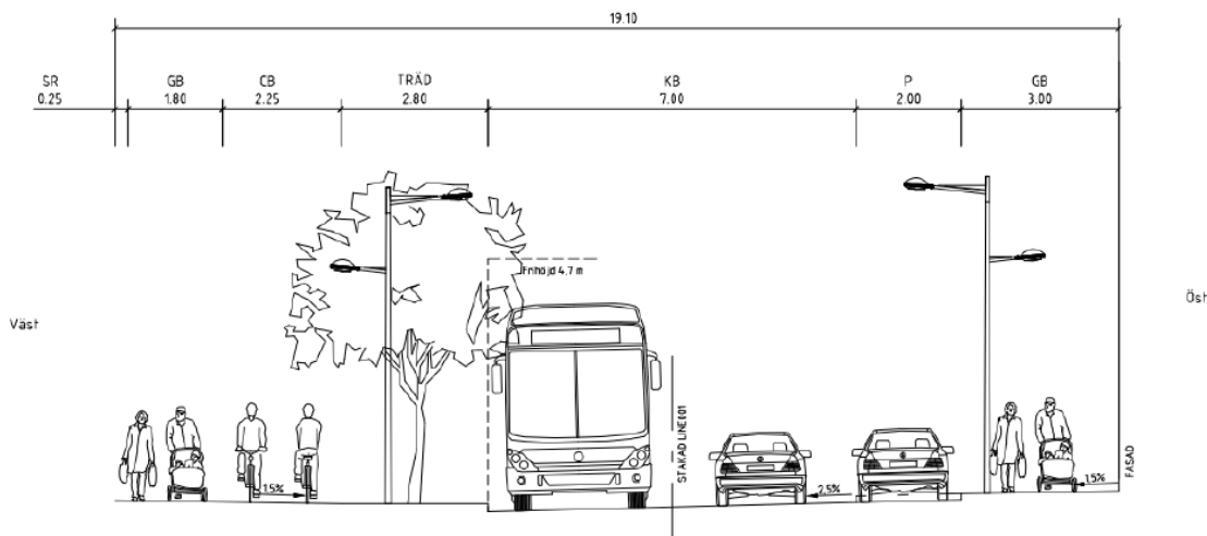
Figur 22. Principsektion (ej skalenlig) för Oxelvägen (Bild: Sweco).
