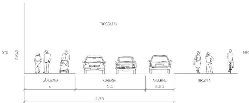
Figur 23. Principsektion för torggatan (ej skalenlig). Bild: Sweco
