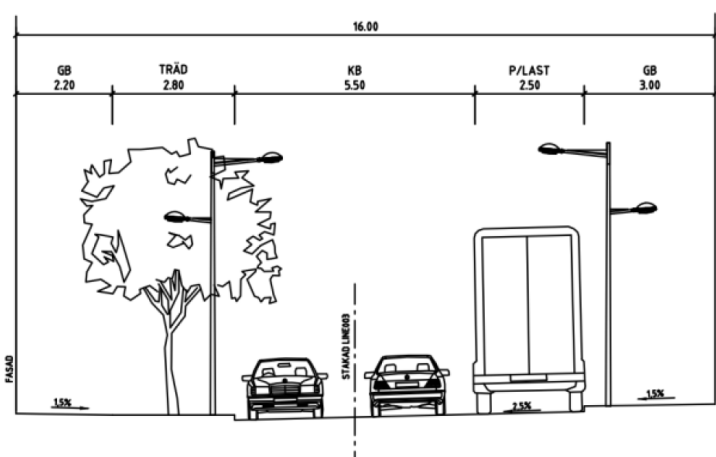
Figur 24. Principsektion (ej skalenlig) för lokalgatan (Bild: Sweco).
