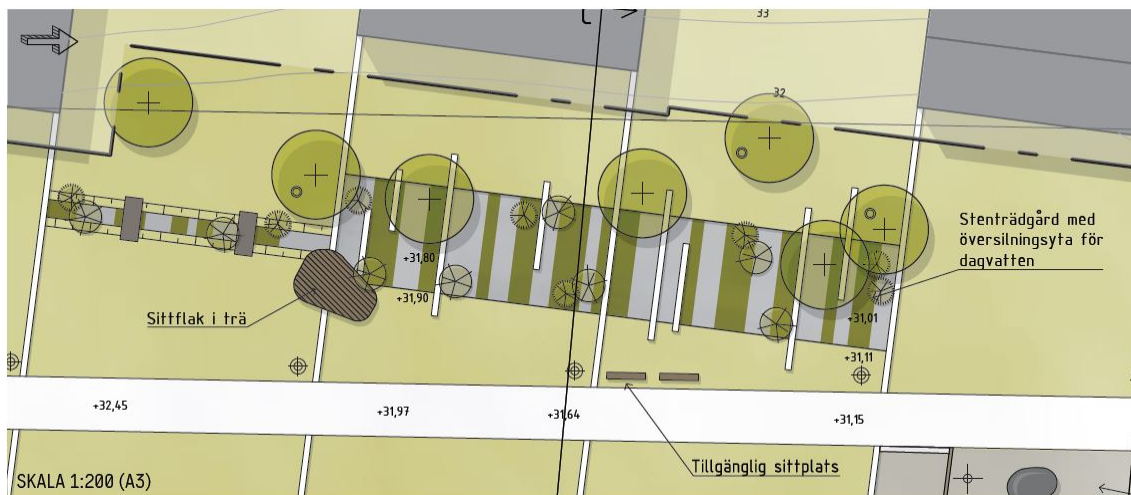
Figur 27. Illustrationen (ej skalenlig) visar föreslagen dagvattenanläggning i parkstråket (Bild: Sweco).
