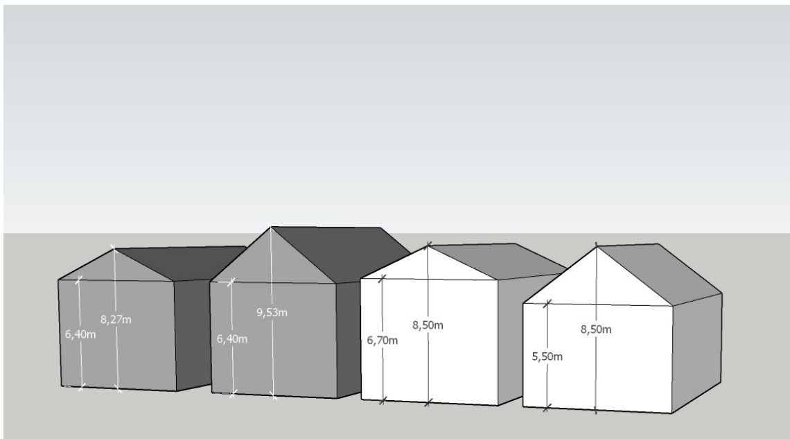
Figur 3. Exempel på husvolymmer med olika bestämmelser för höjd på byggnaderna om huset är 8 meter brett. De två gråa husen till vänster illustrerar planbestämmelsen från stadsplanen som reglerar byggnadshöjd 6,4 med takvinklarna 25 respektive 38 grader. De två vita husen till höger illustrerar planbestämmelsen från planförslaget som reglerar nockhöjd 8,5 och takvinkel mellan 25–38 grader.
