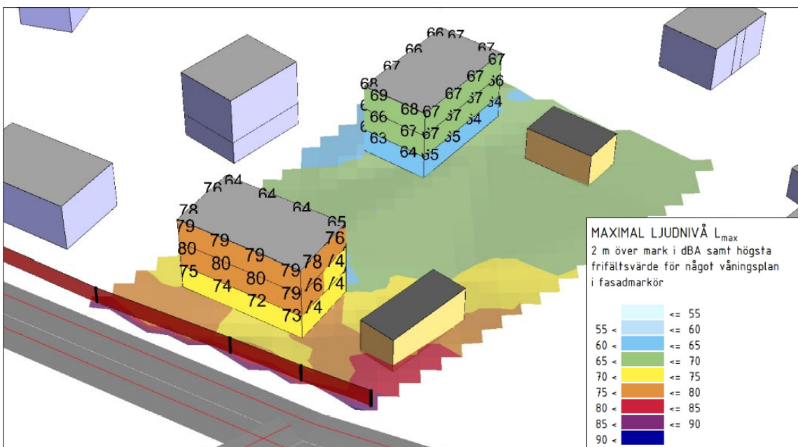
Maximal ljudnivå, möjlig placering av bebyggelse med fasad mot Mensättravägen. Illustration: Norconsult, 2019.
