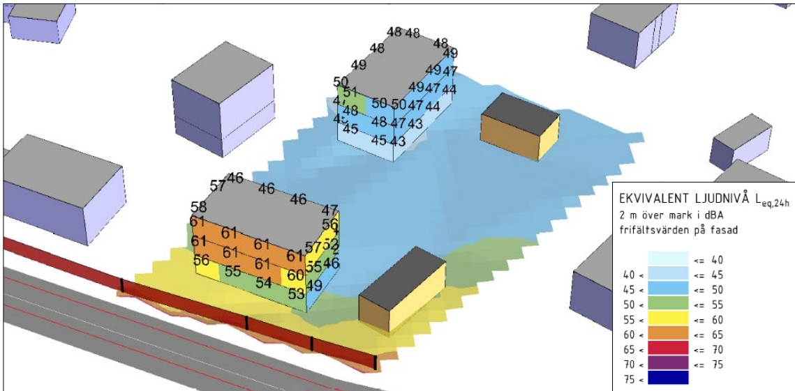
Ekvivalent ljudnivå, möjlig placering av bebyggelse med fasad mot Mensättravägen. Illustration: Norconsult, 2019.
