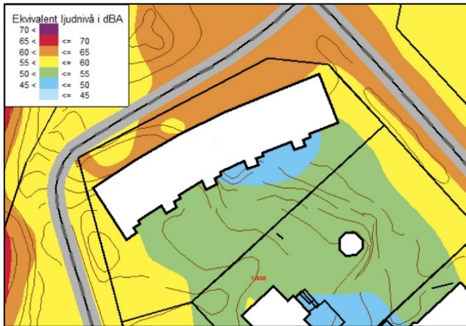
Exempel på möjlig utformning av radbus på fastigheten Lännersta 1:837. Ytterligare bulleravskärmande åtgärder kan behövas. Källa: Structor Akustik.
