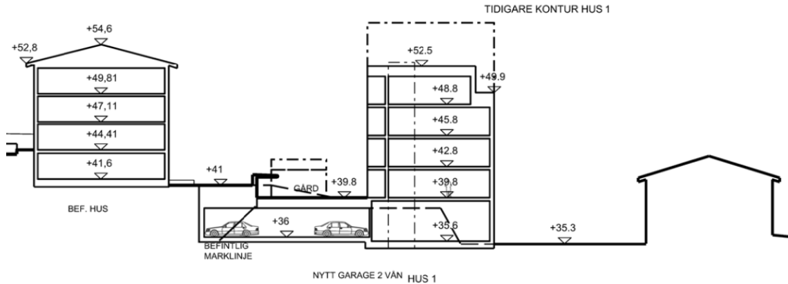
Föreslagen parkering i garage. Illustration: Krook & Tjäder arkitekter.
