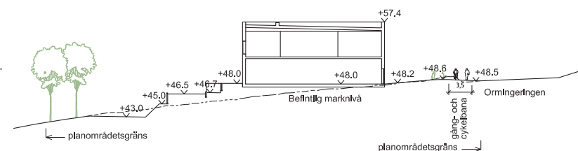
Sektion B-B
