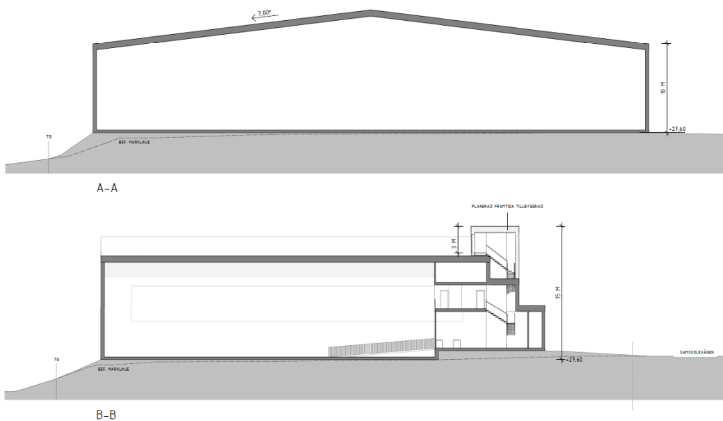
Figur 4. Sektioner genom ny tennishall
