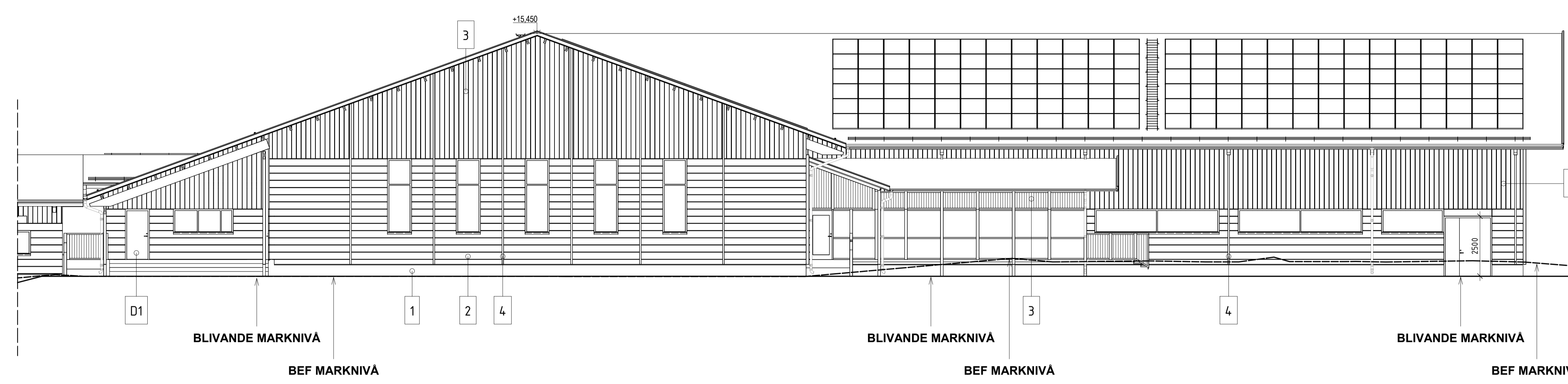
1: 100 Ridhus, Fasad mot väster
