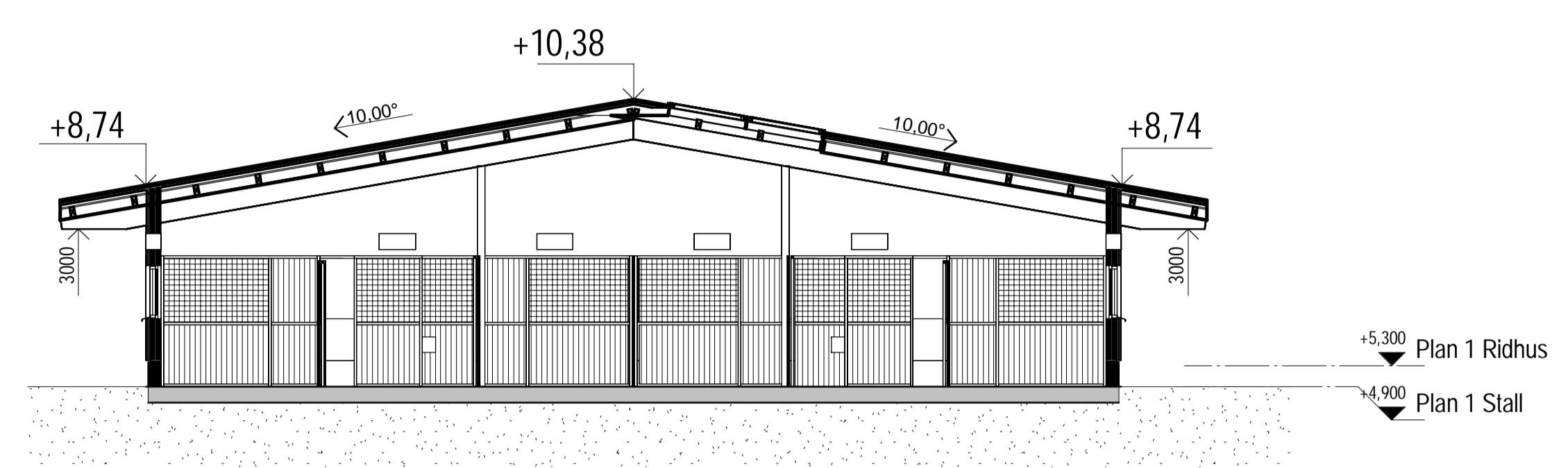
D. 1:100 Sektion D Stall
