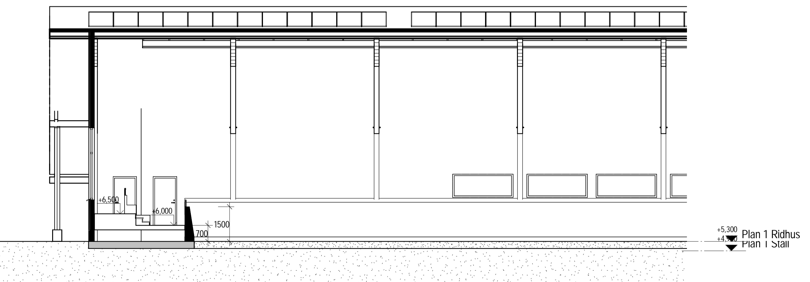
G. 1:100 Sektion G Ridhus
