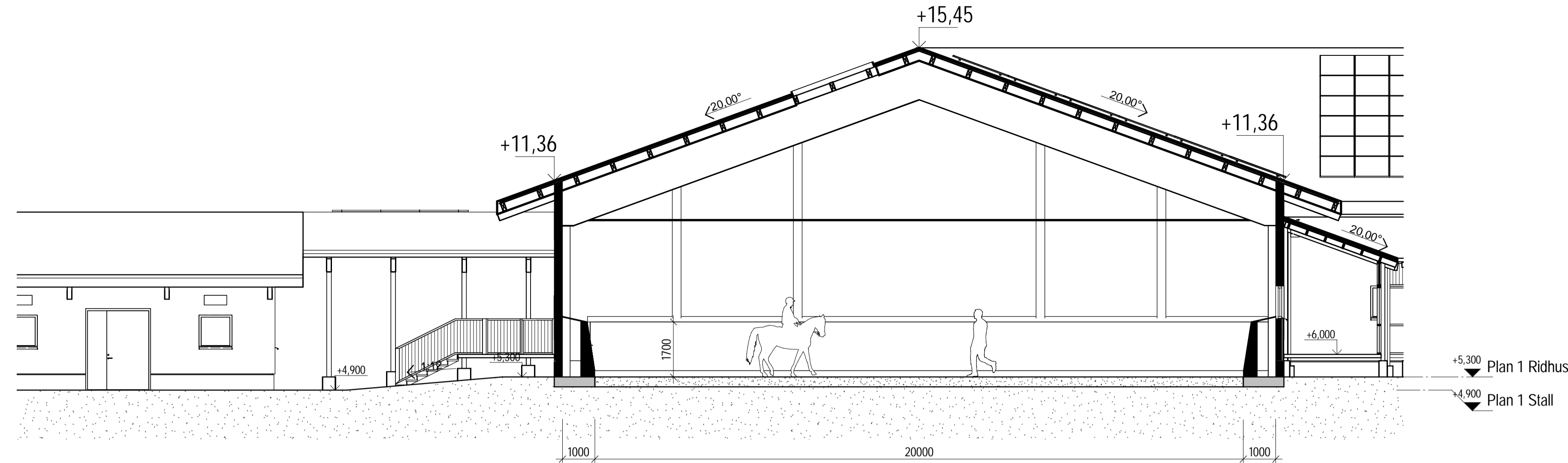
A. 1:100 Sektion A Ridhus
