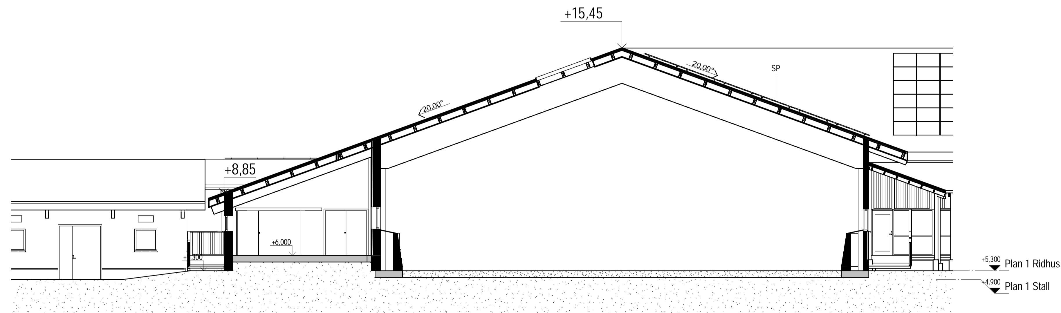
F. 1:100 Sektion F Ridhus
