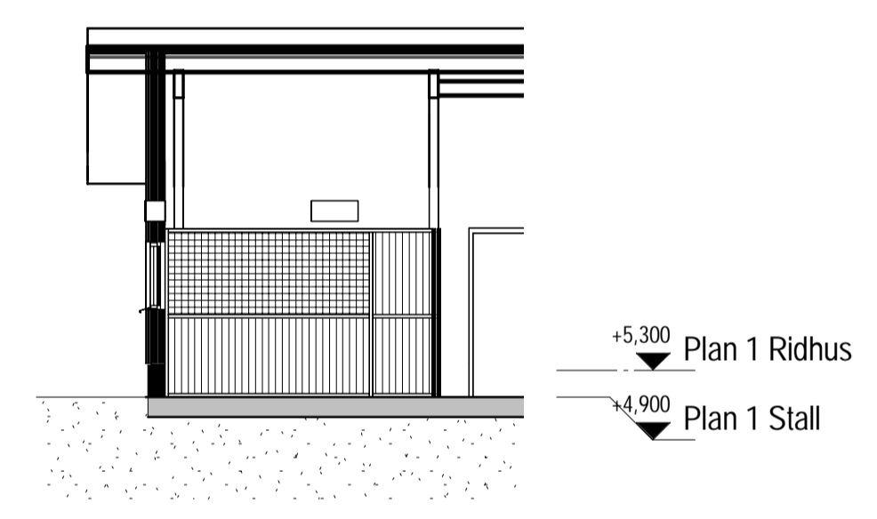
E. 1:100 Sektion E
