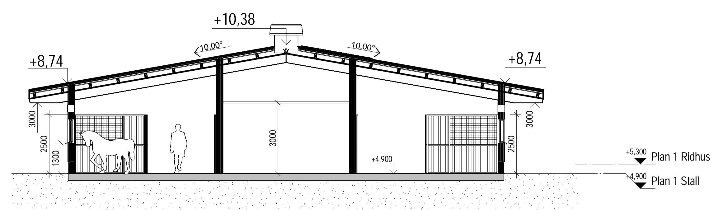
B. 1:100 Sektion B Stall
