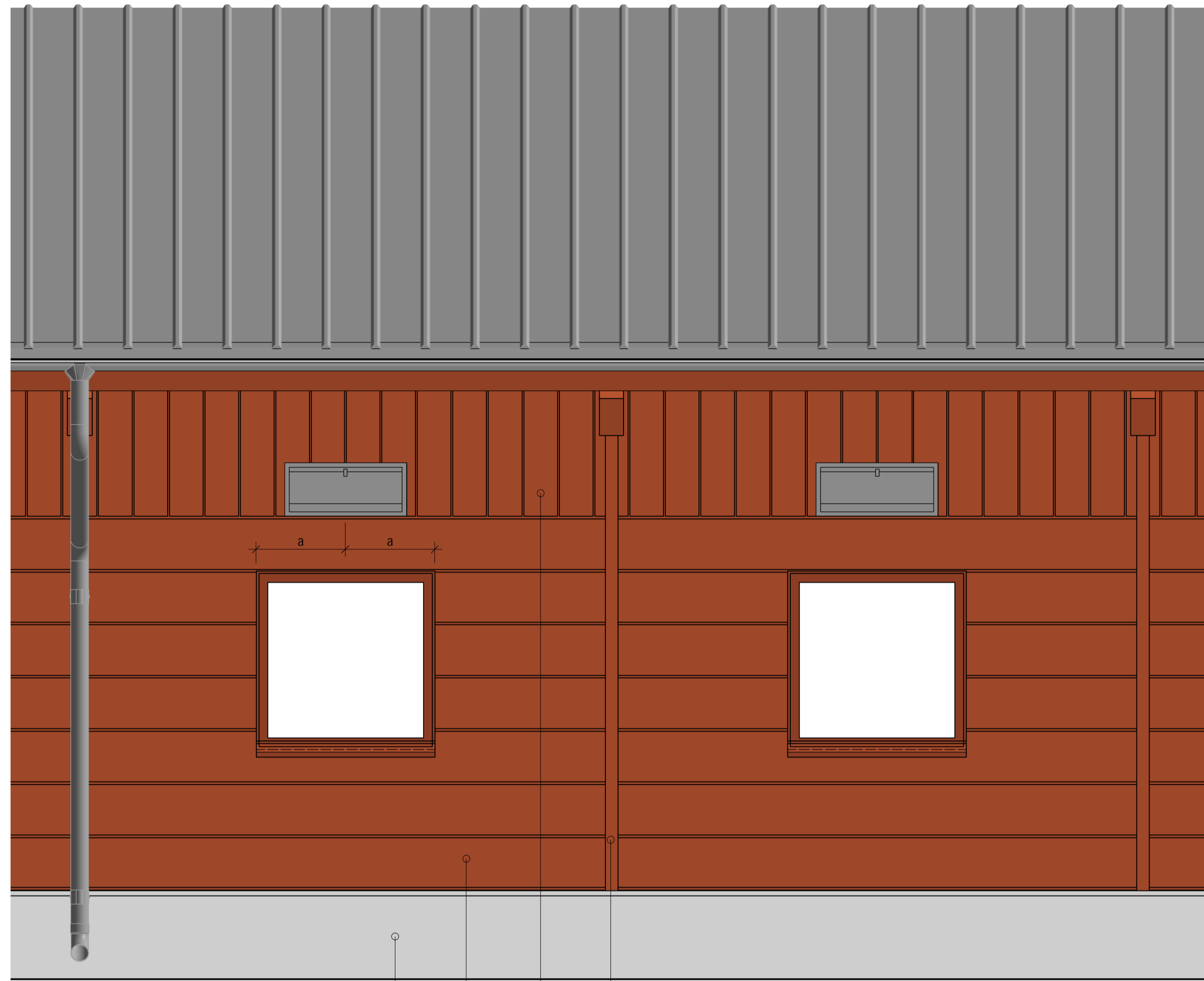
1 : 20 Fasadutsnitt, typlösning
