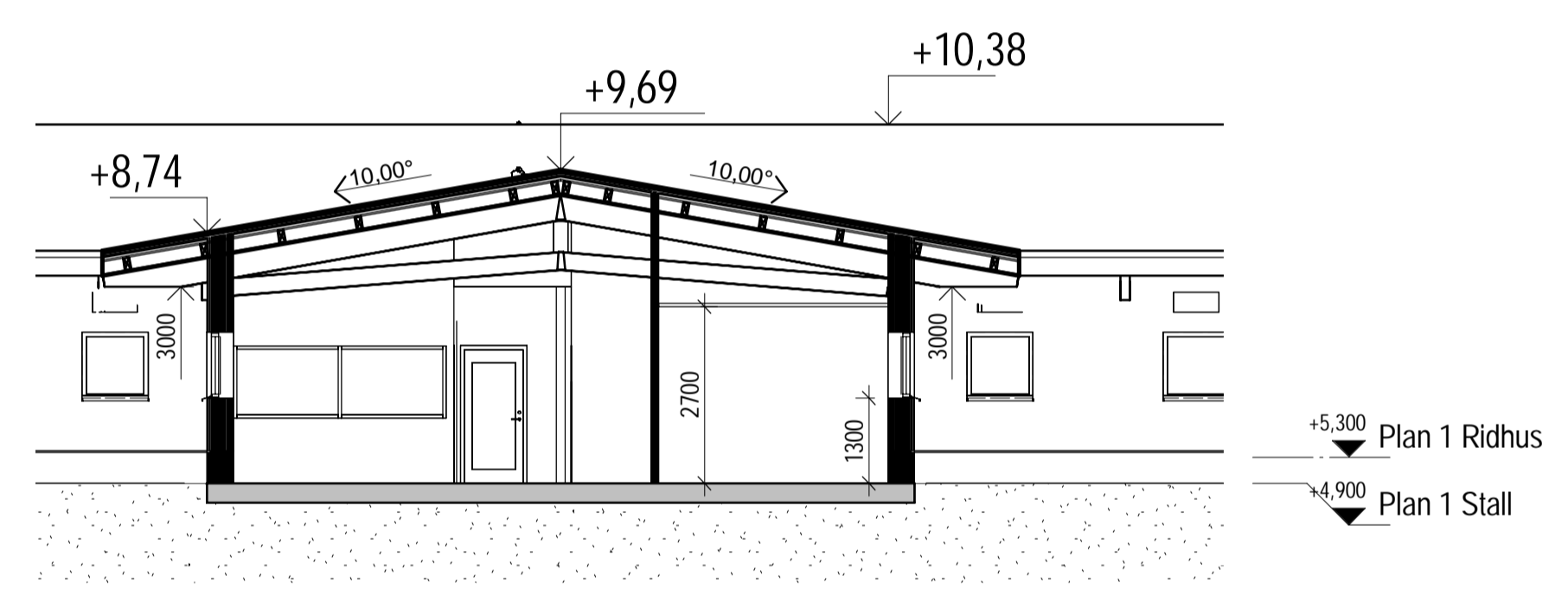
C. 1:100 Sektion C
