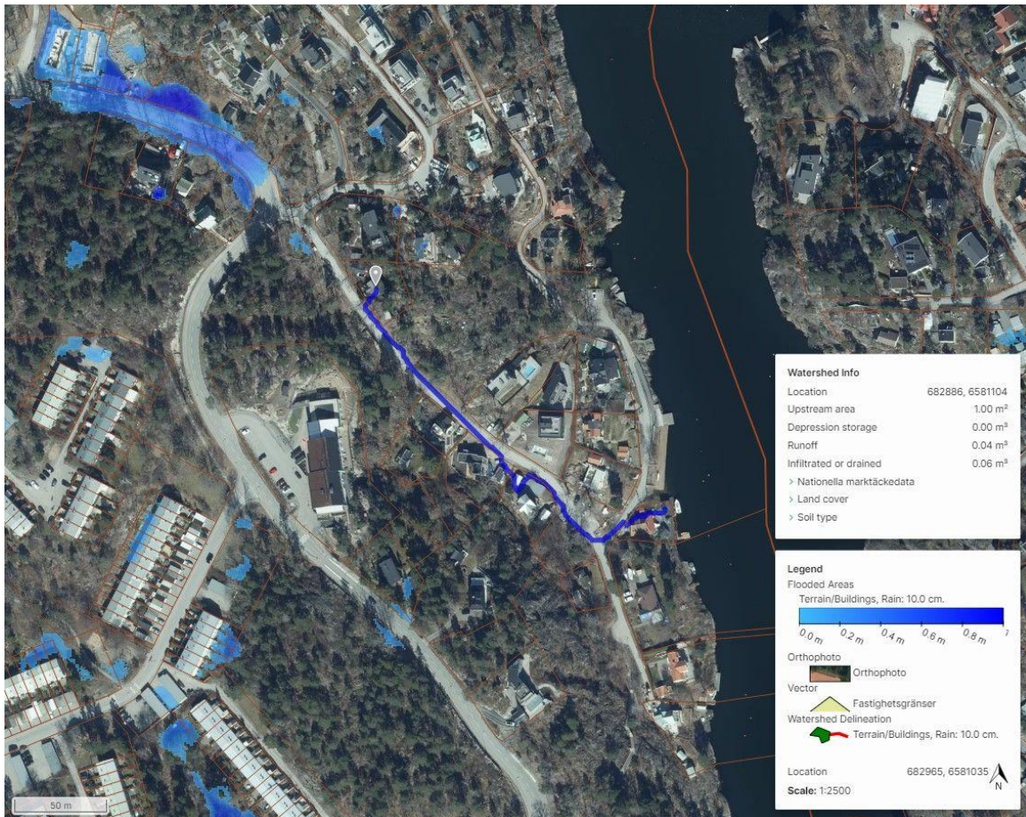
Figur 11. Skyfallsanalys i Scalgo live vid ett 100-mm regn.
