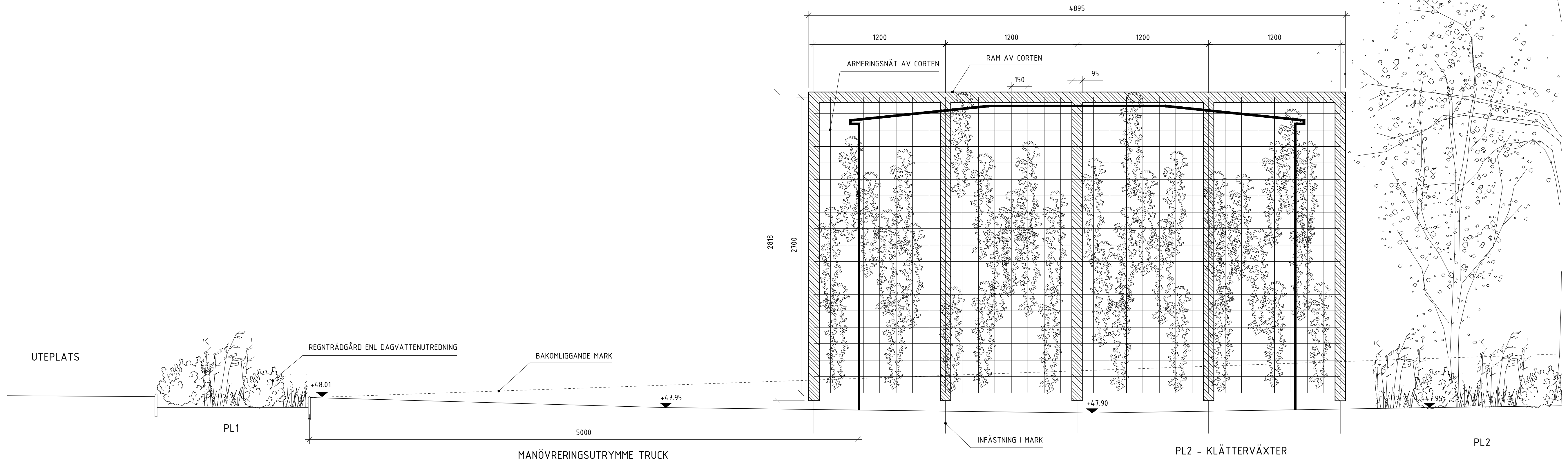
DETALJ - S0 - SPALJÉ ELNÄTSTATION SEKTION A-A' SKALA 1:20 (A1)
