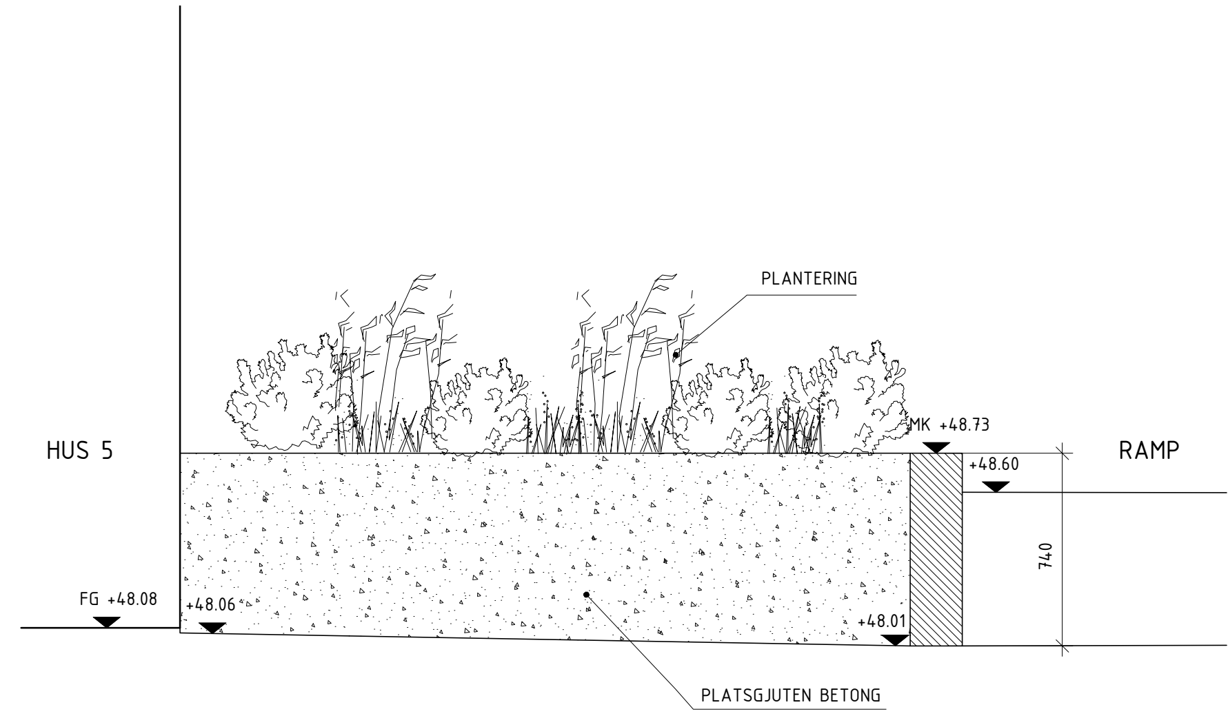
DETALJ - M1 SEKTION C-C' SKALA 1:20 (A1)
