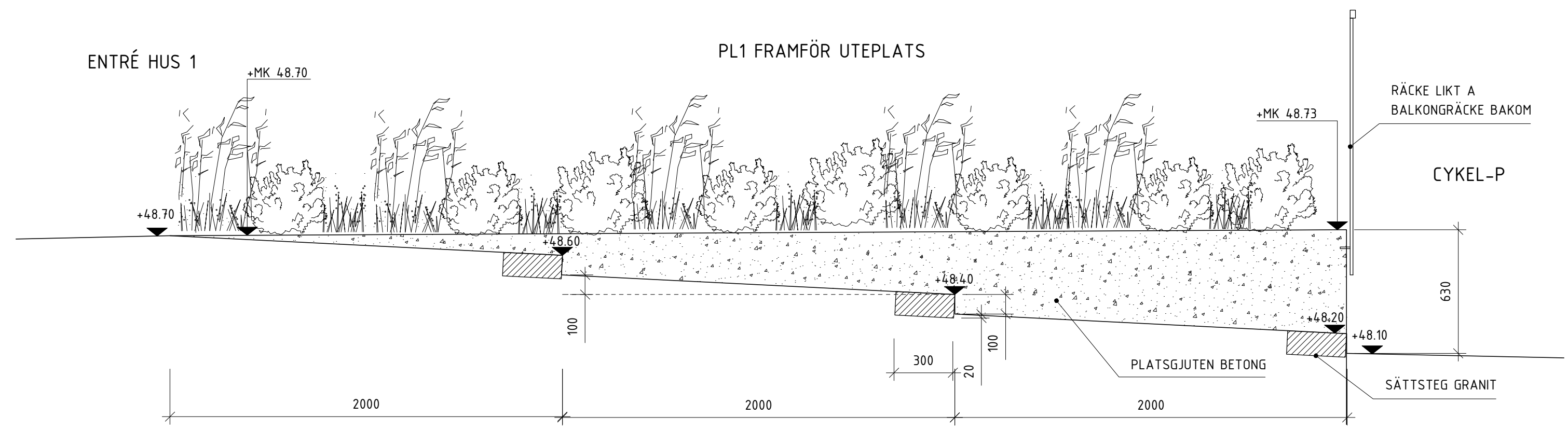
DETALJ - M1, TRP1 SEKTION B-B' SKALA 1:20 (A1)
