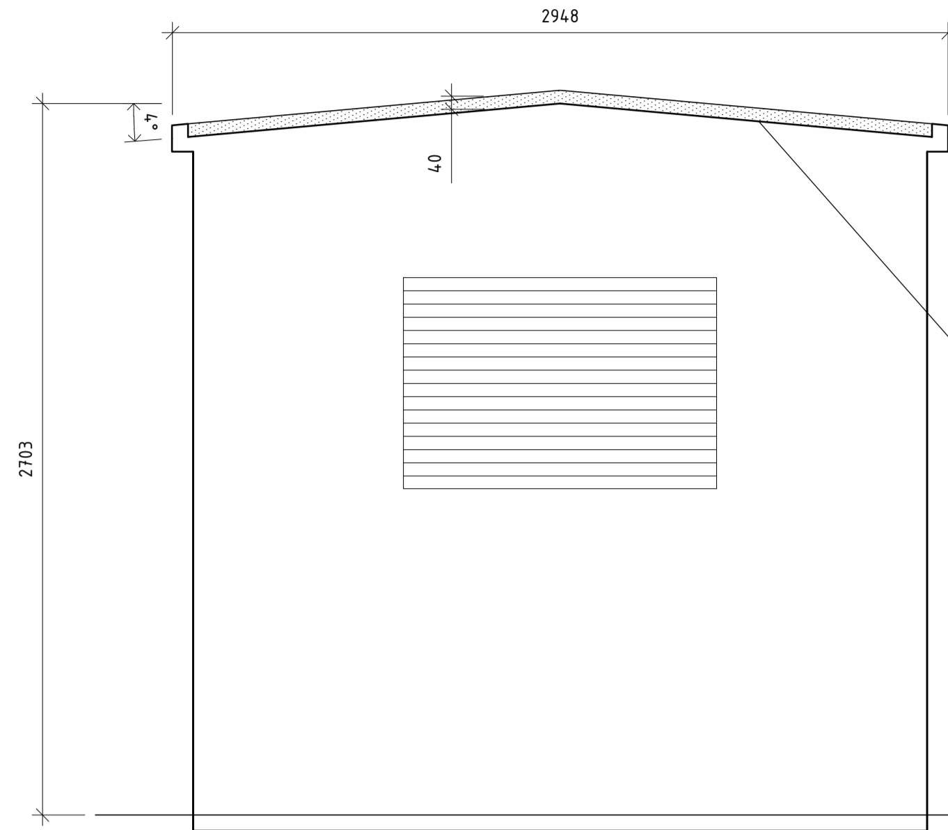
VY ELNÄTSTATION B1 MED SEDUMTAK KORTSIDA, BAKSIDA SKALA 1:20 (A1)
