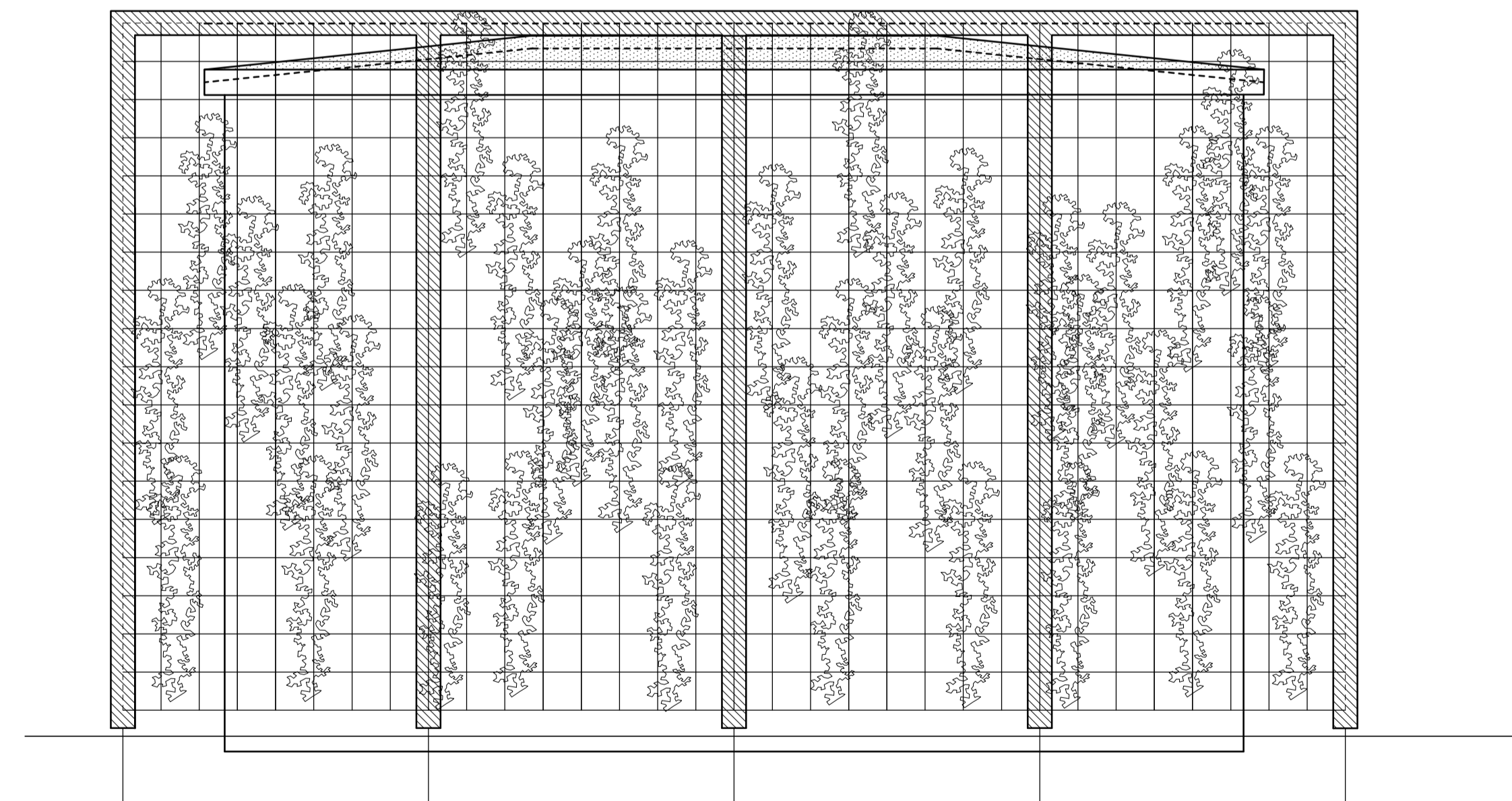
VY ELNÄTSTATION B1 MED SEDUMTAK OCH SPALJÉ LÅNGSIDA SKALA 1:20 (A1)
