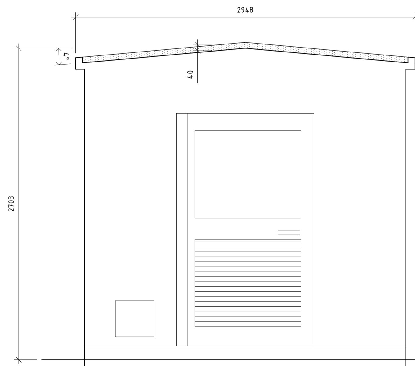
VY ELNÄTSTATION B1 MED SEDUMTAK KORTSIDA MED DÖRR SKALA 1:20 (A1)
