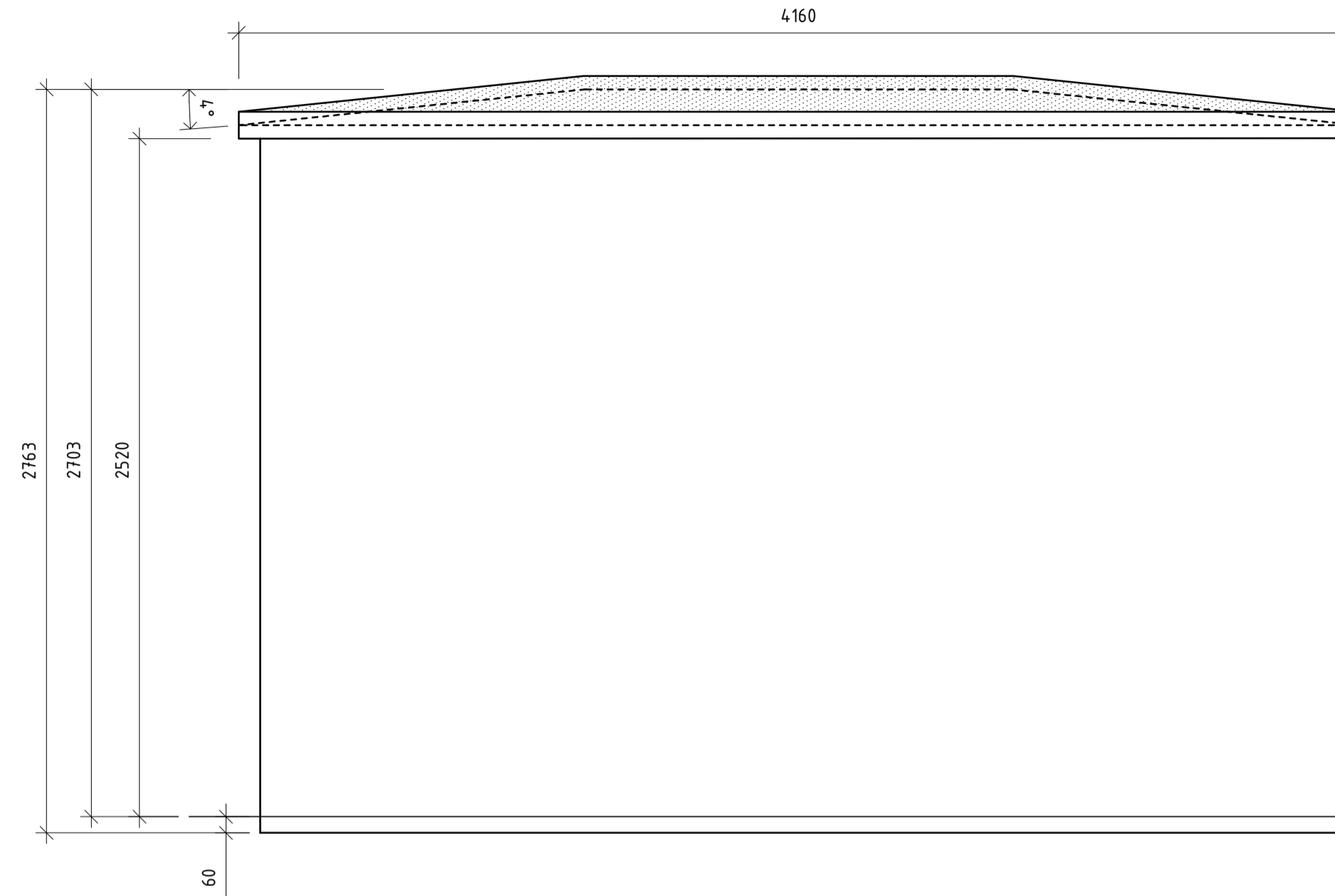
VY ELNÄTSTATION B1 MED SEDUMTAK LÅNGSIDA SKALA 1:20 (A1)
